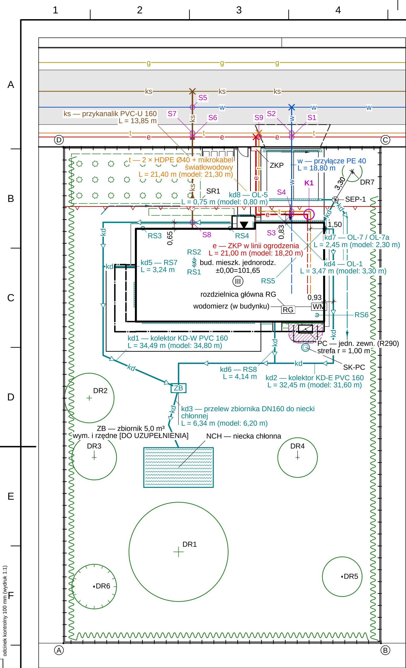
RYSUNEK KOORDYNACYJNY UZBROJENIA TERENU 1:200
