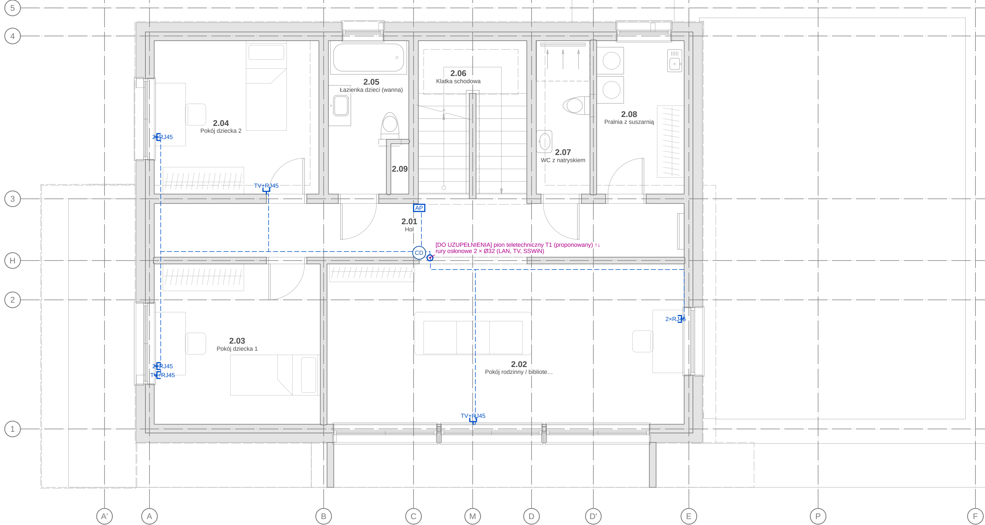
TELETECHNIKA — RZUT I PIĘTRA 1:50
