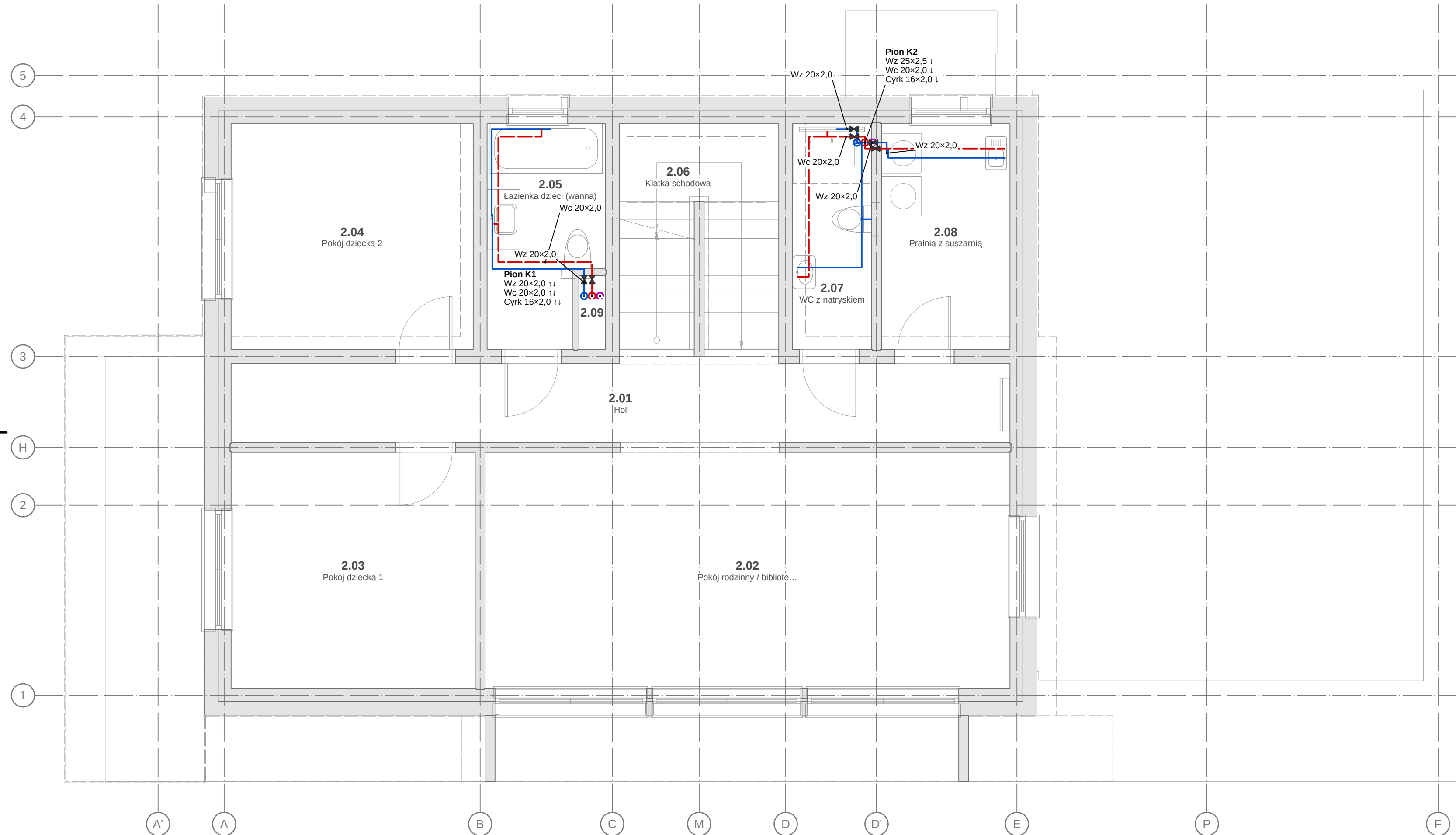
INSTALACJA WODOCIĄGOWA — RZUT I PIĘTRA 1:50
