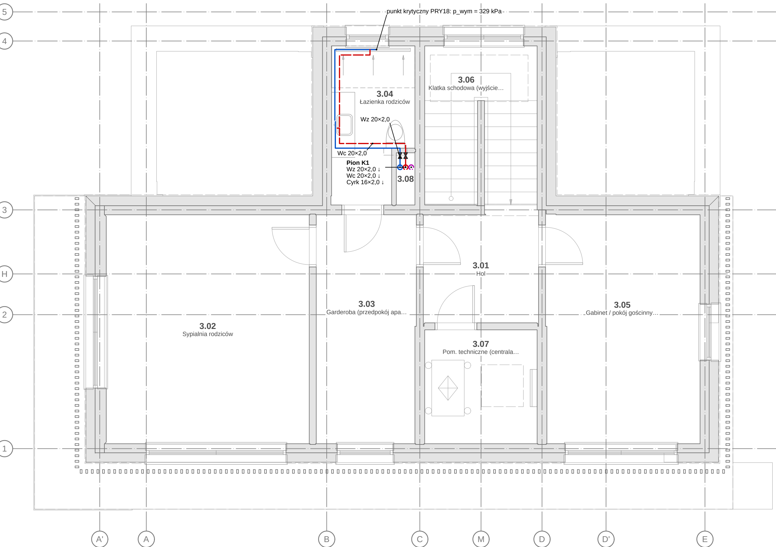
INSTALACJA WODOCIĄGOWA — RZUT II PIĘTRA 1:50
