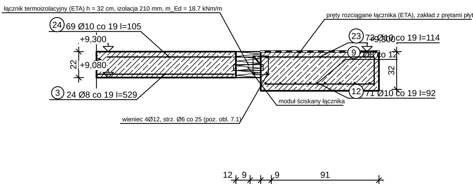
WEZEŁ WSPORNIKA PL-3 — ŁĄCZNIK TERMOIZOLACYJNY 1:20
