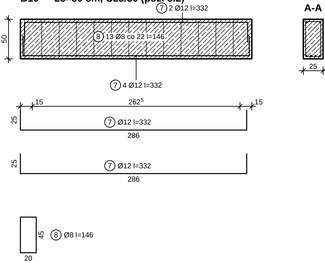
B10 — 25×50 cm, C25/30 (poz. 5.2)
