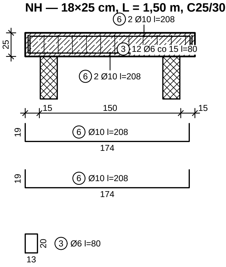
TYPY NADPROŻY — OTWORY I POZYCJE OBLICZEŃ
