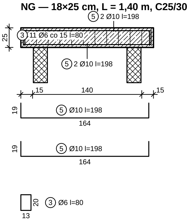
ZESTAWIENIE STALI
