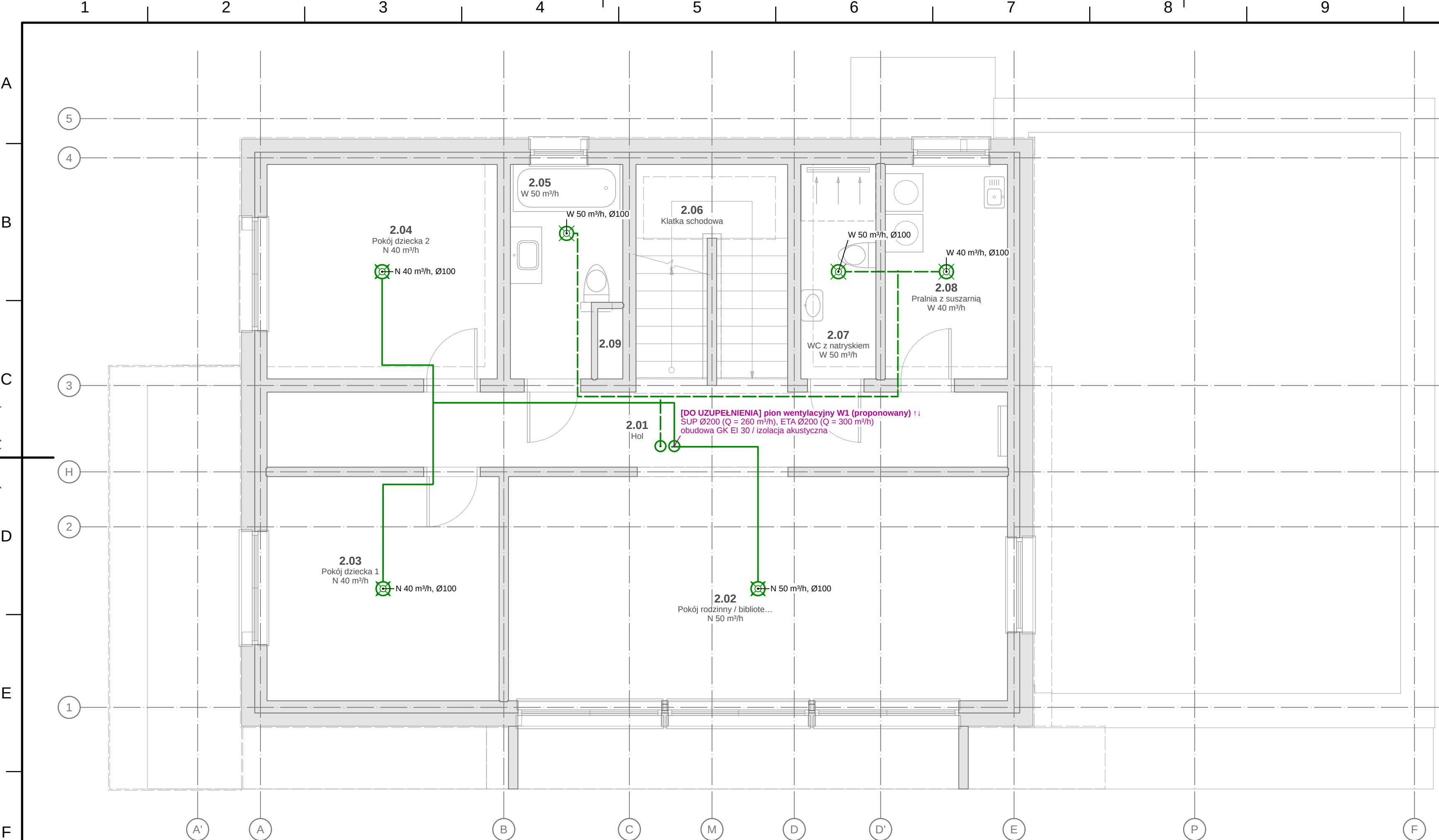
WENTYLACJA MECHANICZNA — RZUT I PIĘTRA 1:50
