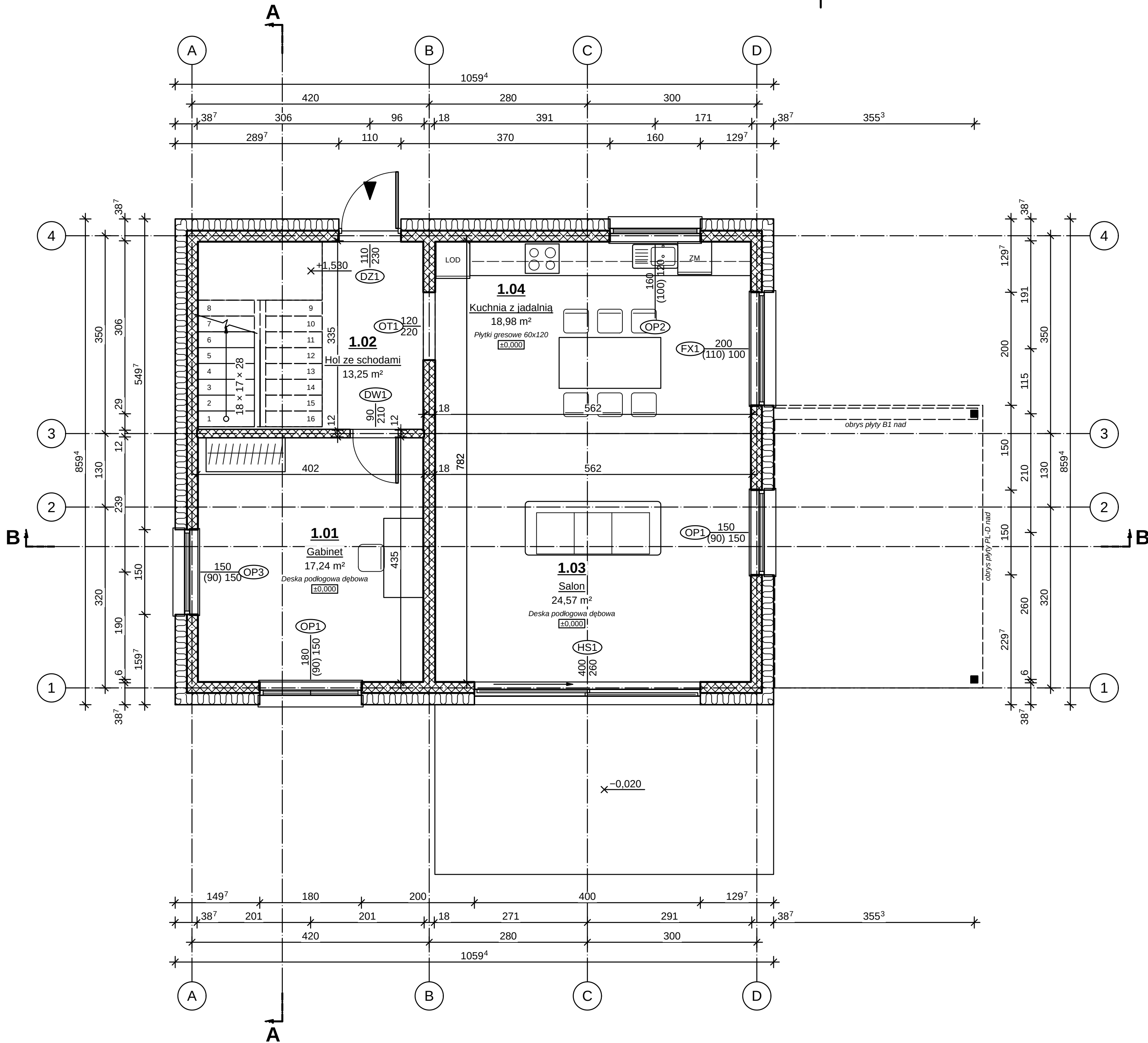
RZUT PARTERU 1:50
