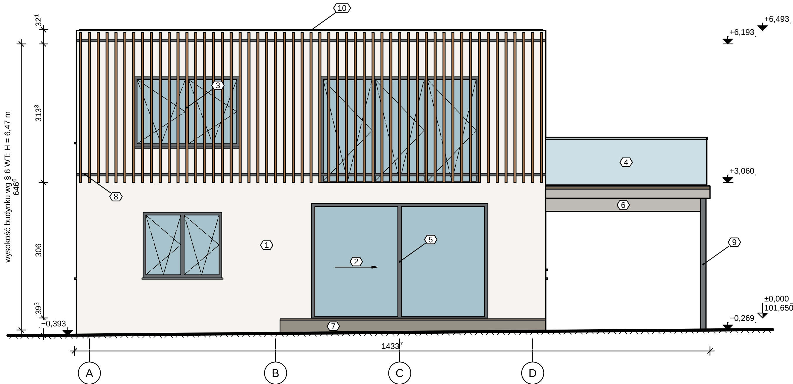
ELEWACJA POŁUDNIOWA 1:50
