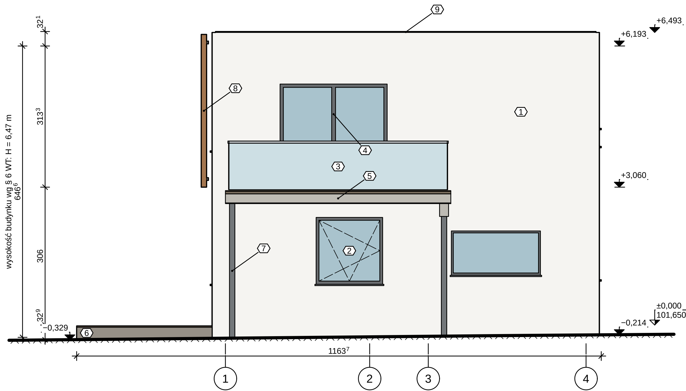
ELEWACJA WSCHODNIA 1:50
