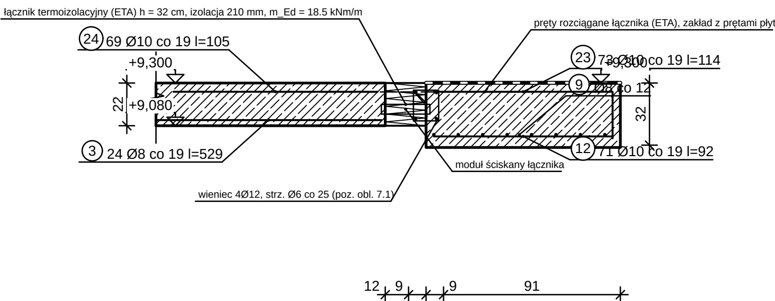
WĘZEL WSPORNIKA PL-3 — ŁĄCZNIK TERMOIZOLACYJNY 1:20
