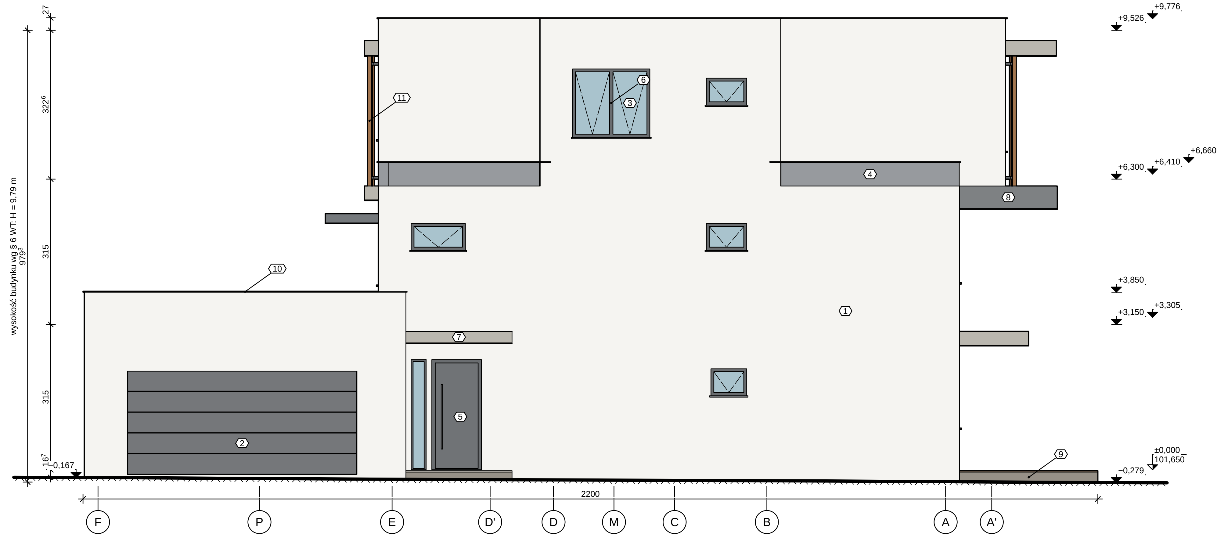
ELEWACJA PÓŁNOCNA 1:50
