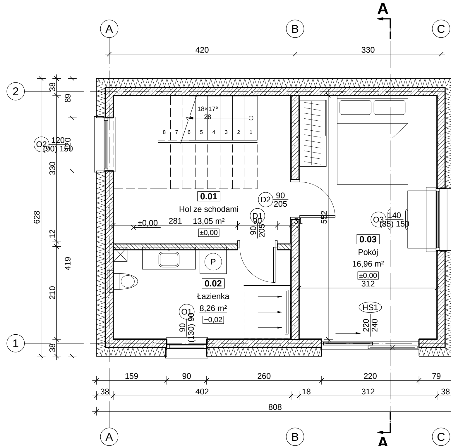
RZUT PARTERU — FRAGMENT 1:50
