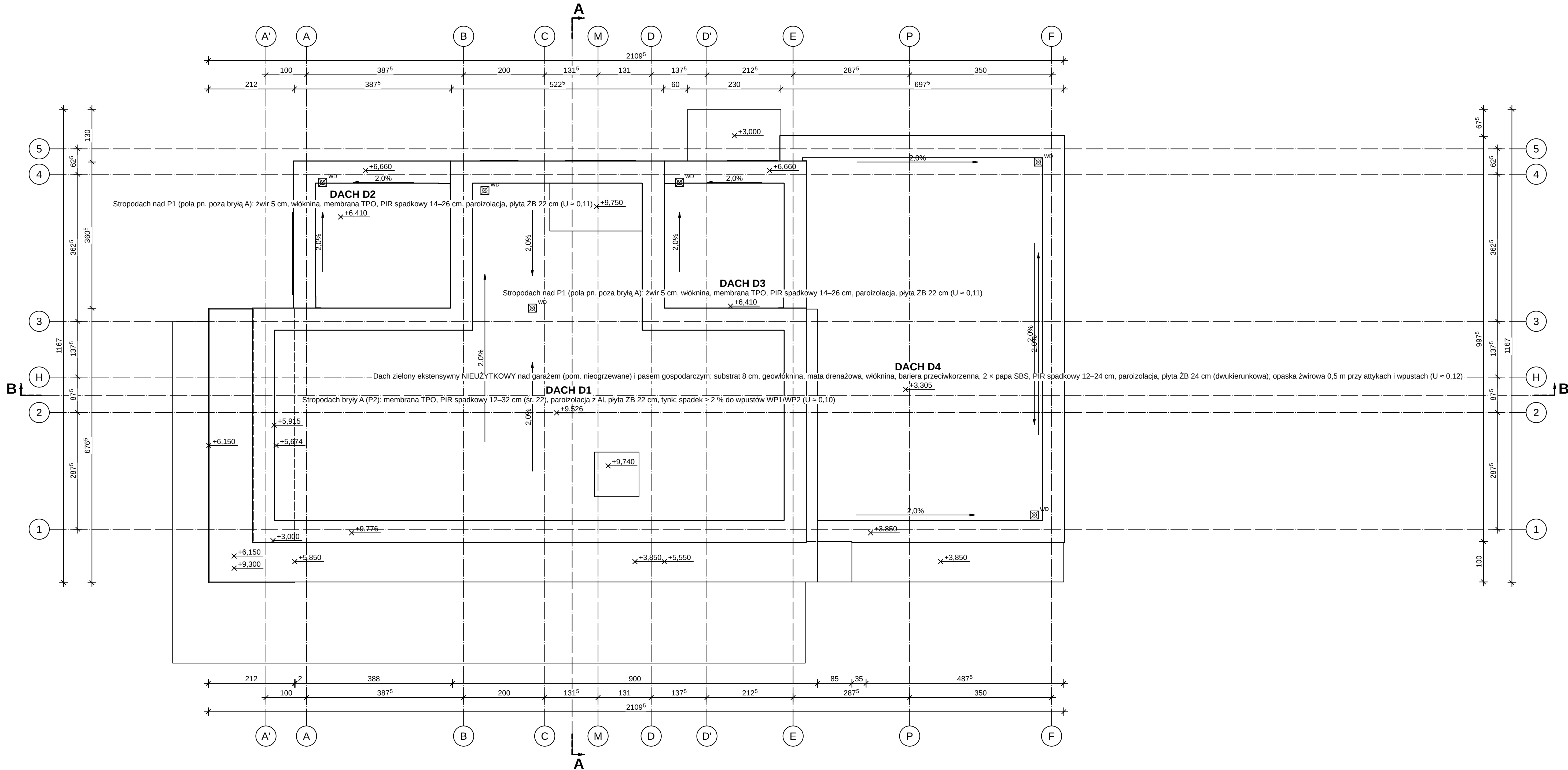
RZUT DACHU 1:50
