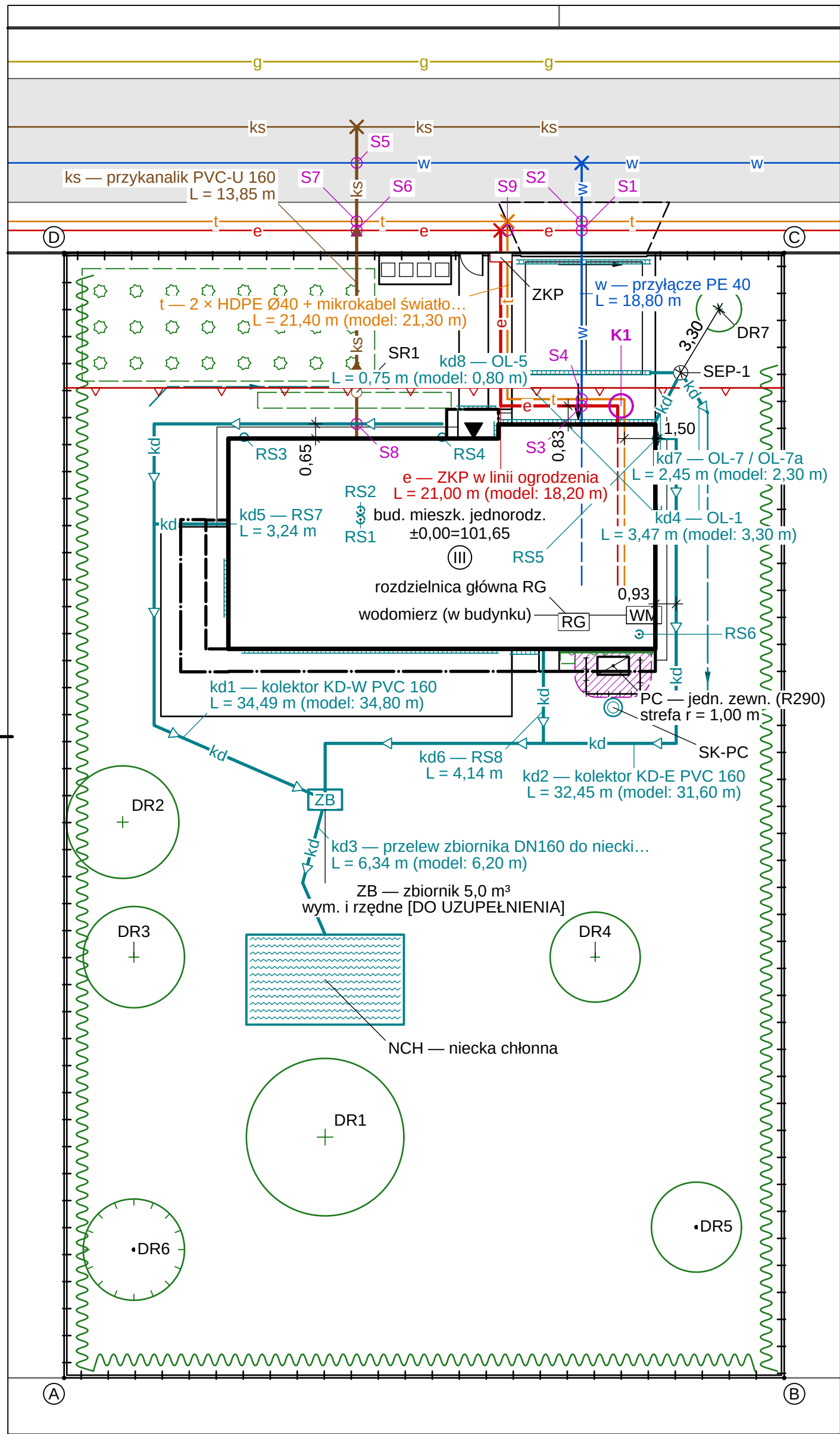
RYSUNEK KOORDYNACYJNY UZBROJENIA TERENU 1:200
