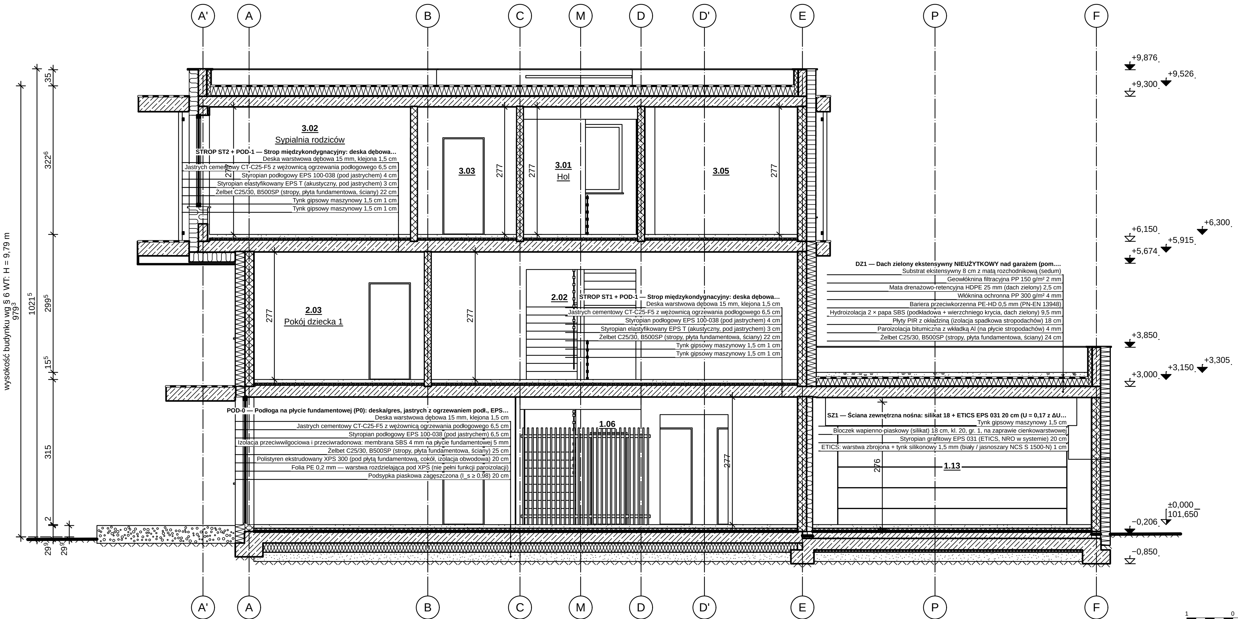
PRZĘKRÓJ B-B 1:50
