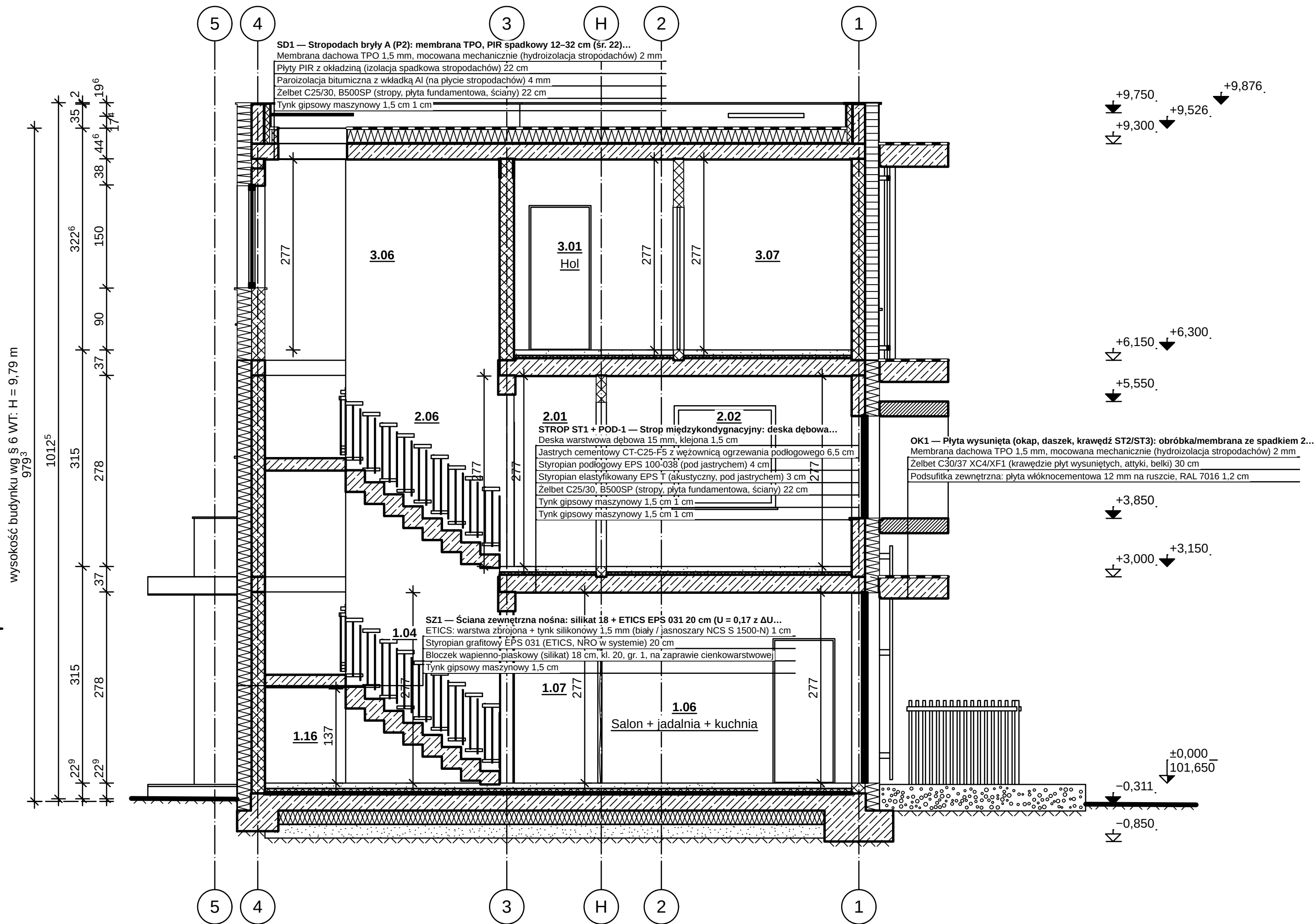
PRZĘKRÓJ A-A 1:50
