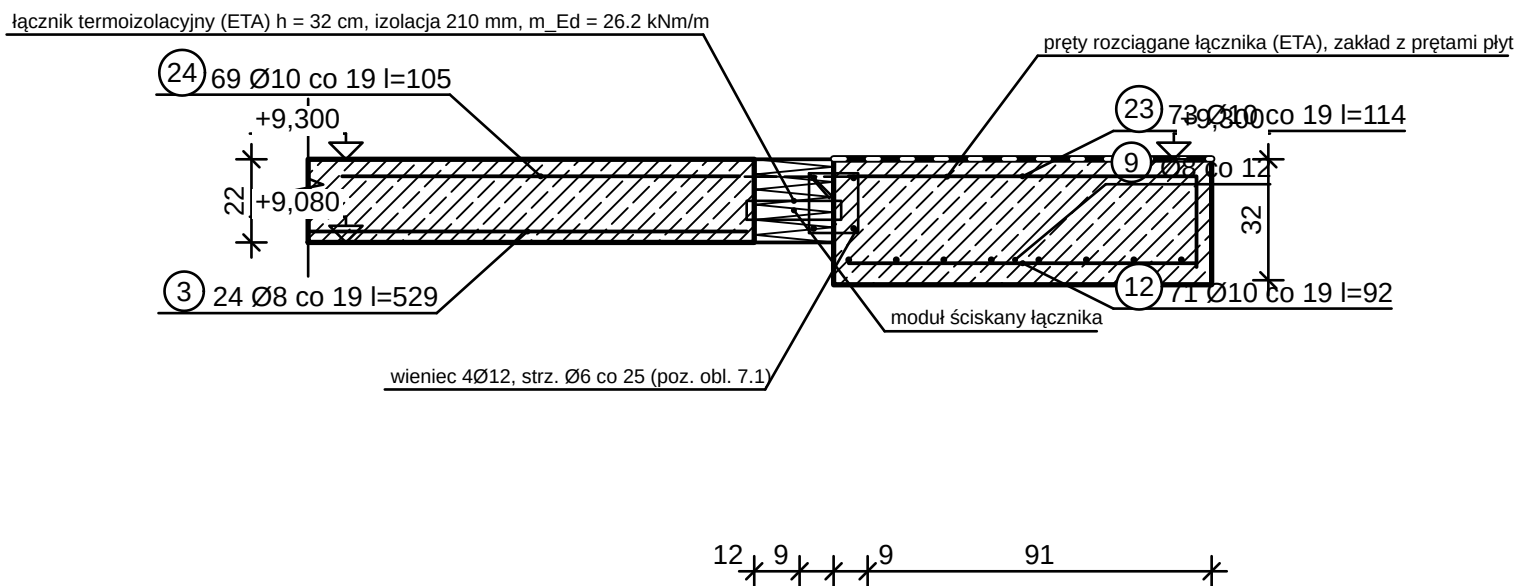
WĘZŁ WSPORNIKA PL-3 — ŁĄCZNIK TERMOIZOLACYJNY 1:20
