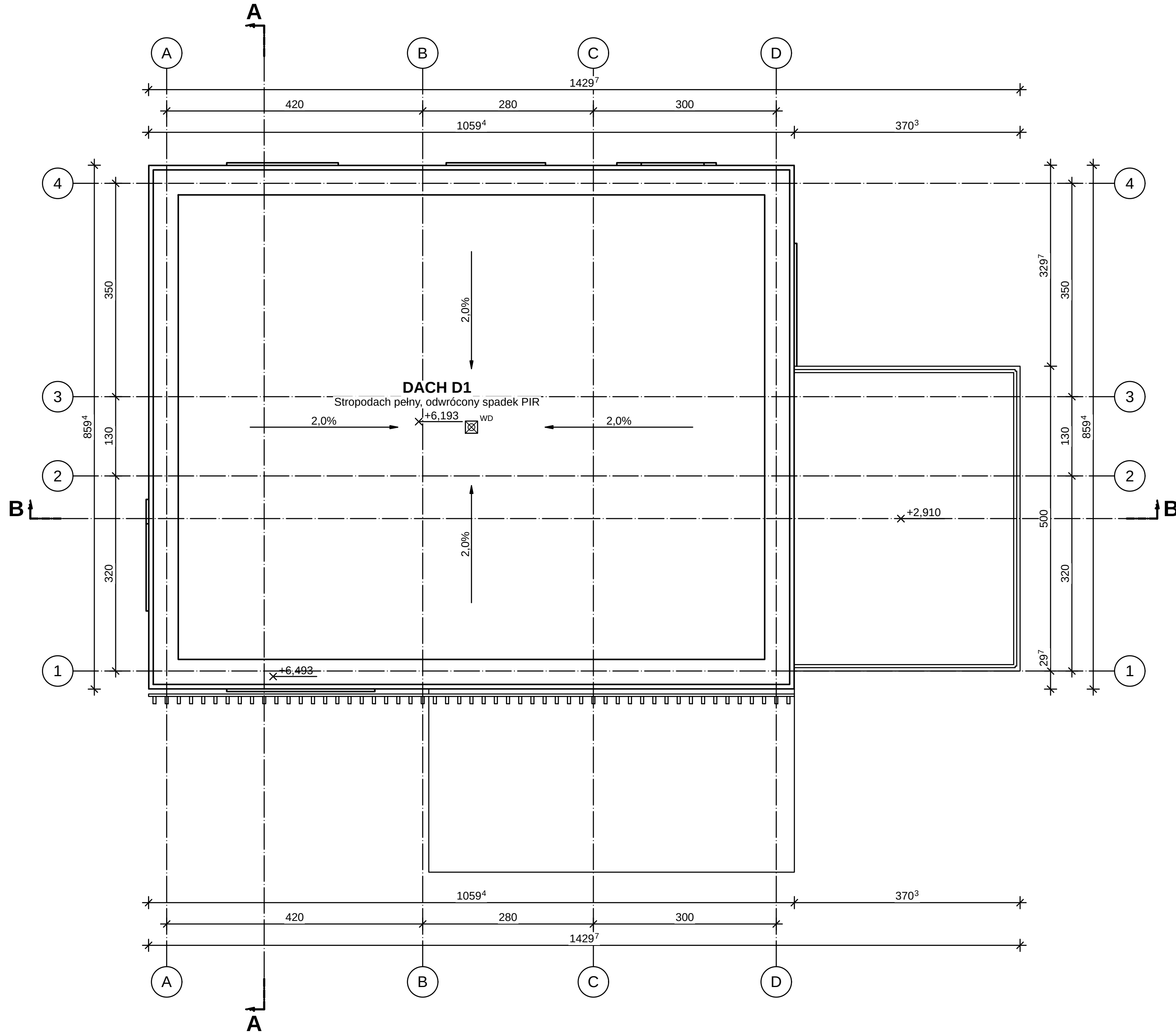
RZUT DACHU 1:50
