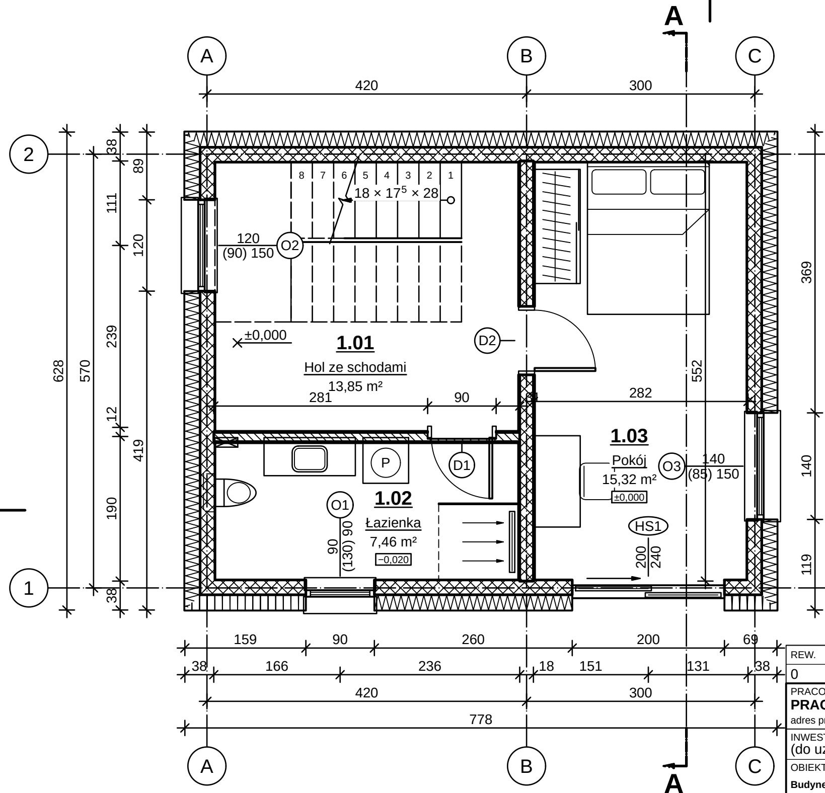
RZUT PARTERU — FRAGMENT 1:50
