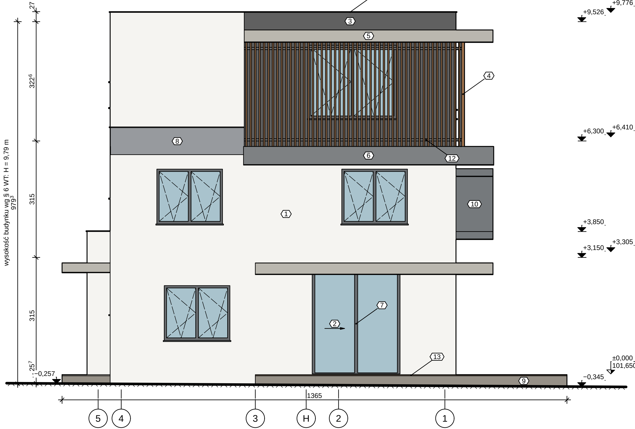
ELEWACJA ZACHODNIA 1:50
