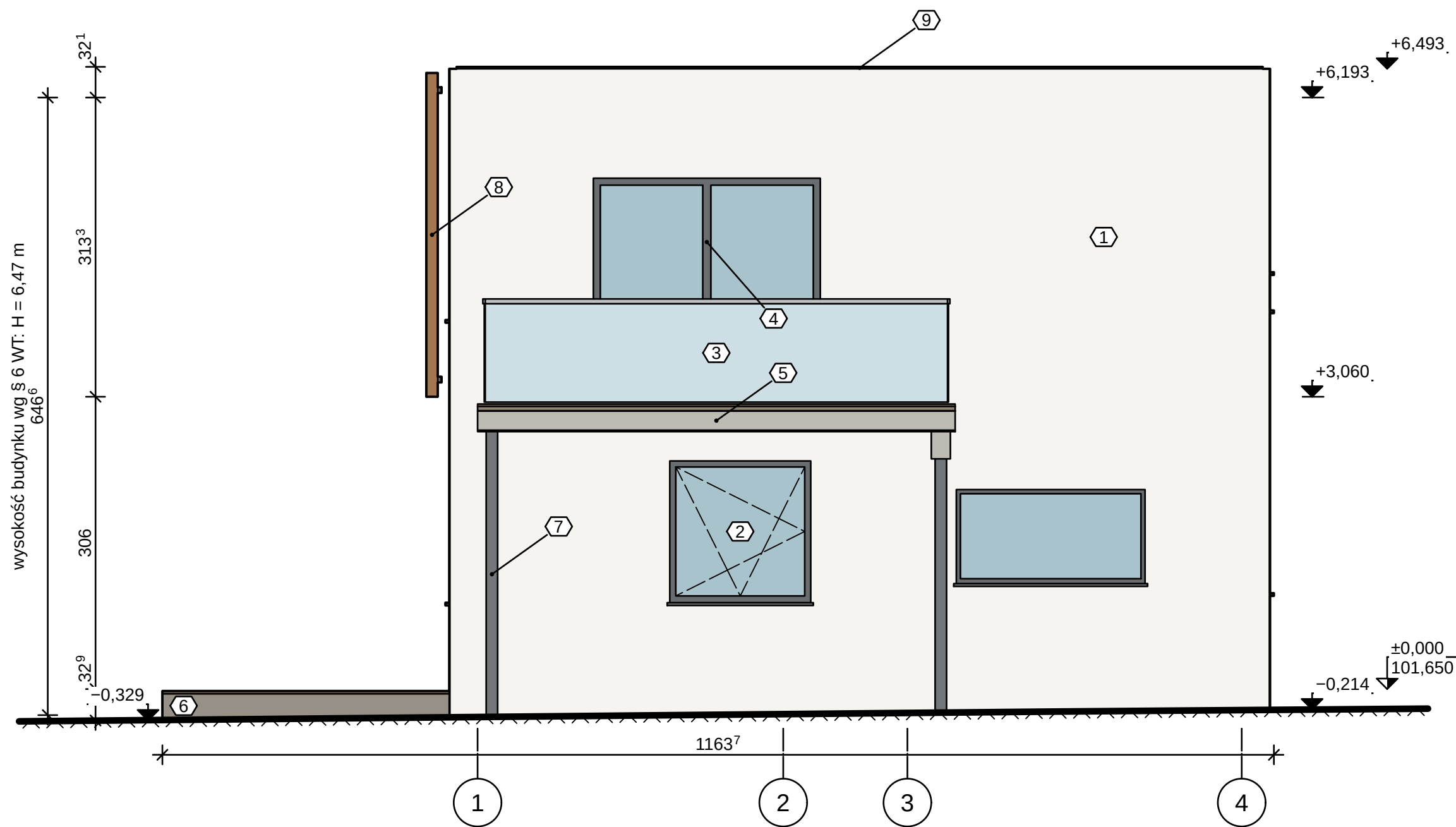
ELEWACJA WSCHODNIA 1:50
