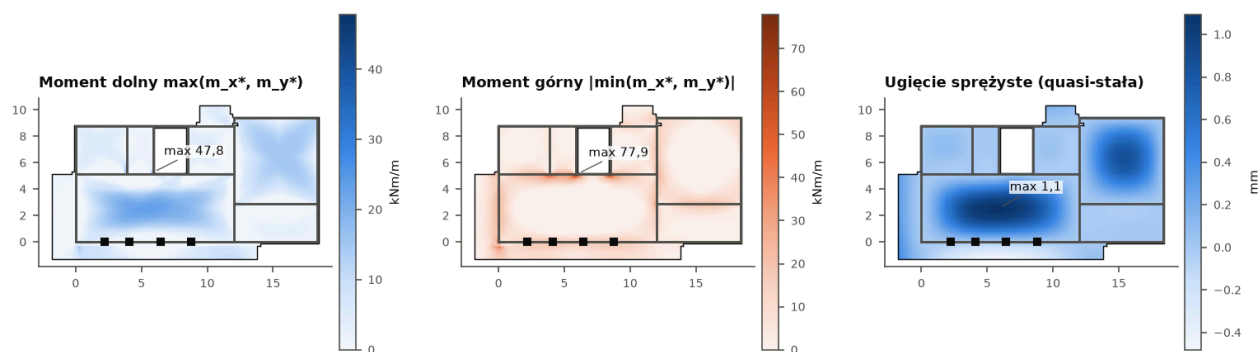
Ilustracja 19. Płyta ST1 + D4 + PL-E + PL-DA: momenty wymiarujące (obwiednia kombinacji 6.10a/b, obciążeń szachownicowych i sytuacji wyjątkowej) oraz ugięcie sprężyste od kombinacji quasi-stałej (bez zarysowania i pełzania — te w obliczeniach 7.4.3).
