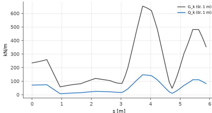
Ilustracja 93. Ława ZF9: przekrój poprzeczny i rozkład obciążenia wzdłuż ławy.
