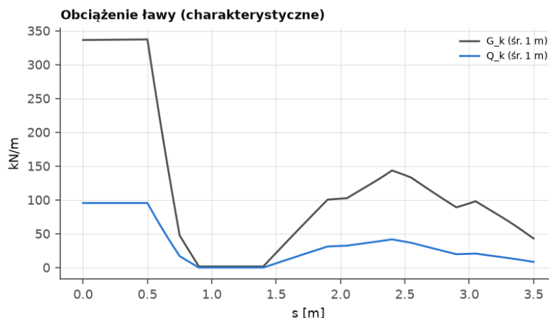
Ilustracja 95. Ława ZF11: przekrój poprzeczny i rozkład obciążenia wzdłuż ławy.
