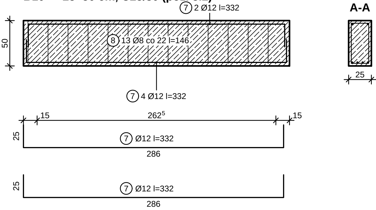
B10 — 25×50 cm, C25/30 (poz. 5.2)
