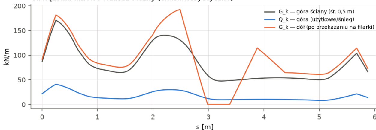
Ilustracja 81. Ściana S0-16: widok z otworami i rozkład obciążeń charakterystycznych wzdłuż osi.
