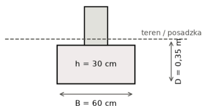
Ława ZF7 — przekrój
