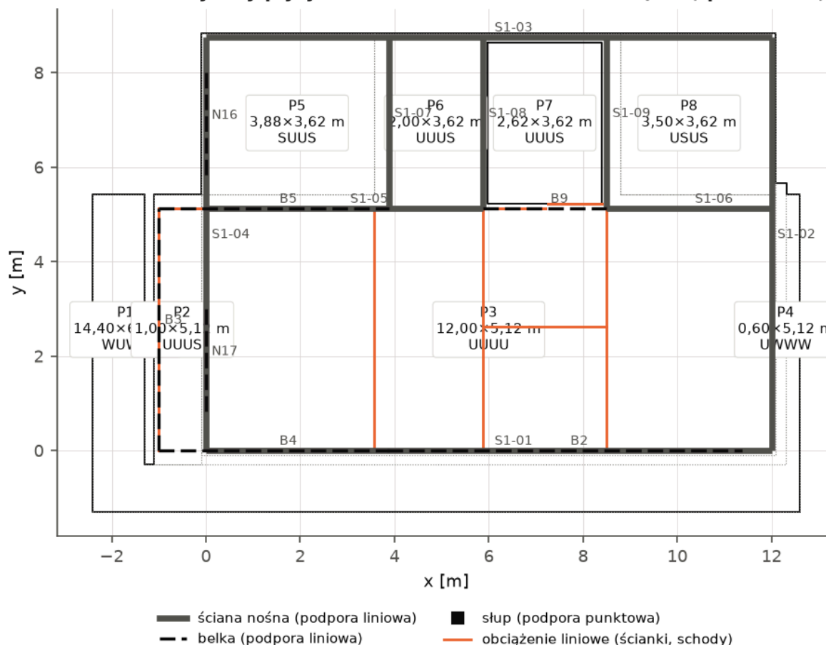
Schemat statyczny płyty ST2 + ST2Z + D2 + D3 + PL-2 (rzut; poziom +6,150 m)
