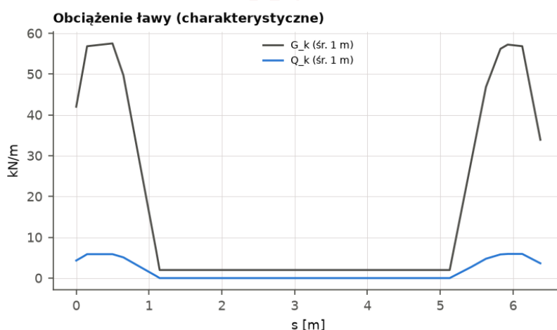
Ilustracja 89. Ława ZF5: przekrój poprzeczny i rozkład obciążenia wzdłuż ławy.
