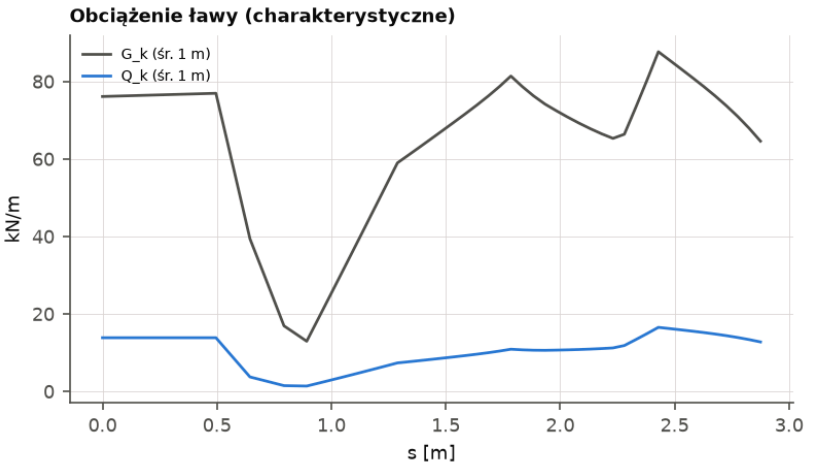
Ilustracja 99. Ława ZF15: przekrój poprzeczny i rozkład obciążenia wzdłuż ławy.
