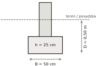
Ława ZF15 — przekrój
