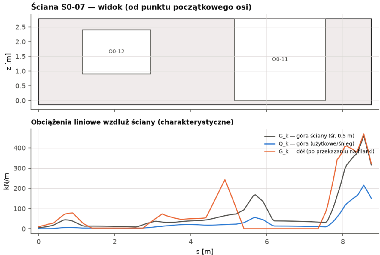
Ilustracja 75. Ściana S0-07: widok z otworami i rozkład obciążeń charakterystycznych wzdłuż osi.
