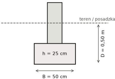
Ława ZF10 — przekrój
