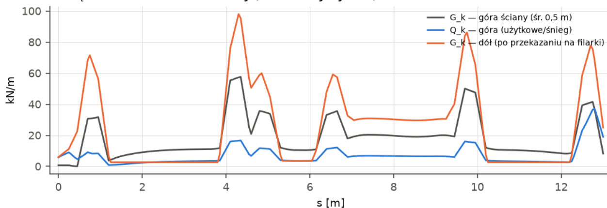
Ilustracja 55. Ściana S2-01: widok z otworami i rozkład obciążeń charakterystycznych wzdłuż osi.
