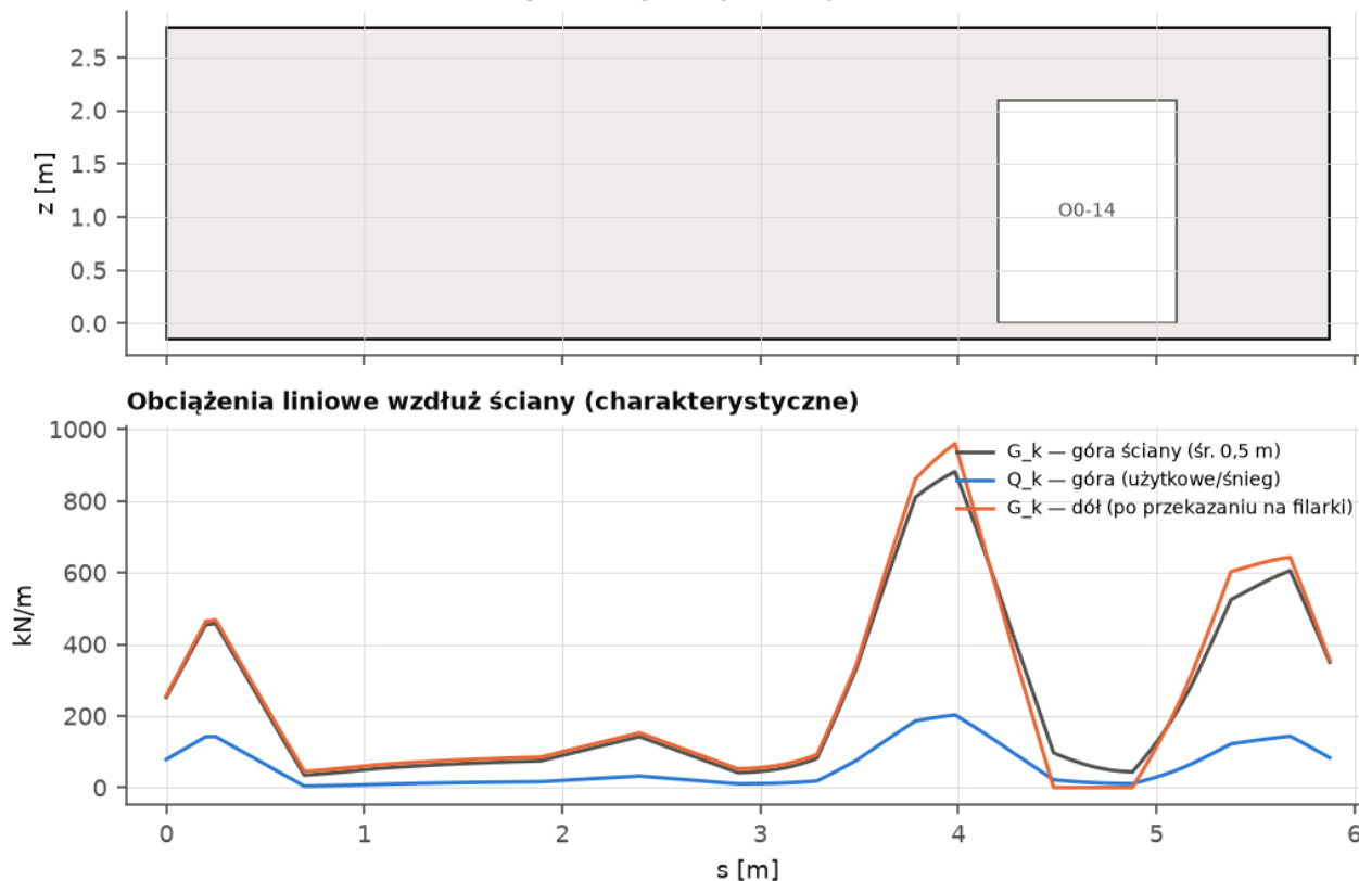
Ilustracja 76. Ściana S0-08: widok z otworami i rozkład obciążeń charakterystycznych wzdłuż osi.
