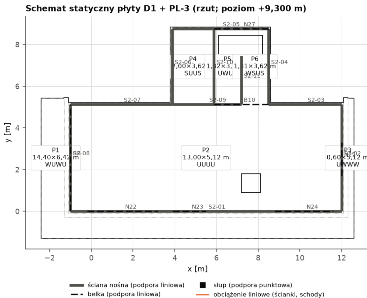
Ilustracja 3. Schemat statyczny płyty D1 + PL-3: pola (P — wymiary, warunki brzegowe x=0/x=l_x/y=0/y=l_y : S — podparcie swobodne, U — ciągłość/utwierdzenie, W — brzeg swobodny/niepełny), podpory.
