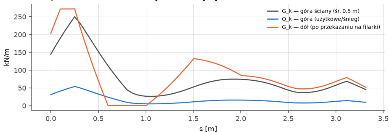
Ilustracja 62. Ściana S2-09: widok z otworami i rozkład obciążeń charakterystycznych wzdłuż osi.
