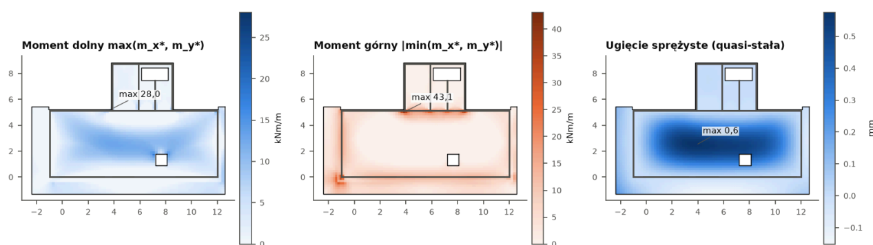
Ilustracja 4. Płyta D1 + PL-3: momenty wymiarujące (obwiednia kombinacji 6.10a/b, obciążeń szachownicowych i sytuacji wyjątkowej) oraz ugięcie sprężyste od kombinacji quasi-stałej (bez zarysowania i pełzania — te w obliczeniach 7.4.3).
