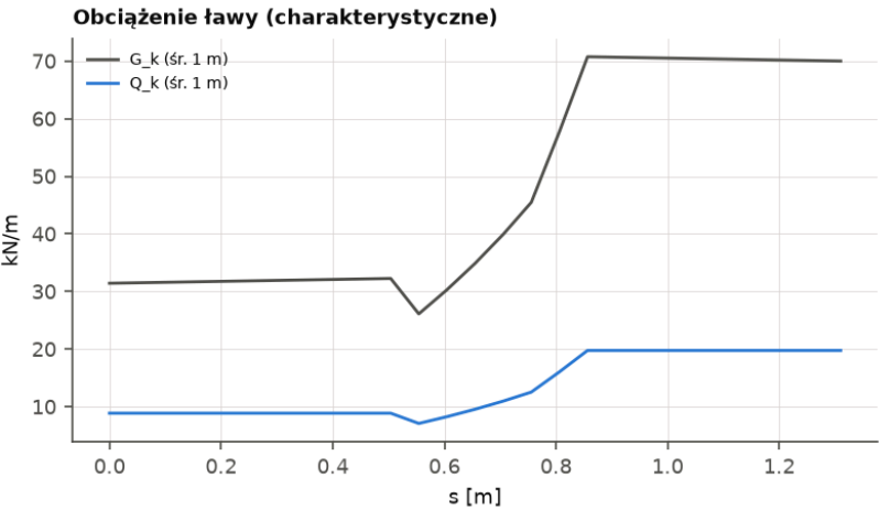
Ilustracja 94. Ława ZF10: przekrój poprzeczny i rozkład obciążenia wzdłuż ławy.
