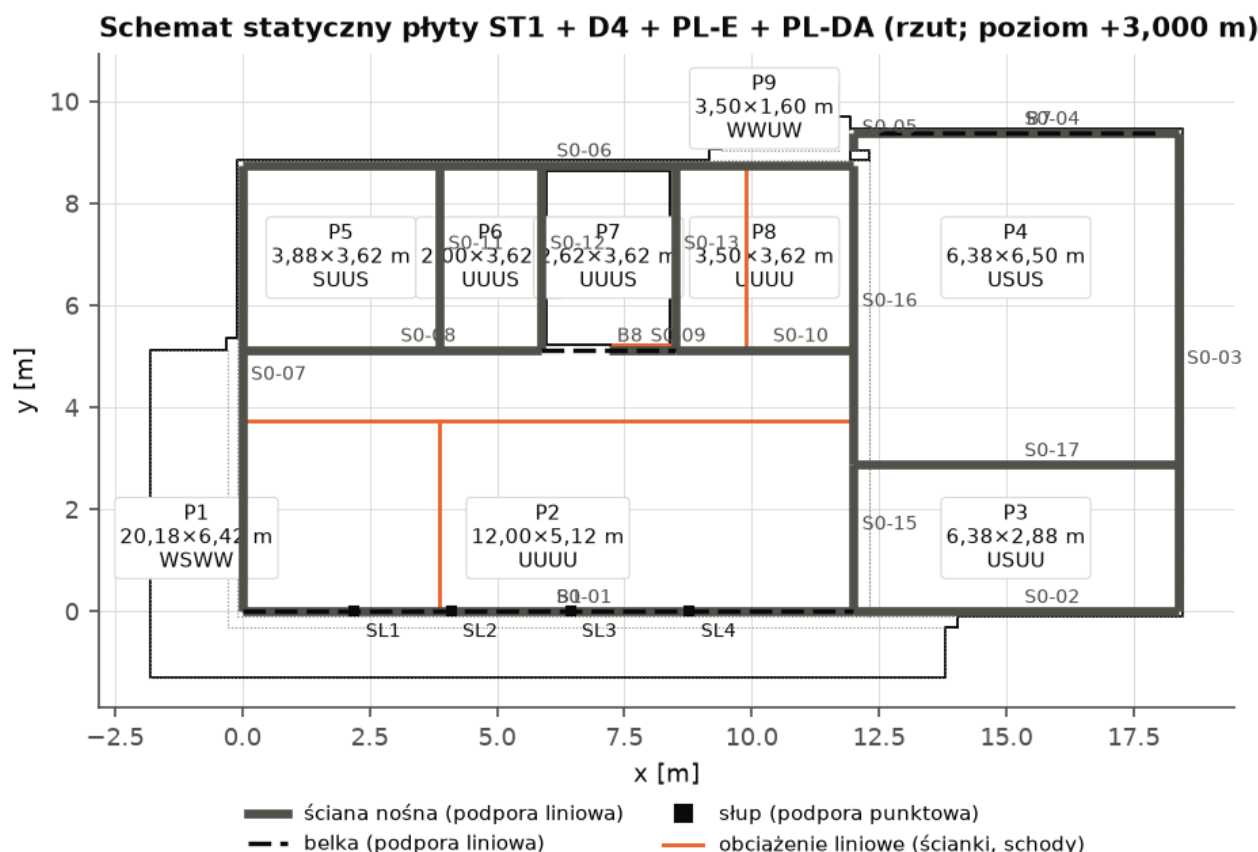
Ilustracja 18. Schemat statyczny płyty ST1 + D4 + PL-E + PL-DA: pola (P — wymiary, warunki brzegowe x=0/x=l , y=0/y=l : S — podparcie swobodne, U — ciągłość/utwierdzenie, W — brzeg swobodny/niepełny), podpory.
