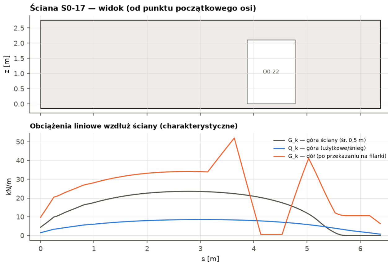
Ilustracja 86. Ściana S0-17: widok z otworami i rozkład obciążeń charakterystycznych wzdłuż osi.
