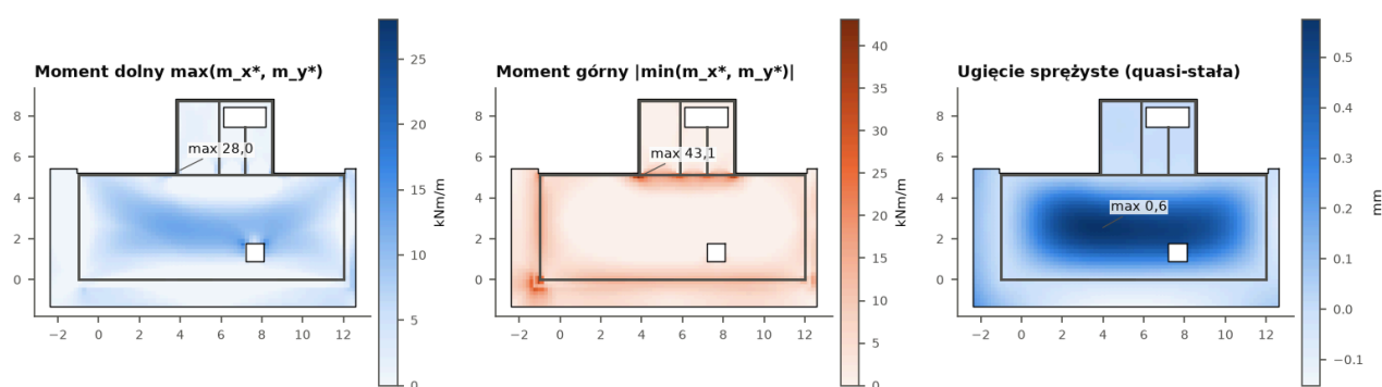
Ilustracja 21. Płyta D1 + PL-3: momenty wymiarujące (obwiednia kombinacji 6.10a/b, obciążeń szachownicowych i sytuacji wyjątkowej) oraz ugięcie sprężyste od kombinacji quasi-stałej (bez zarysowania i pełzania — te w obliczeniach 7.4.3).
