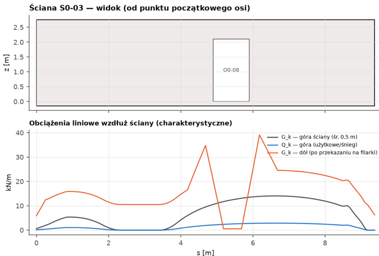
Ilustracja 83. Ściana S0-03: widok z otworami i rozkład obciążeń charakterystycznych wzdłuż osi.
