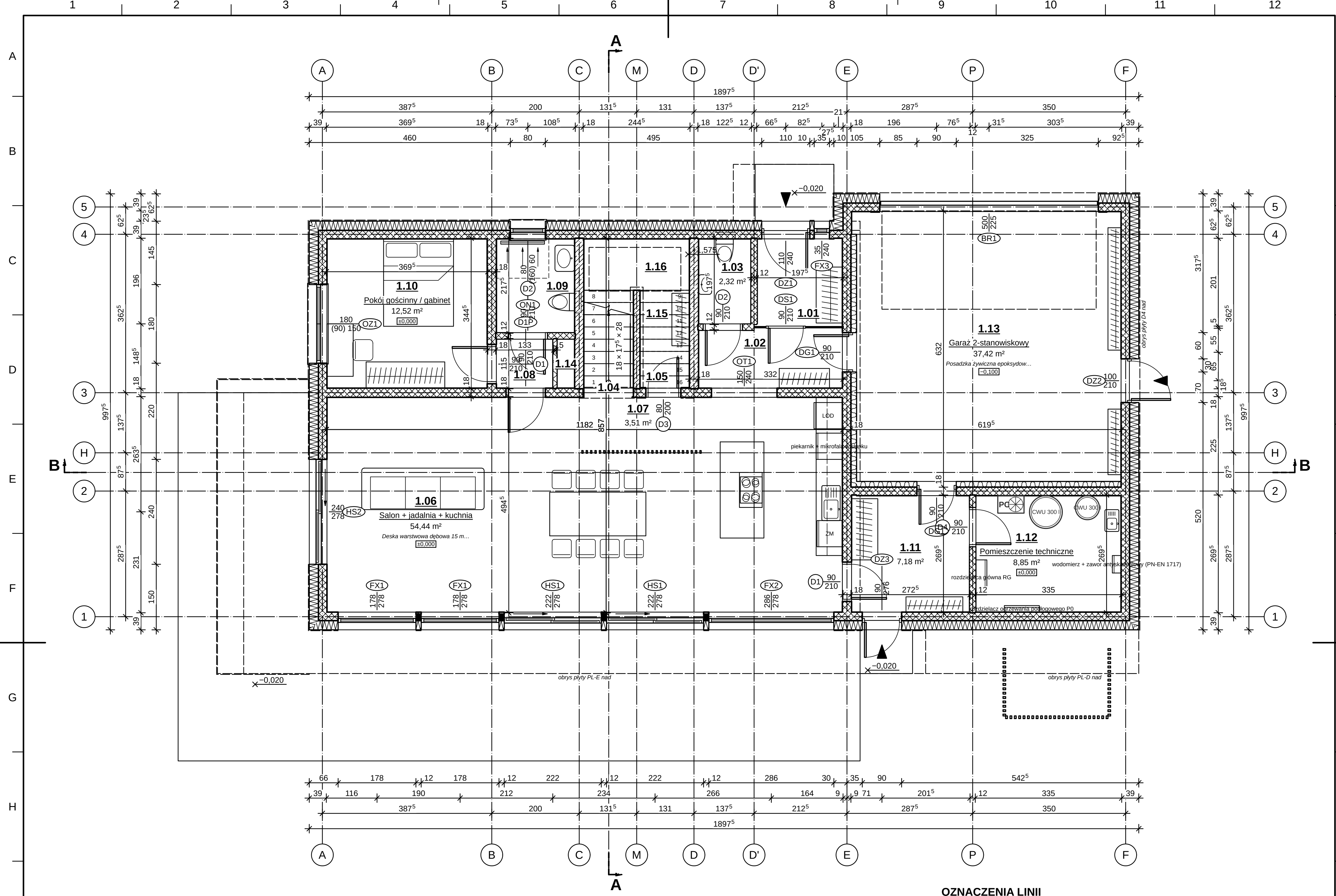
RZUT PARTERU 1:50
