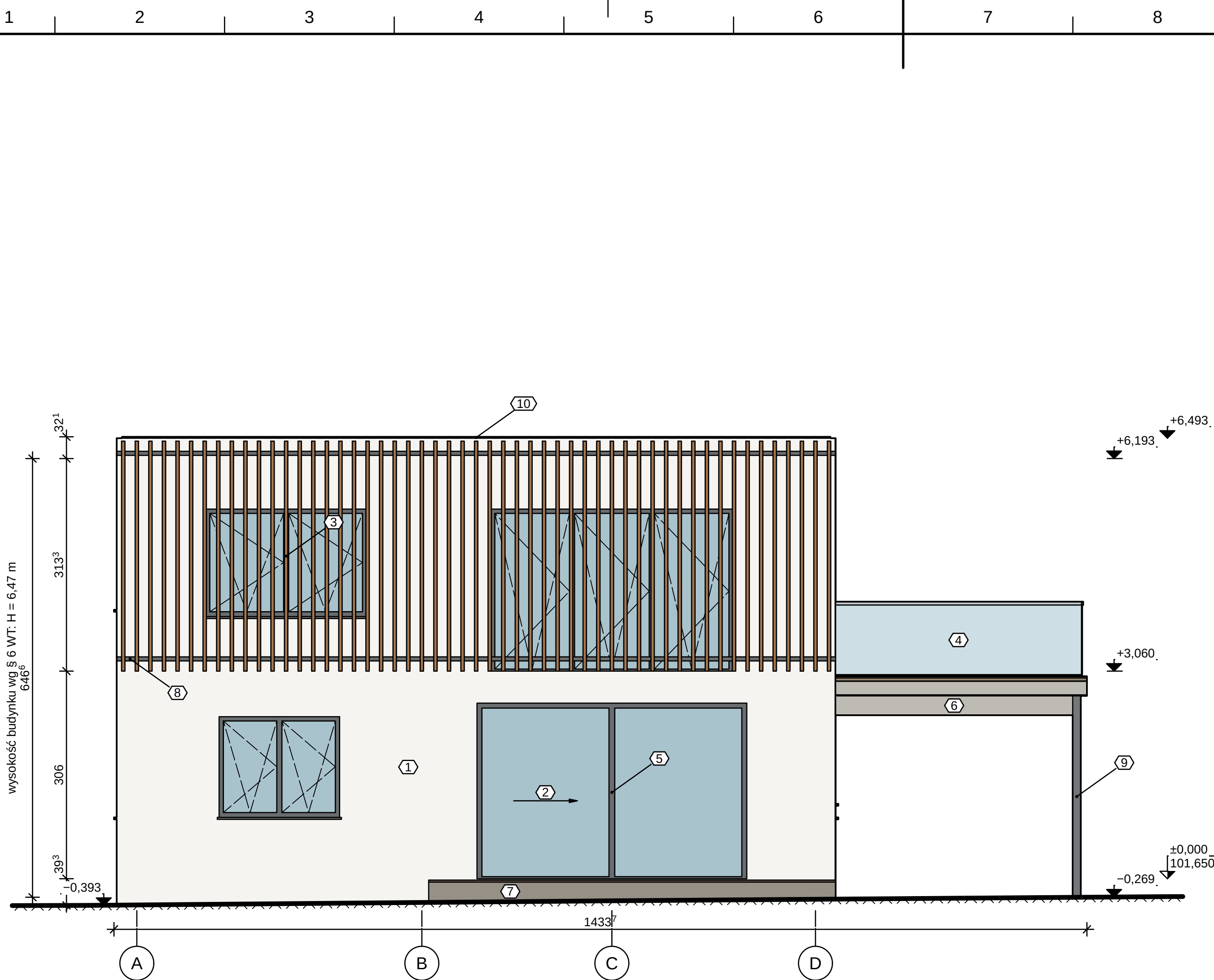
ELEWACJA POŁUDNIOWA 1:50
