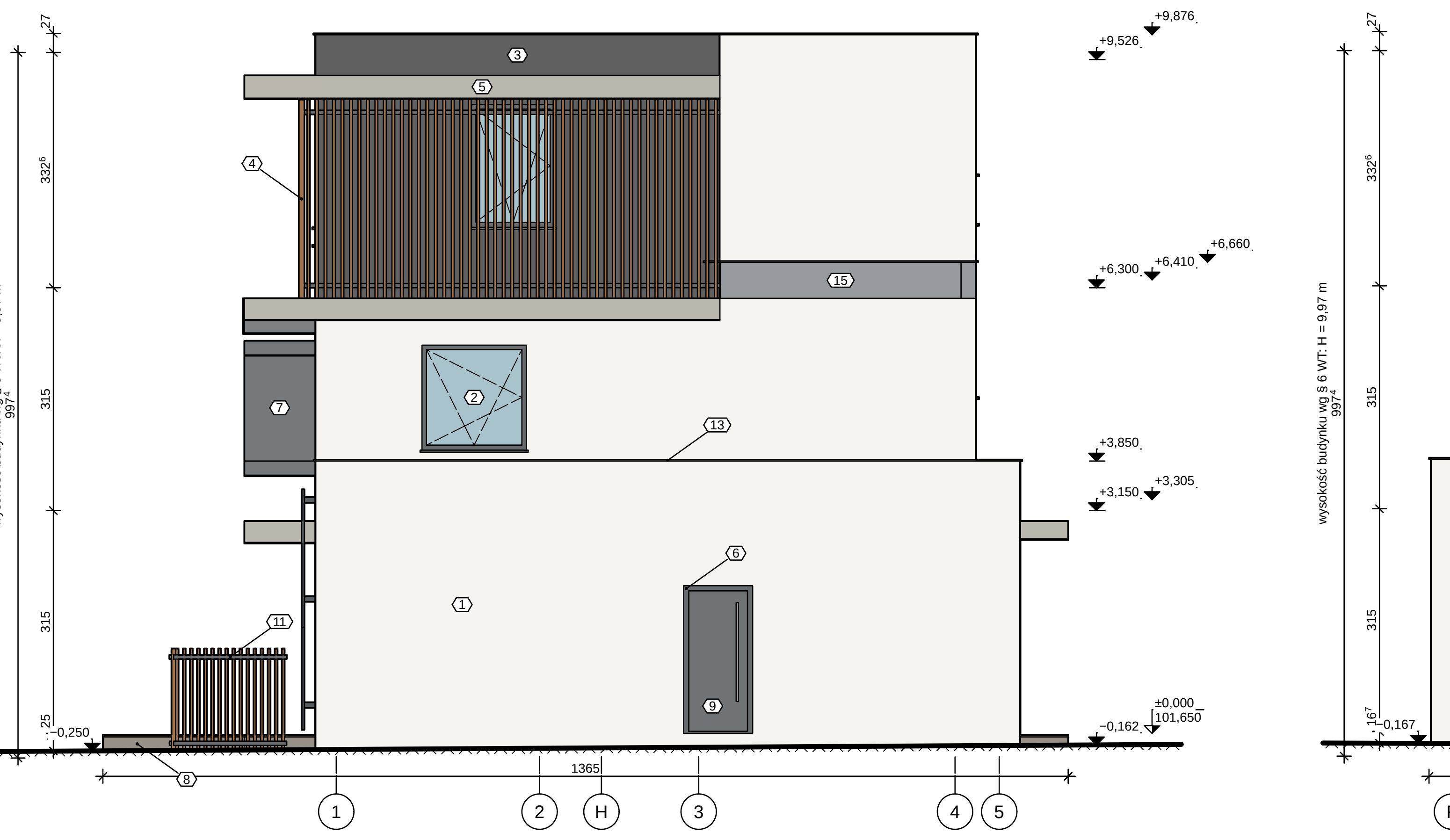
ELEWACJA WSCHODNIA 1:50
