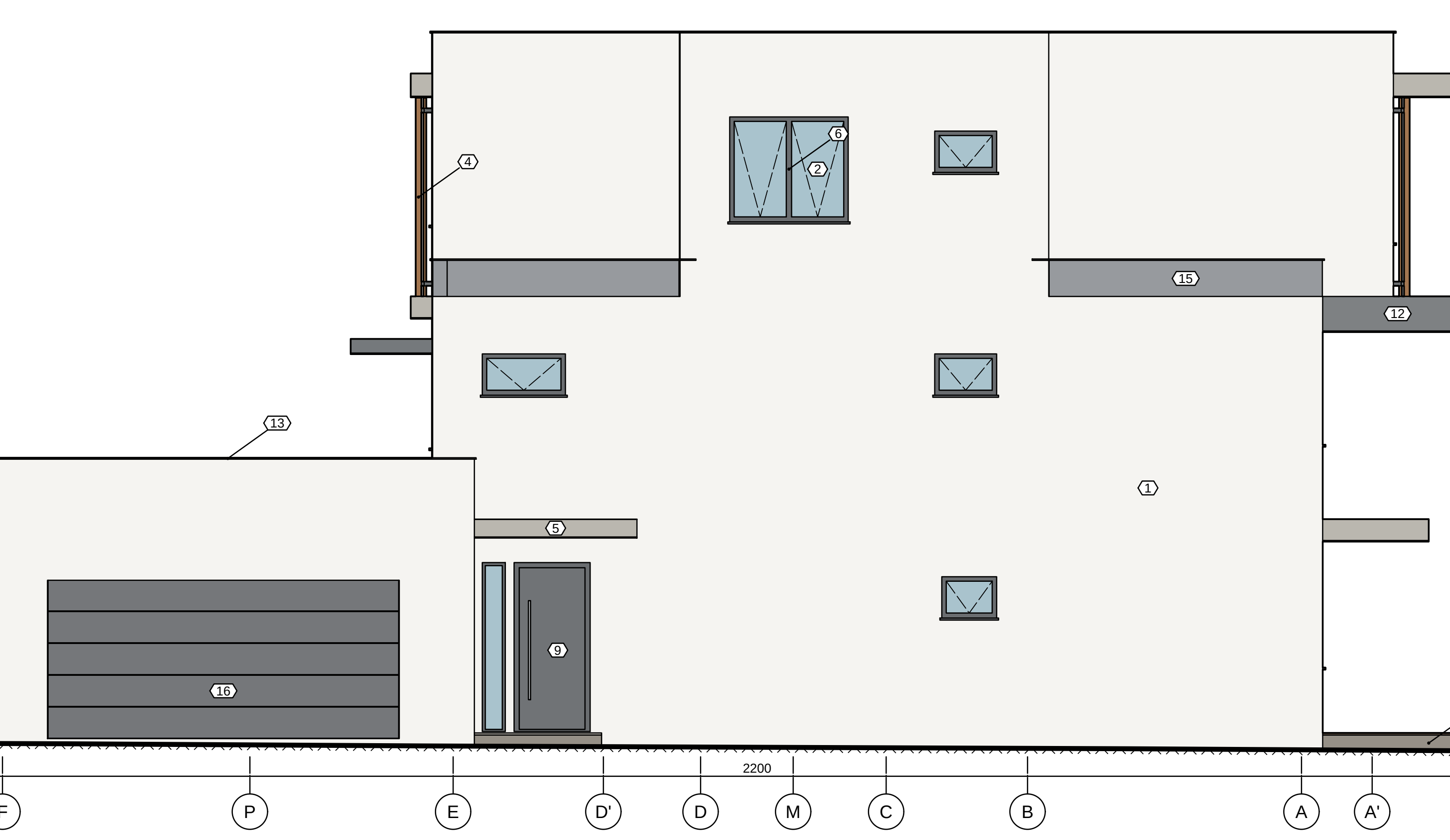
ELEWACJA PÓŁNOCNA (OD ULICY) 1:50
