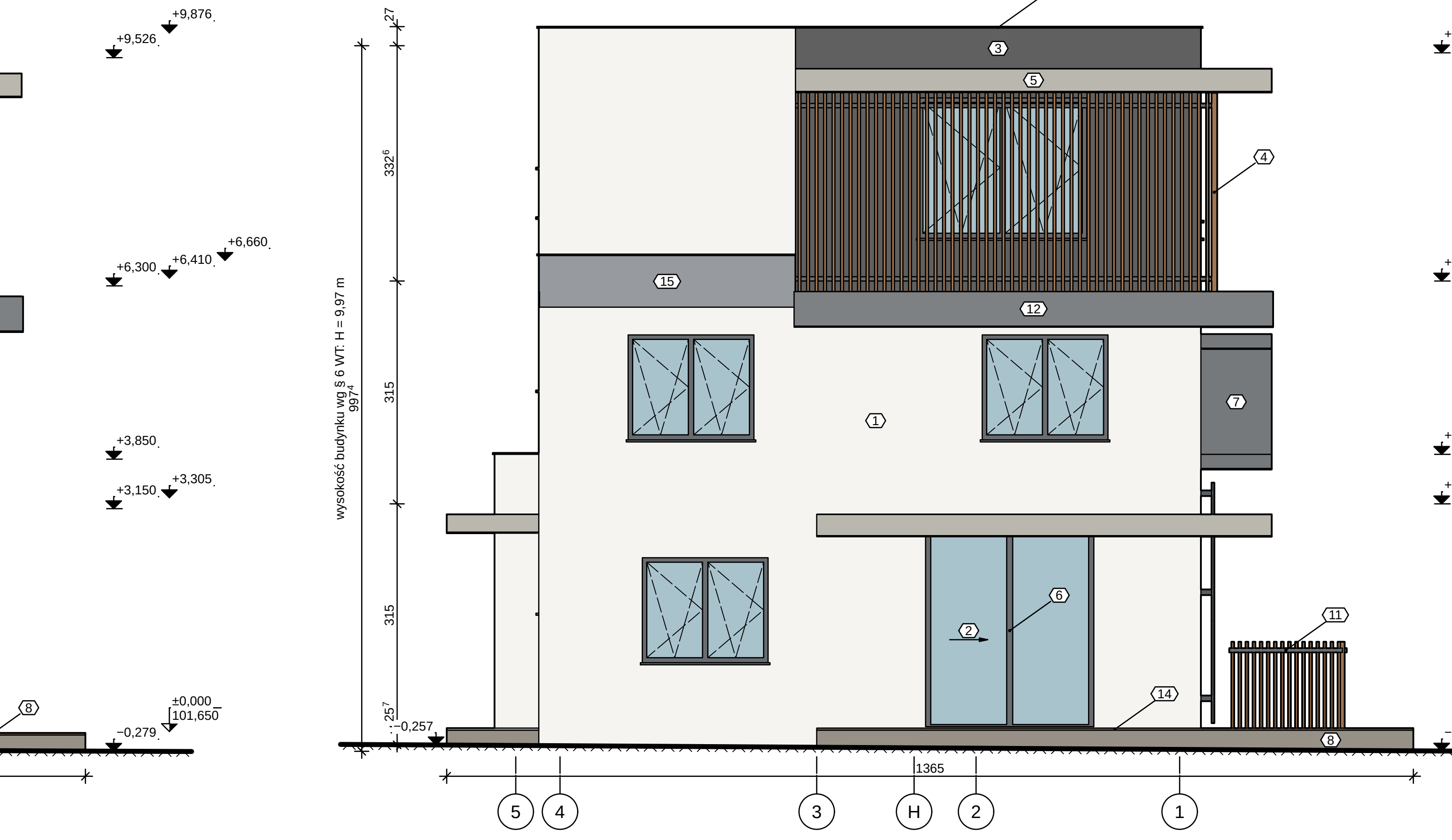
ELEWACJA ZACHODNIA 1:50
