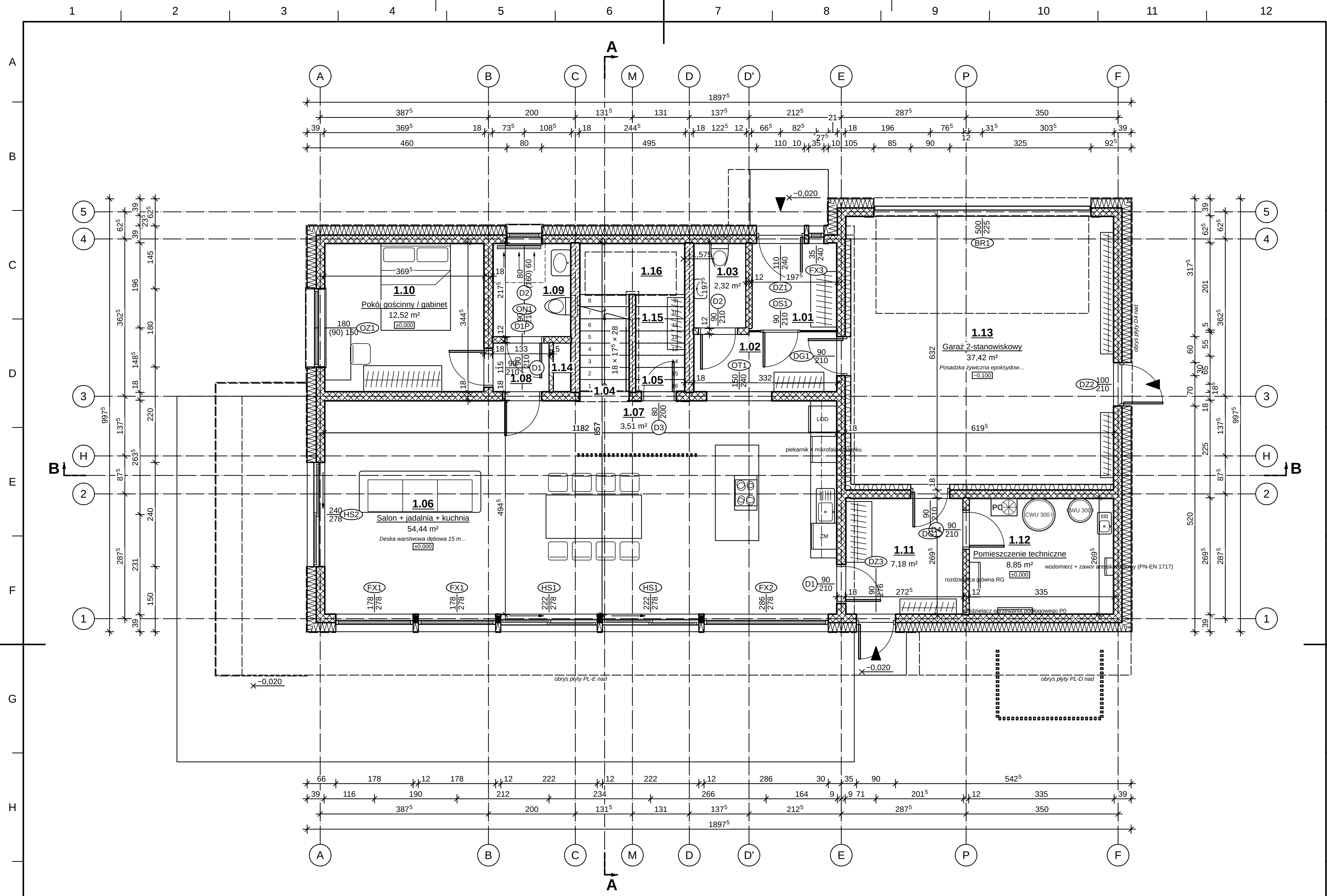
RZUT PARTERU 1:50
