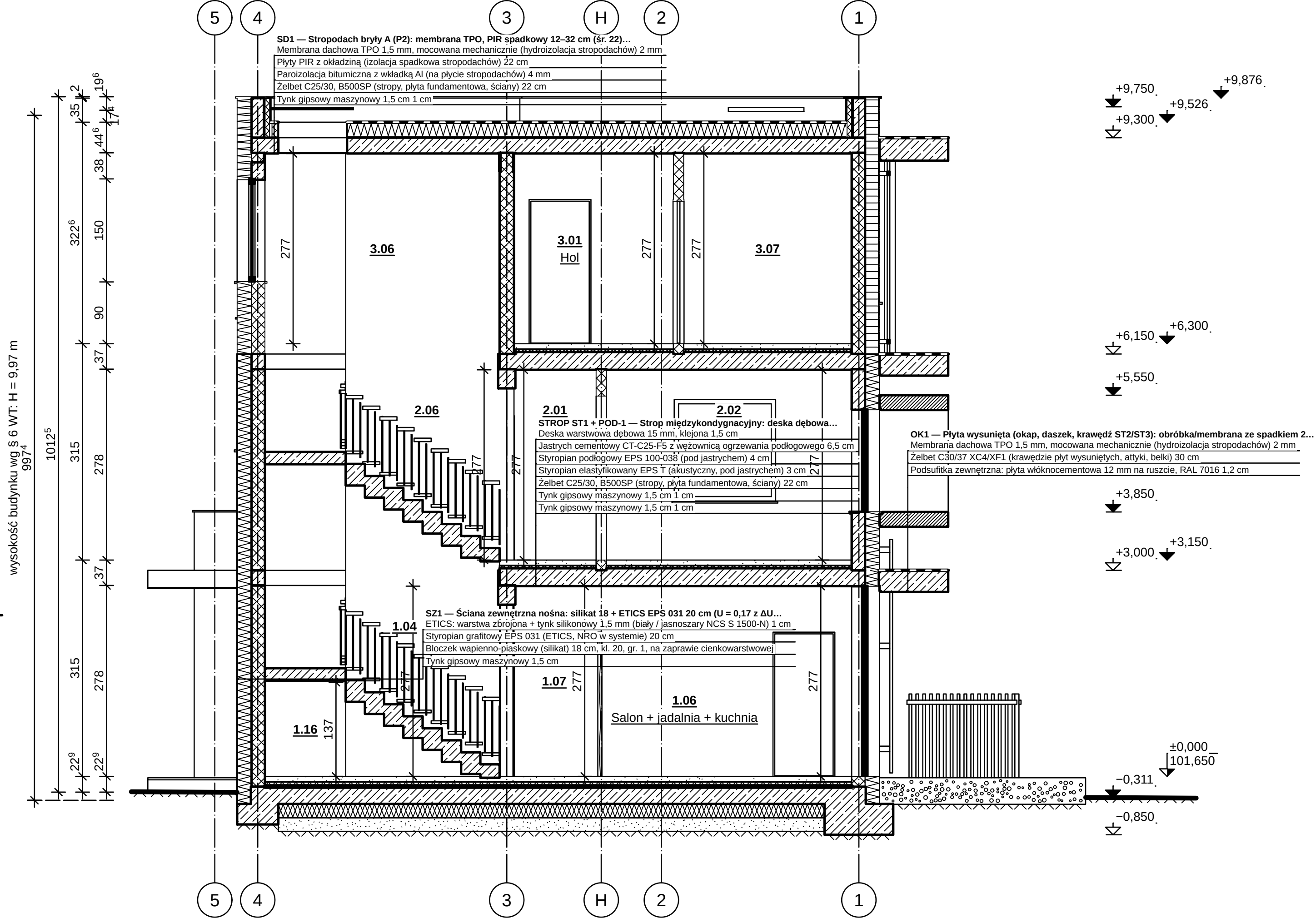
PRZĘKRÓJ A-A 1:50
