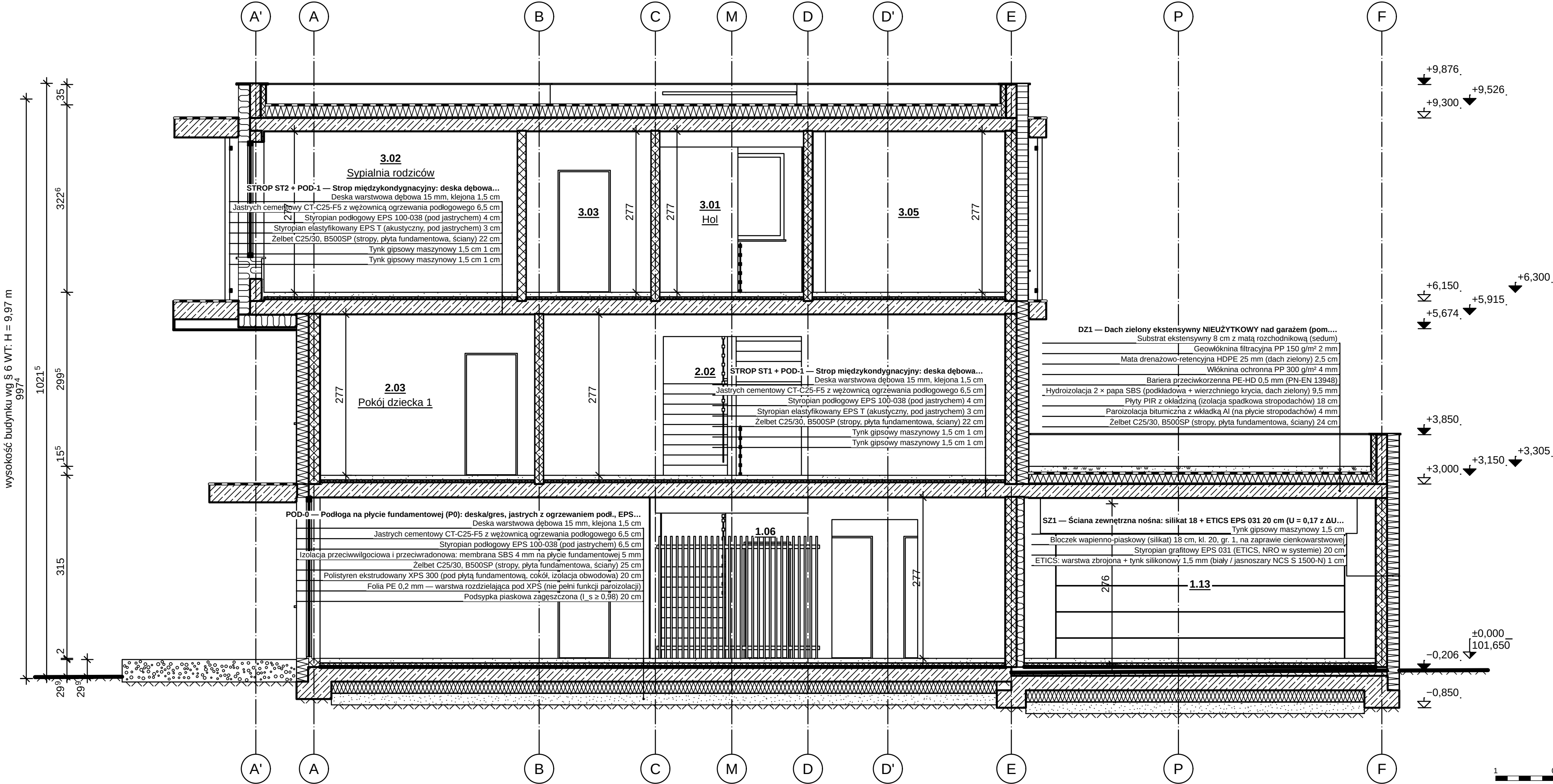
PRZĘKRÓJ B-B 1:50
