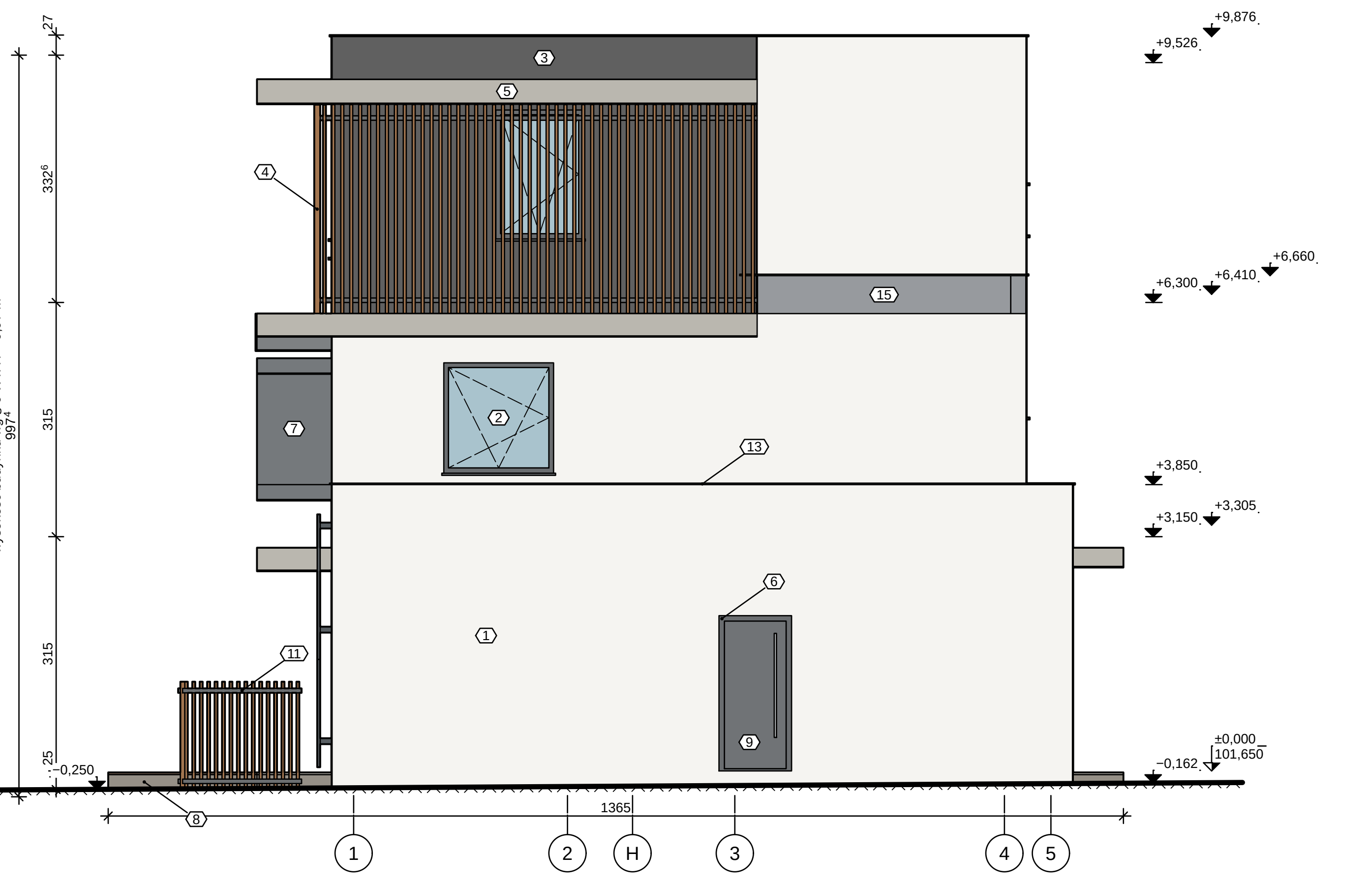
ELEWACJA WSCHODNIA 1:50
