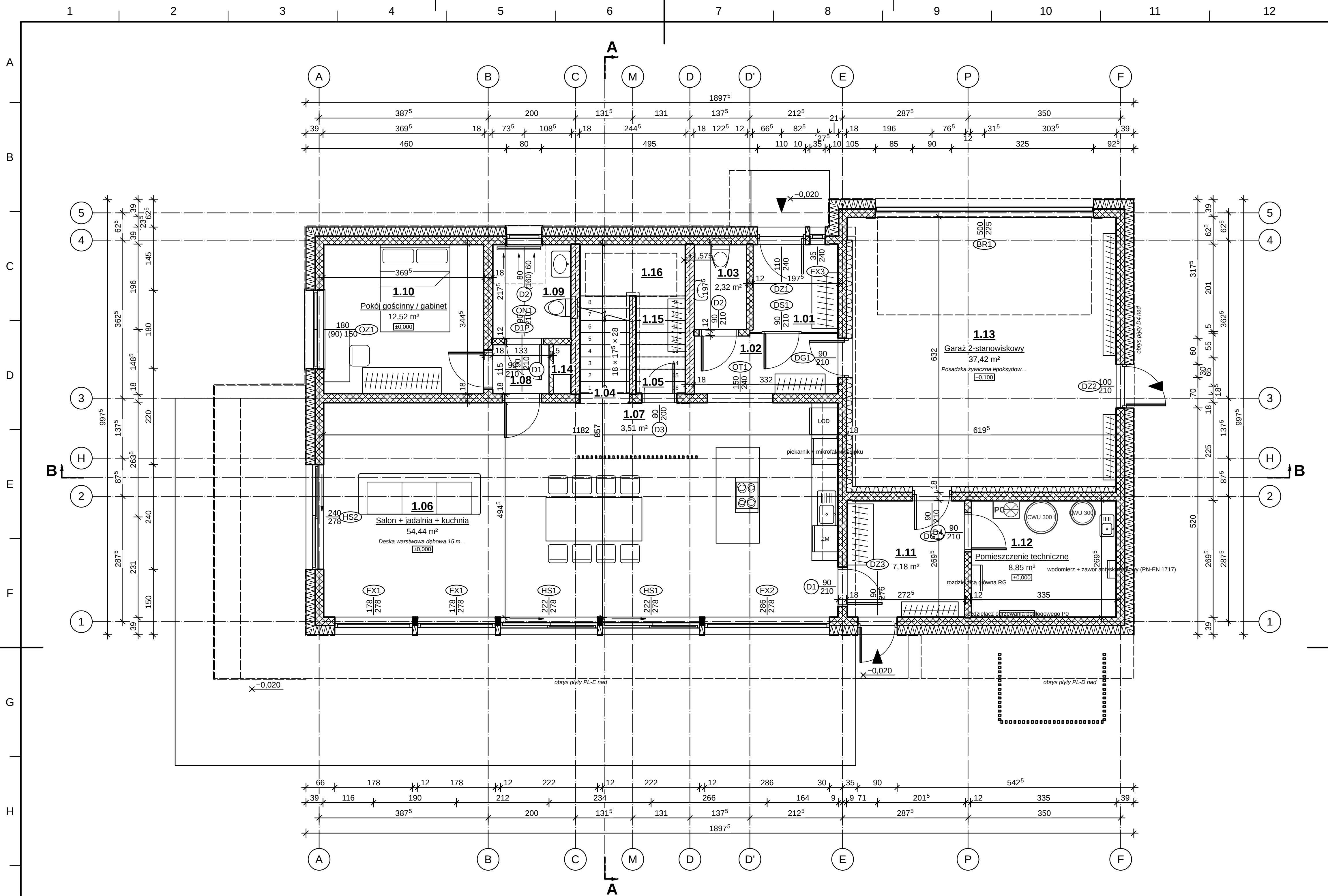
RZUT PARTERU 1:50
