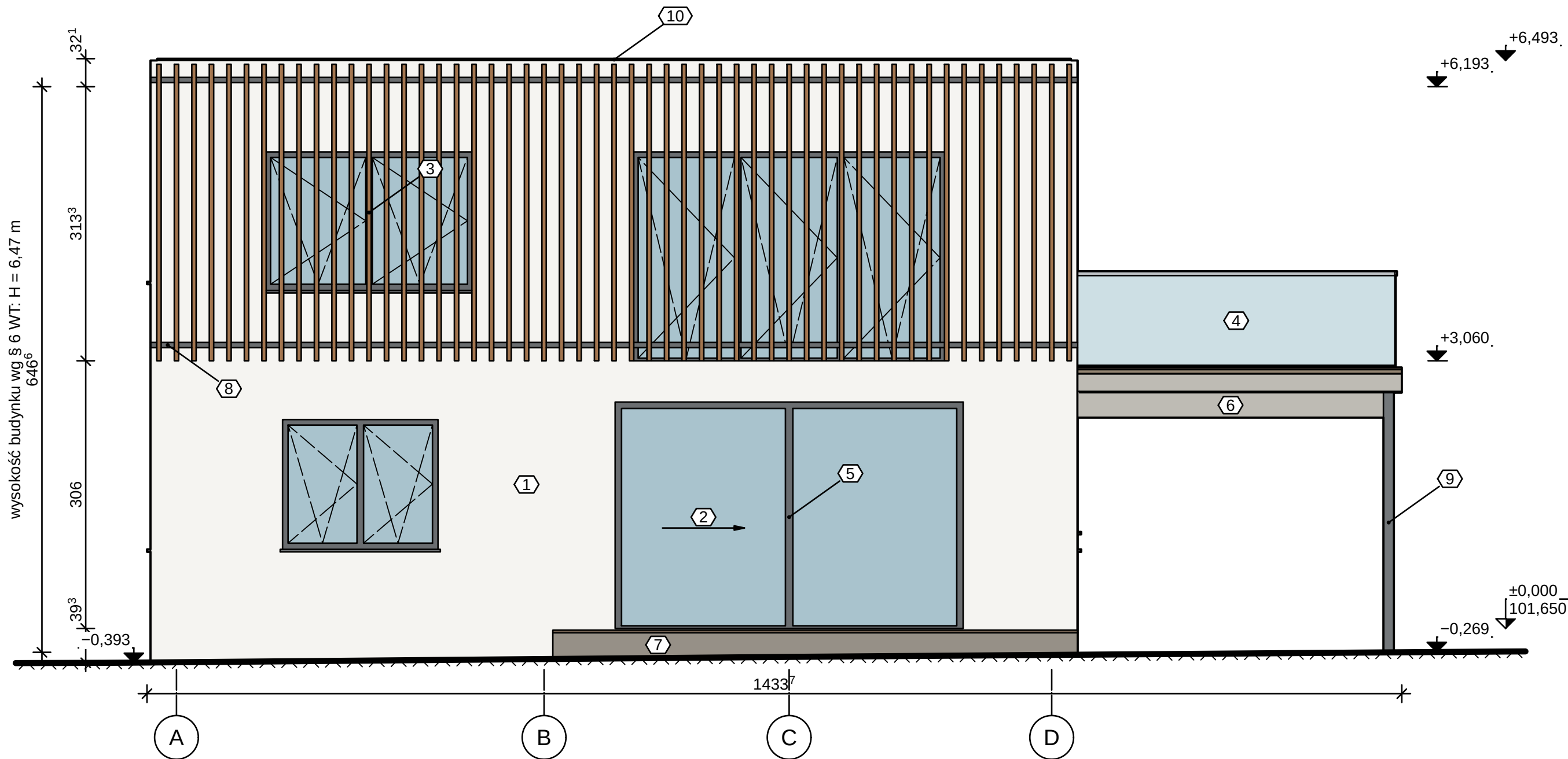
ELEWACJA POŁUDNIOWA 1:50
