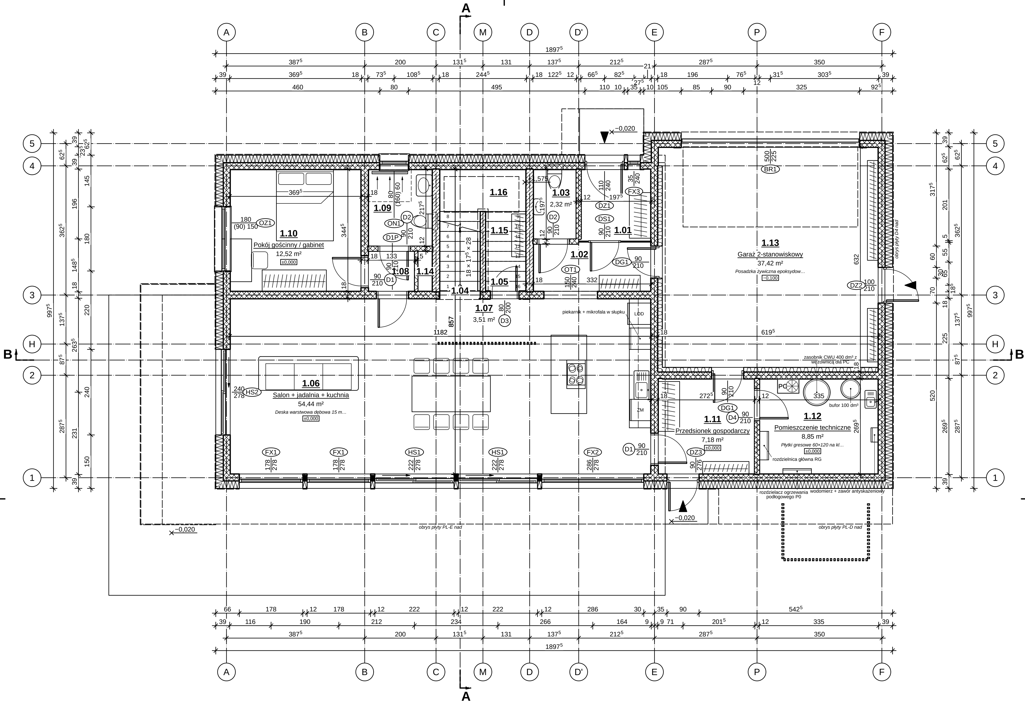
RZUT PARTERU 1:50
