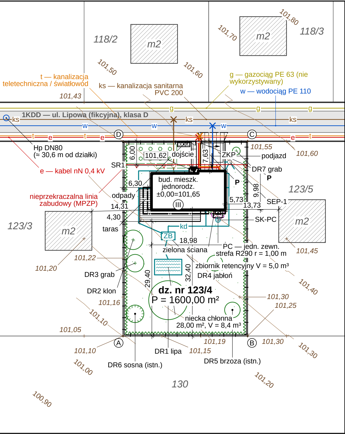
PLAN ZAGOSPODAROWANIA DZIAŁKI 1:500
