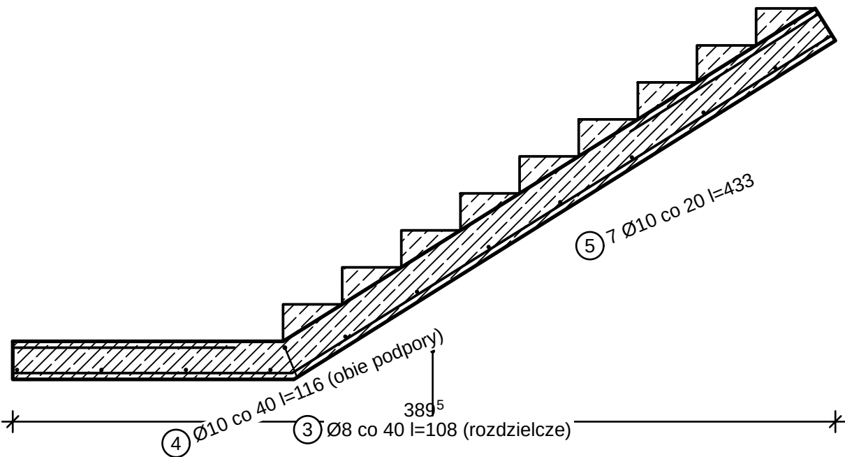
ZBROJENIE SCHODÓW 1:25
