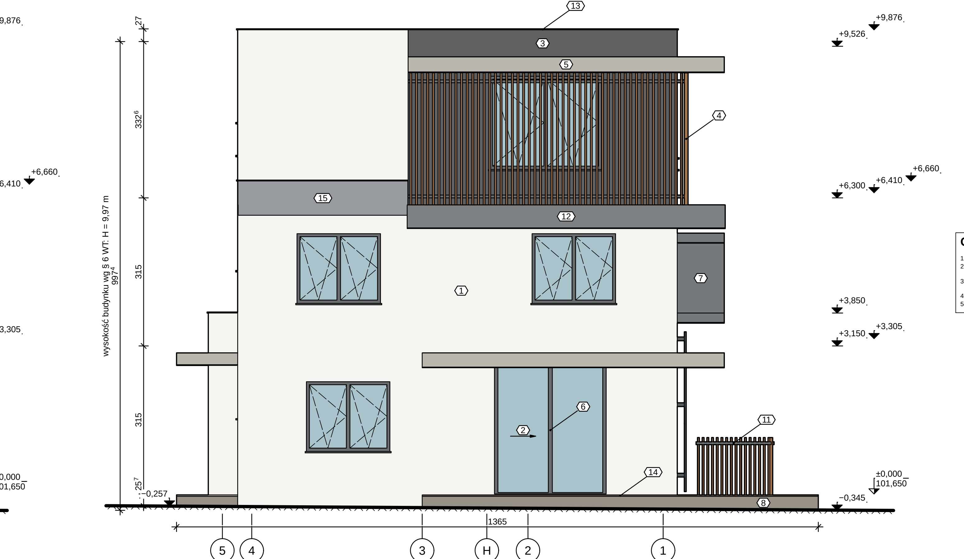
ELEWACJA ZACHODNIA 1:50
