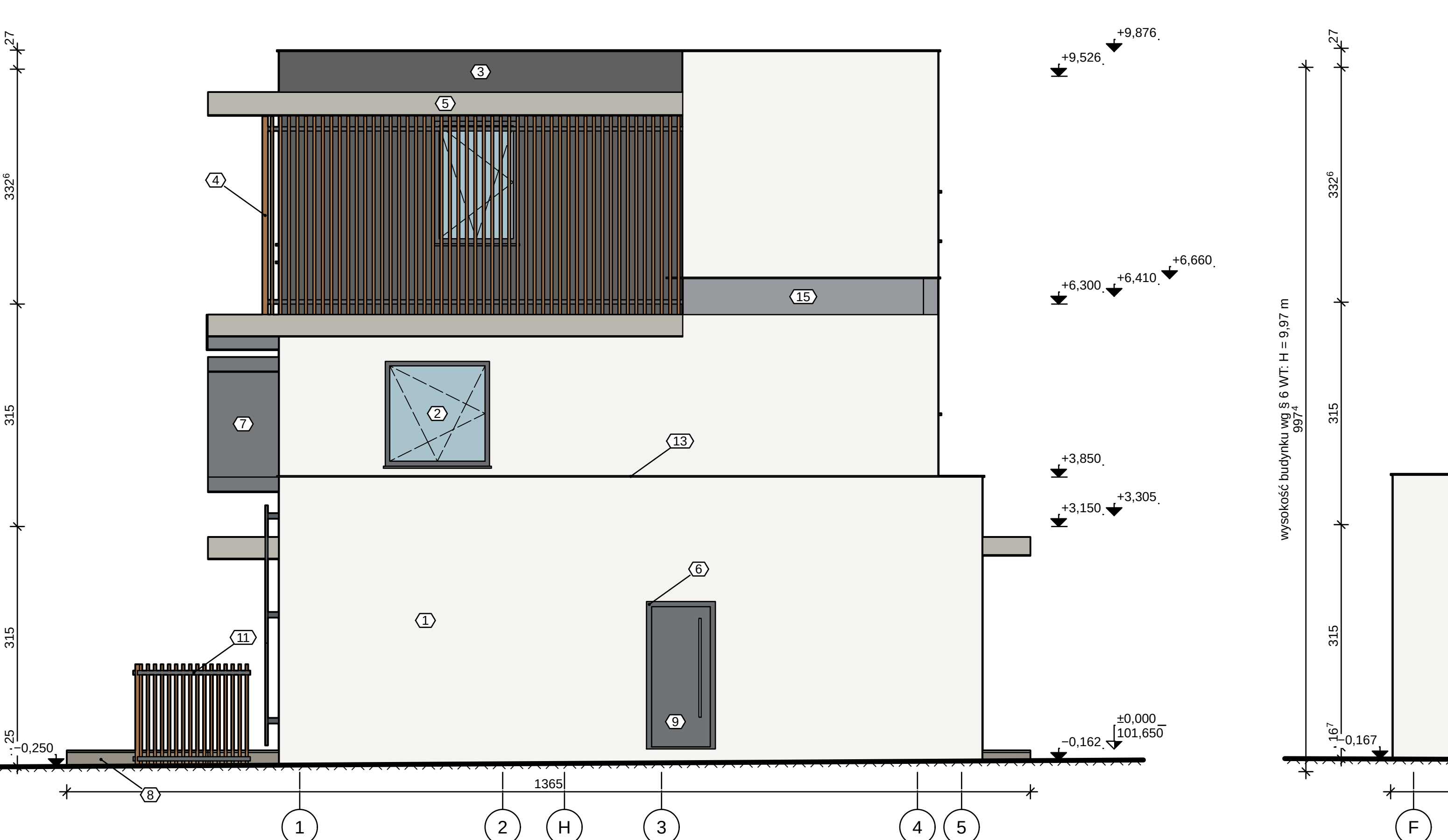
ELEVACJA WSCHODNIA 1:50
