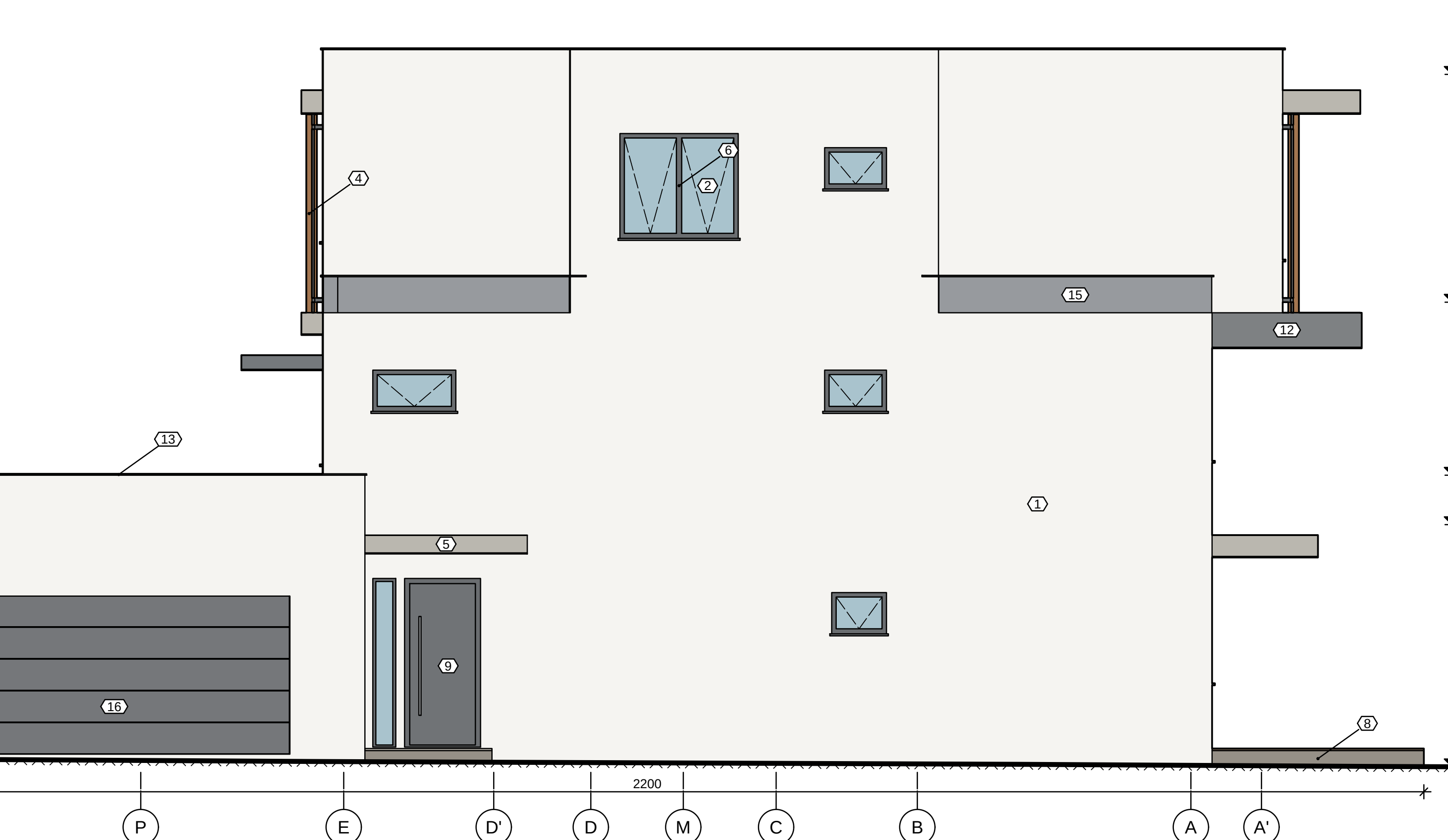
ELEVACJA PÓŁNOCNA (OD ULICY) 1:50
