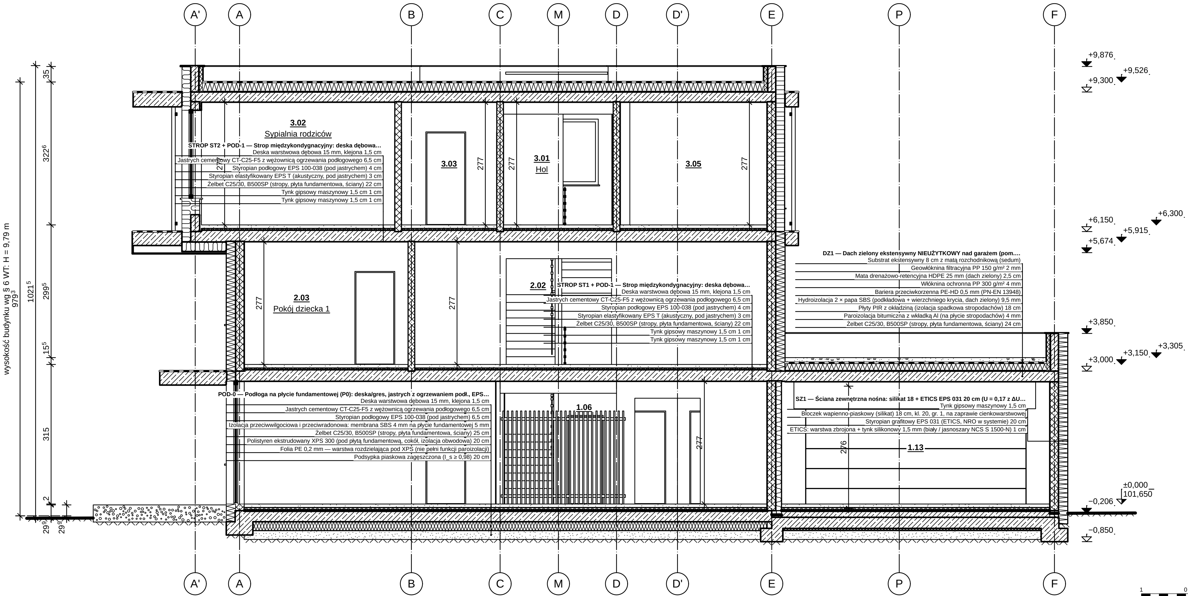
PRZEKRÓJ B-B 1:50
