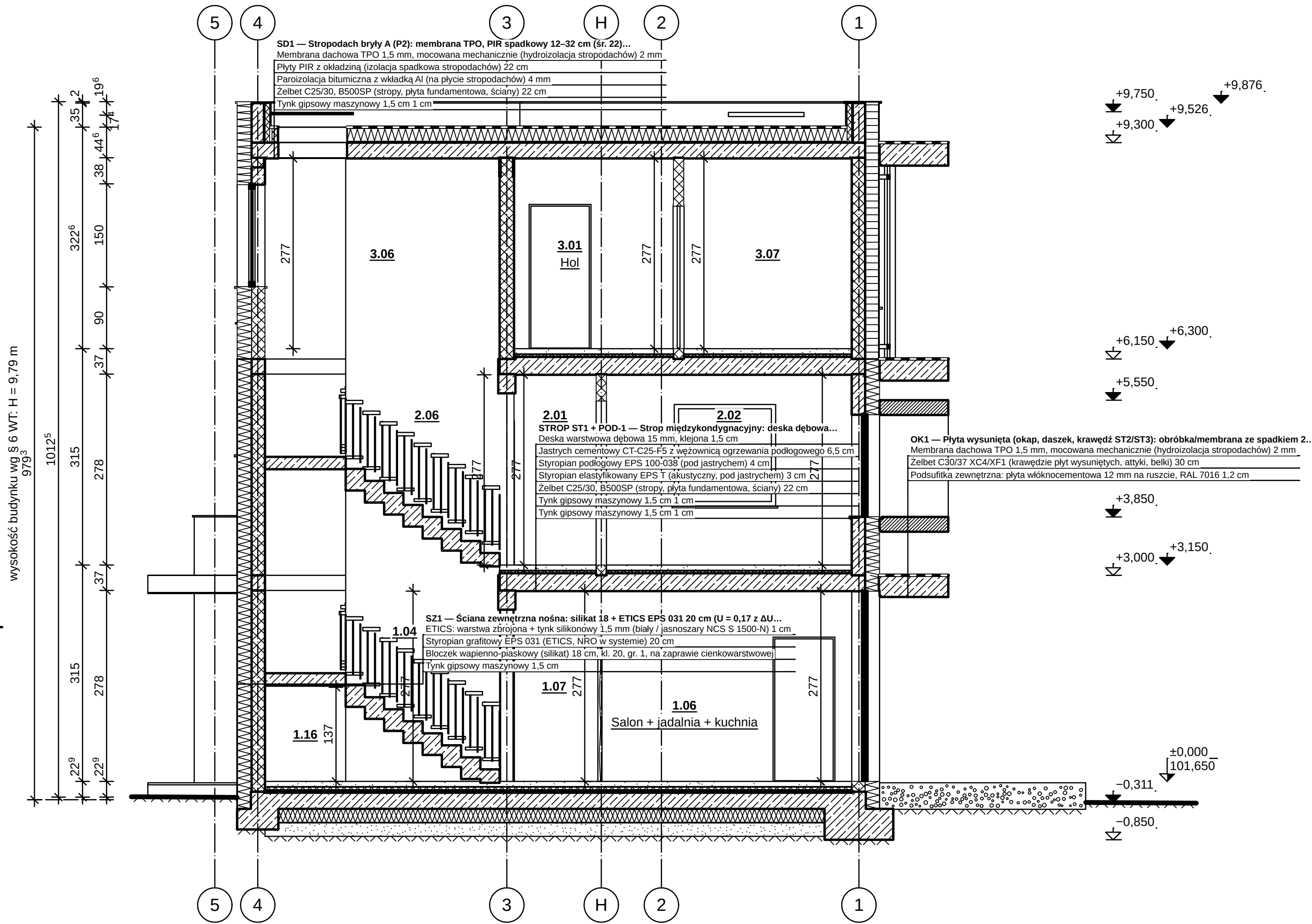
PRZEKRÓJ A-A 1:50
