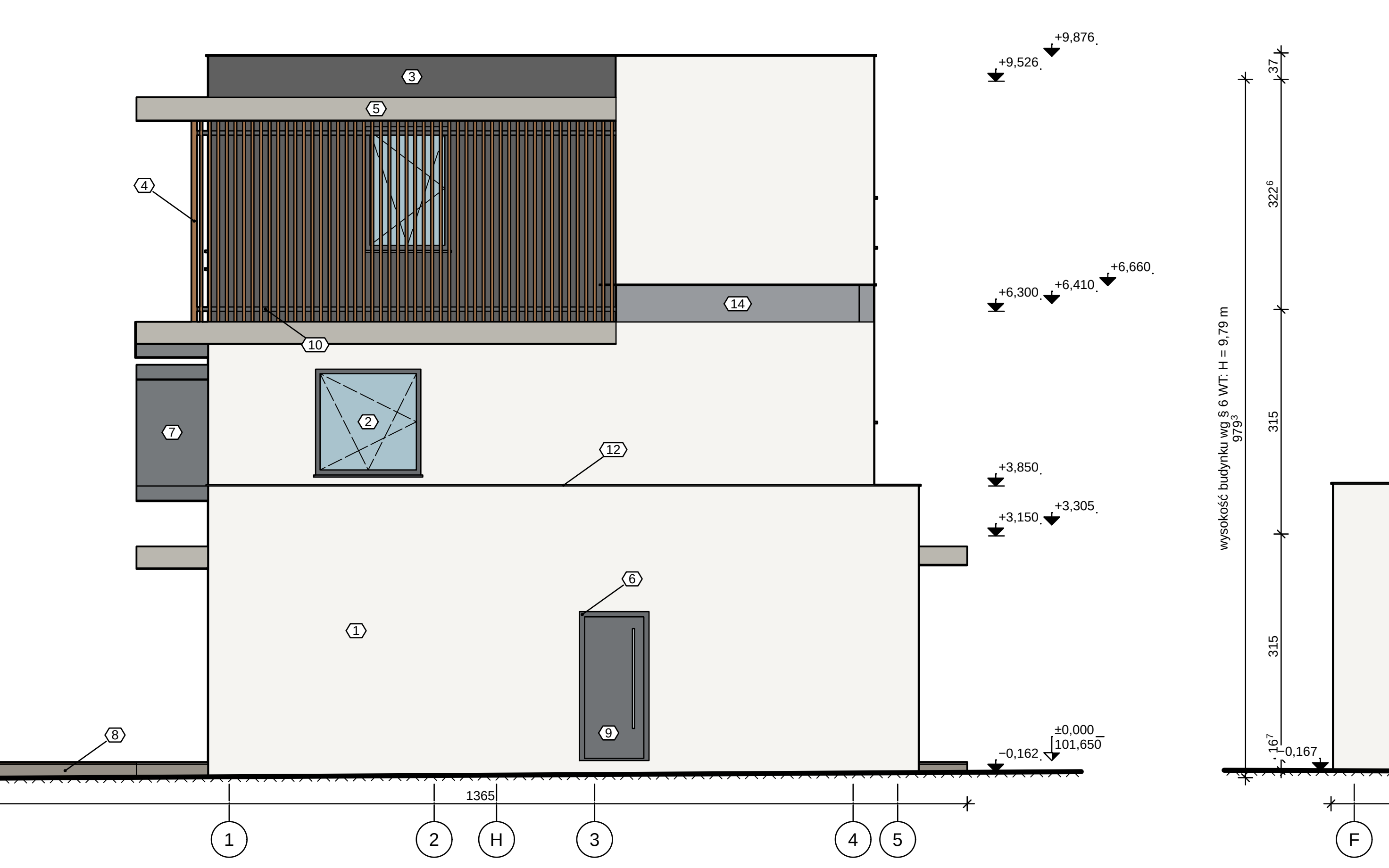
ELEWACJA WSCHODNIA 1:50
