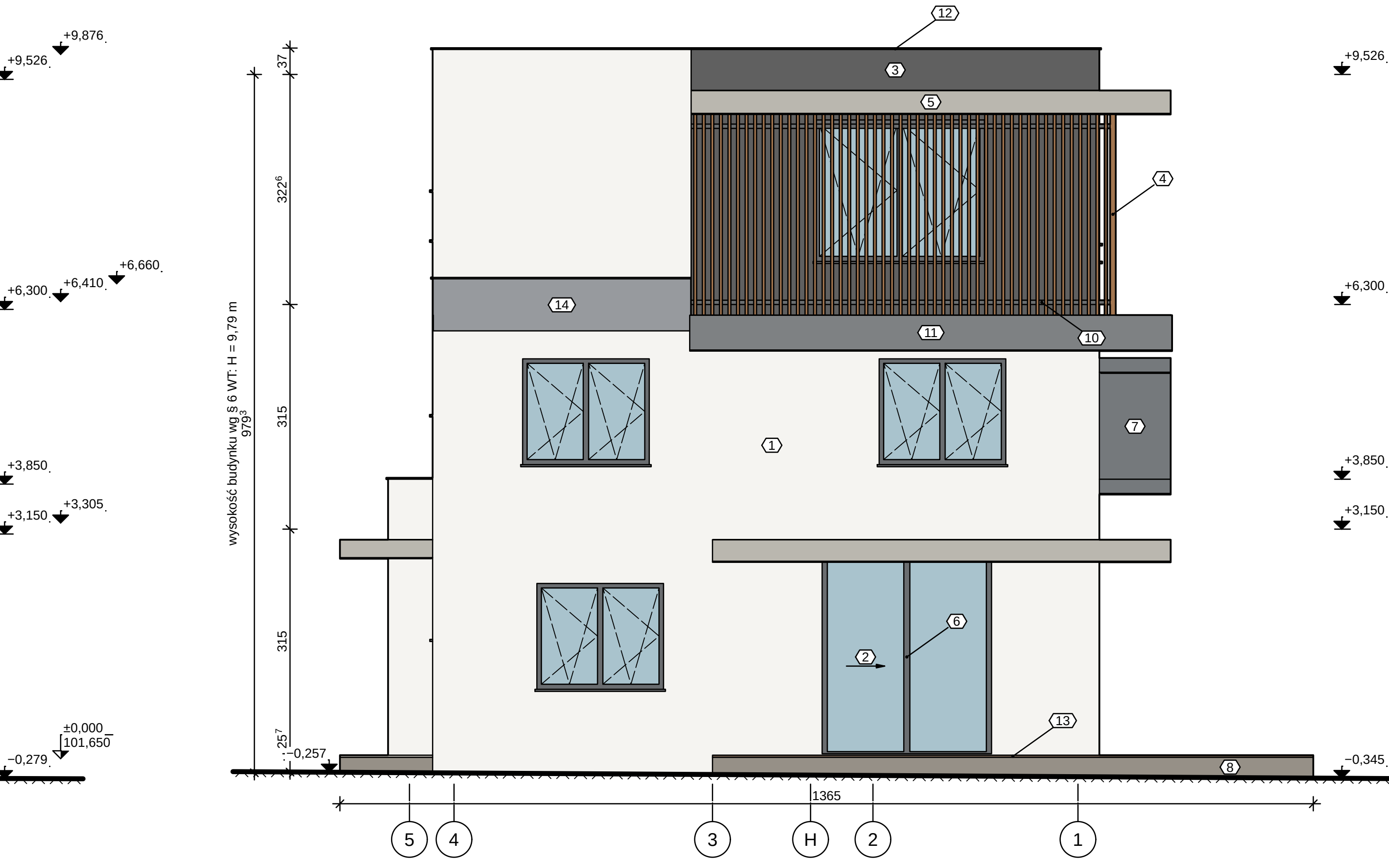
ELEWACJA ZACHODNIA 1:50
