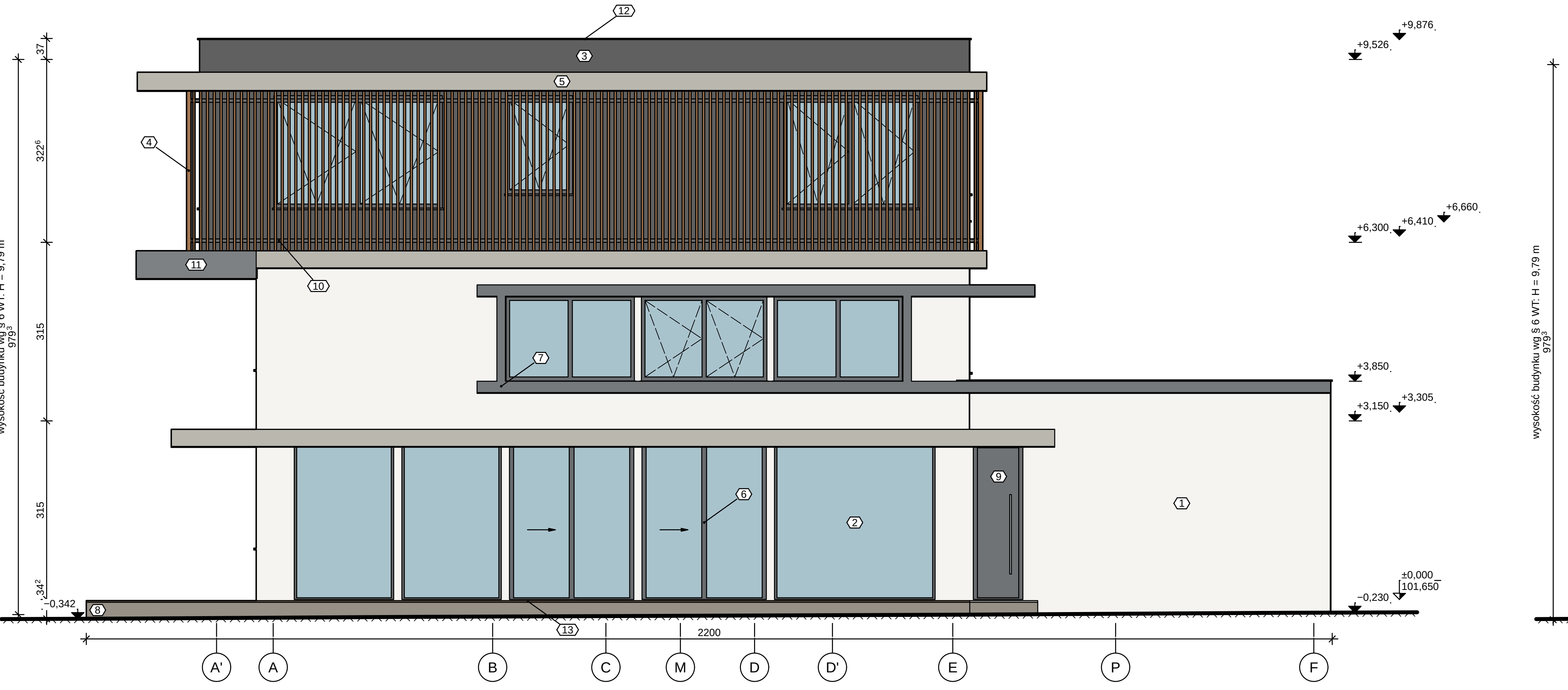
ELEWACJA POŁUDNIOWA (OGRODOWA) 1:50
