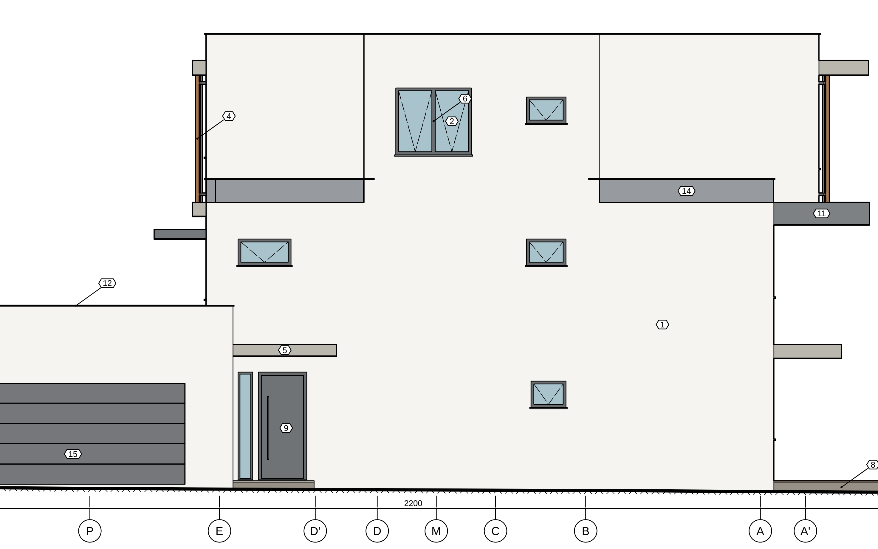
ELEWACJA PÓŁNOCNA (OD ULICY) 1:50
