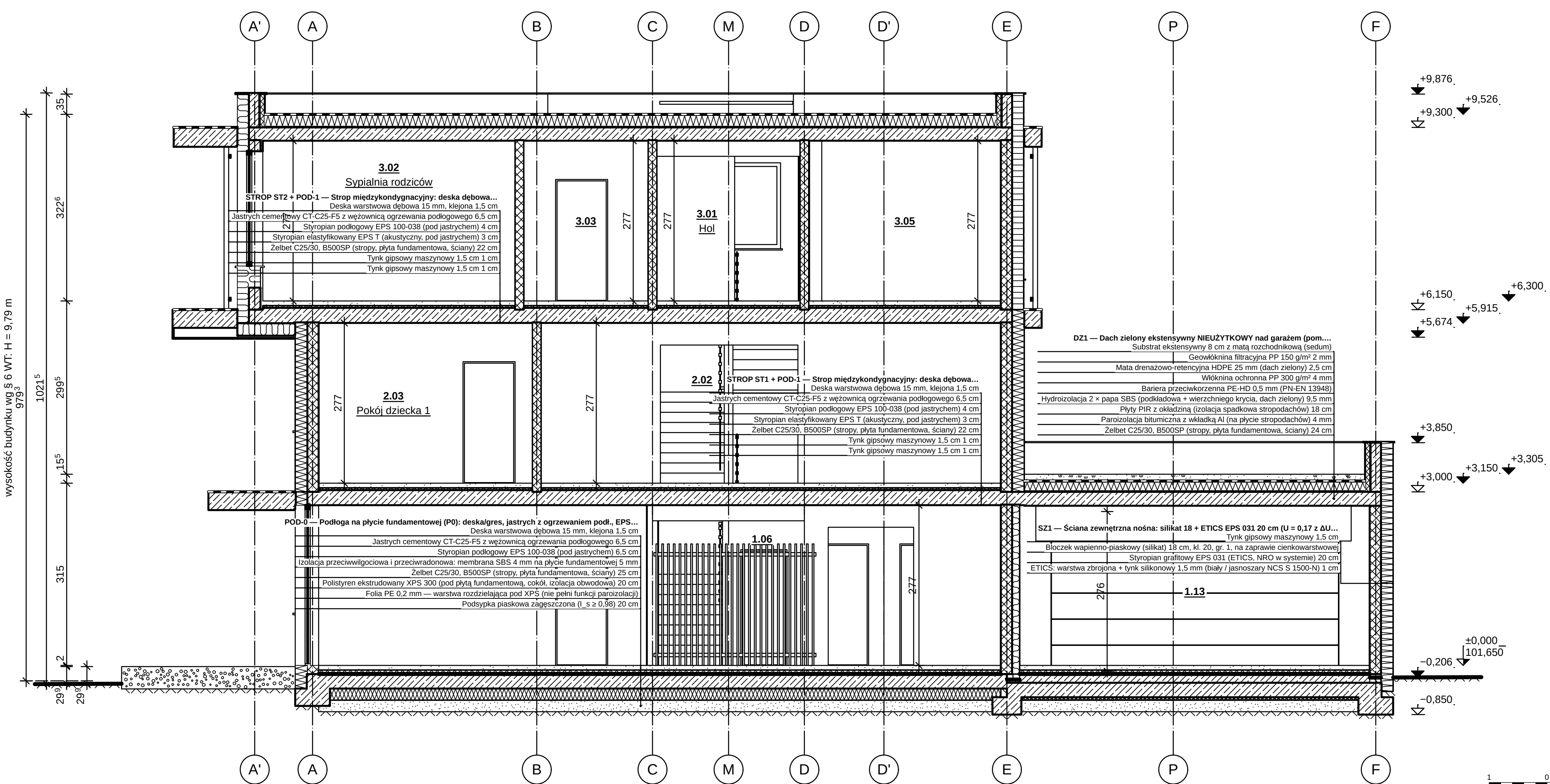
PRZEKRÓJ B-B 1:50
