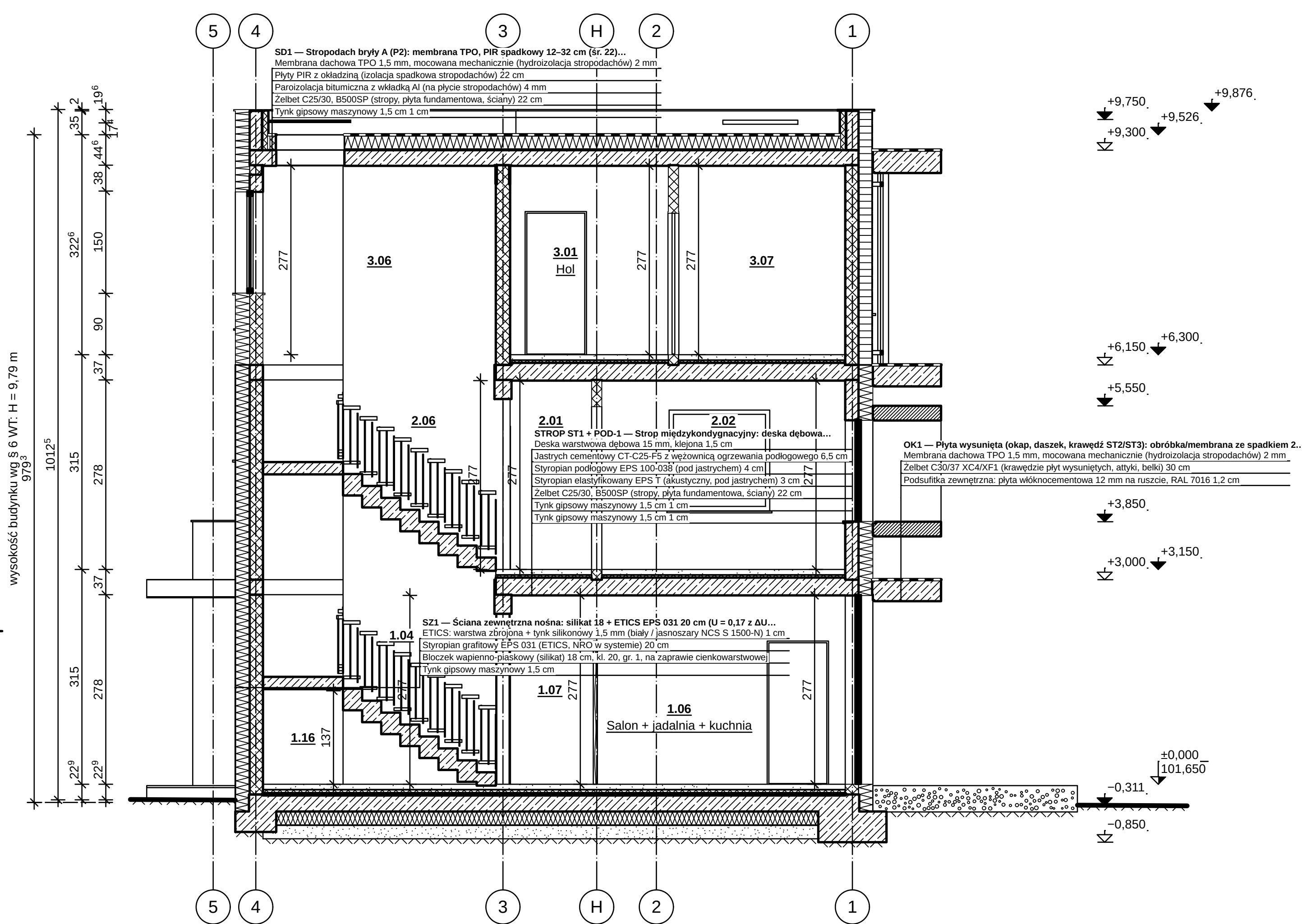
PRZEKRÓJ A-A 1:50
