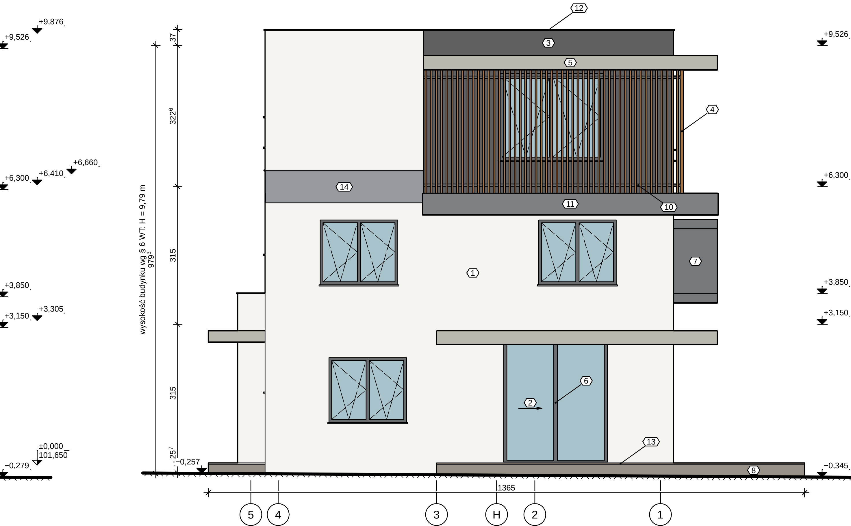
ELEWACJA ZACHODNIA 1:50
