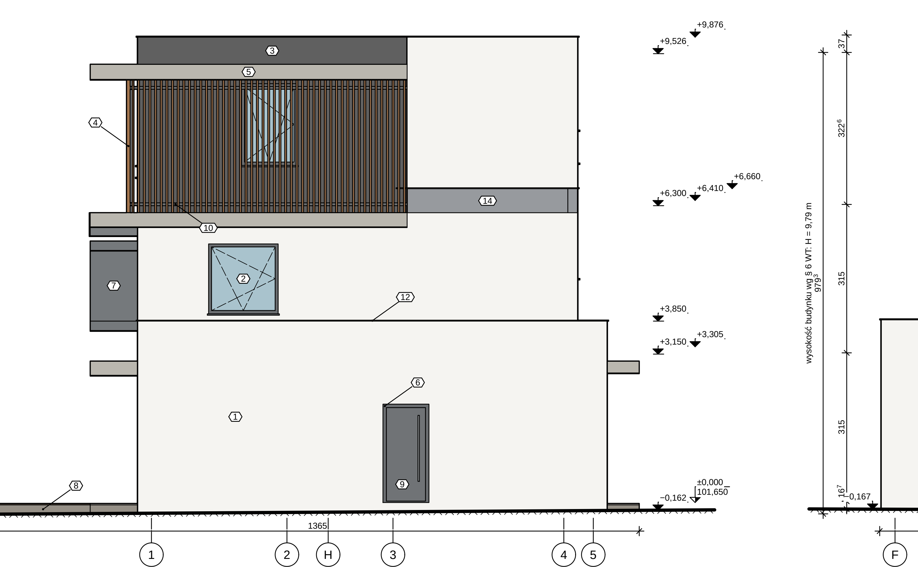
ELEWACJA WSCHODNIA 1:50
