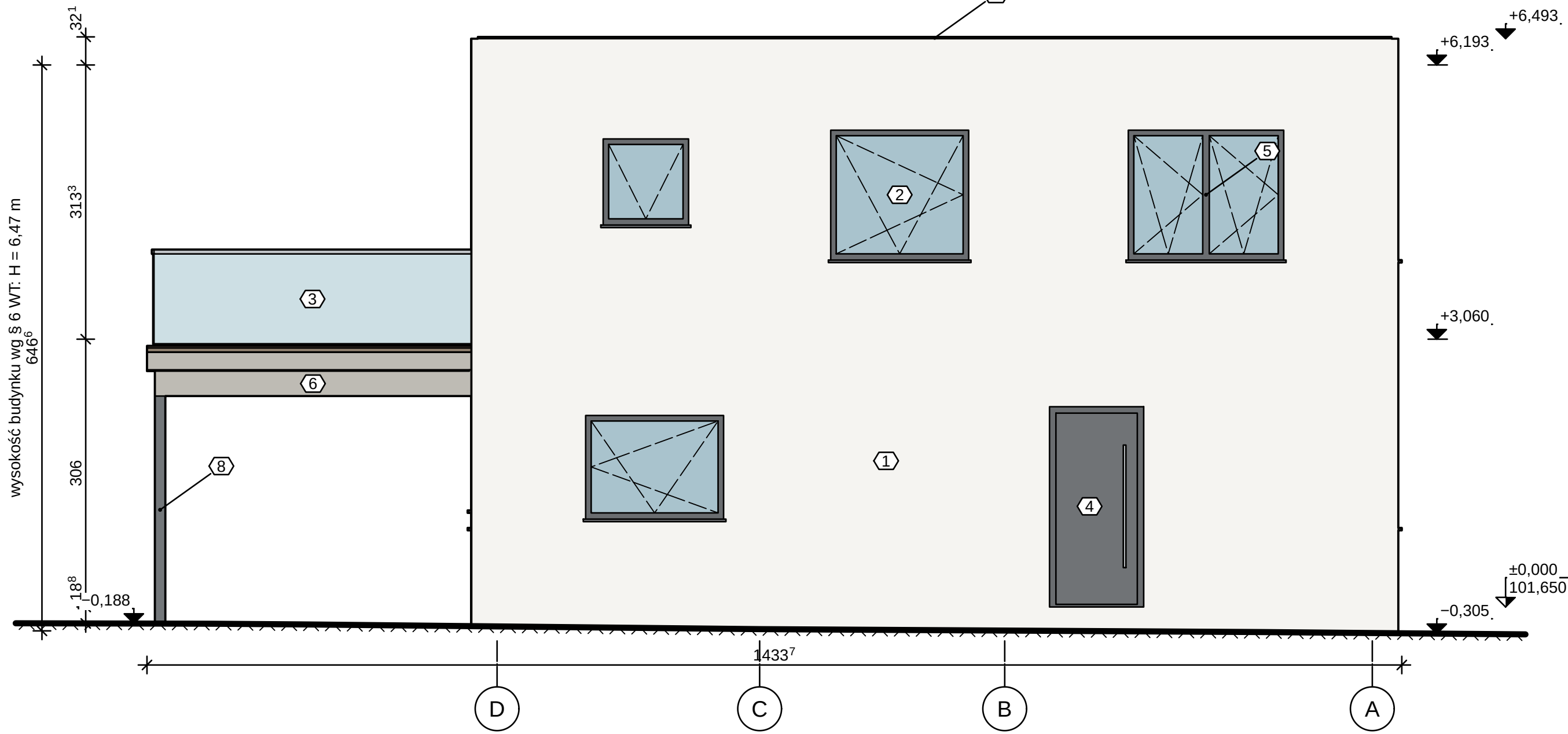
ELEWACJA PÓŁNOCNA 1:50
