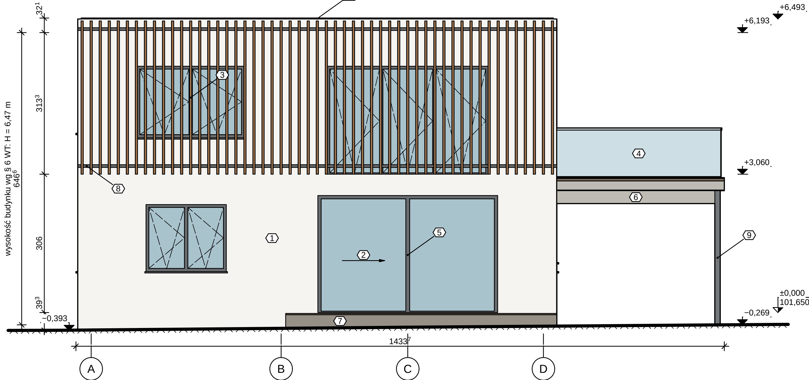
ELEWACJA POŁUDNIOWA 1:50
