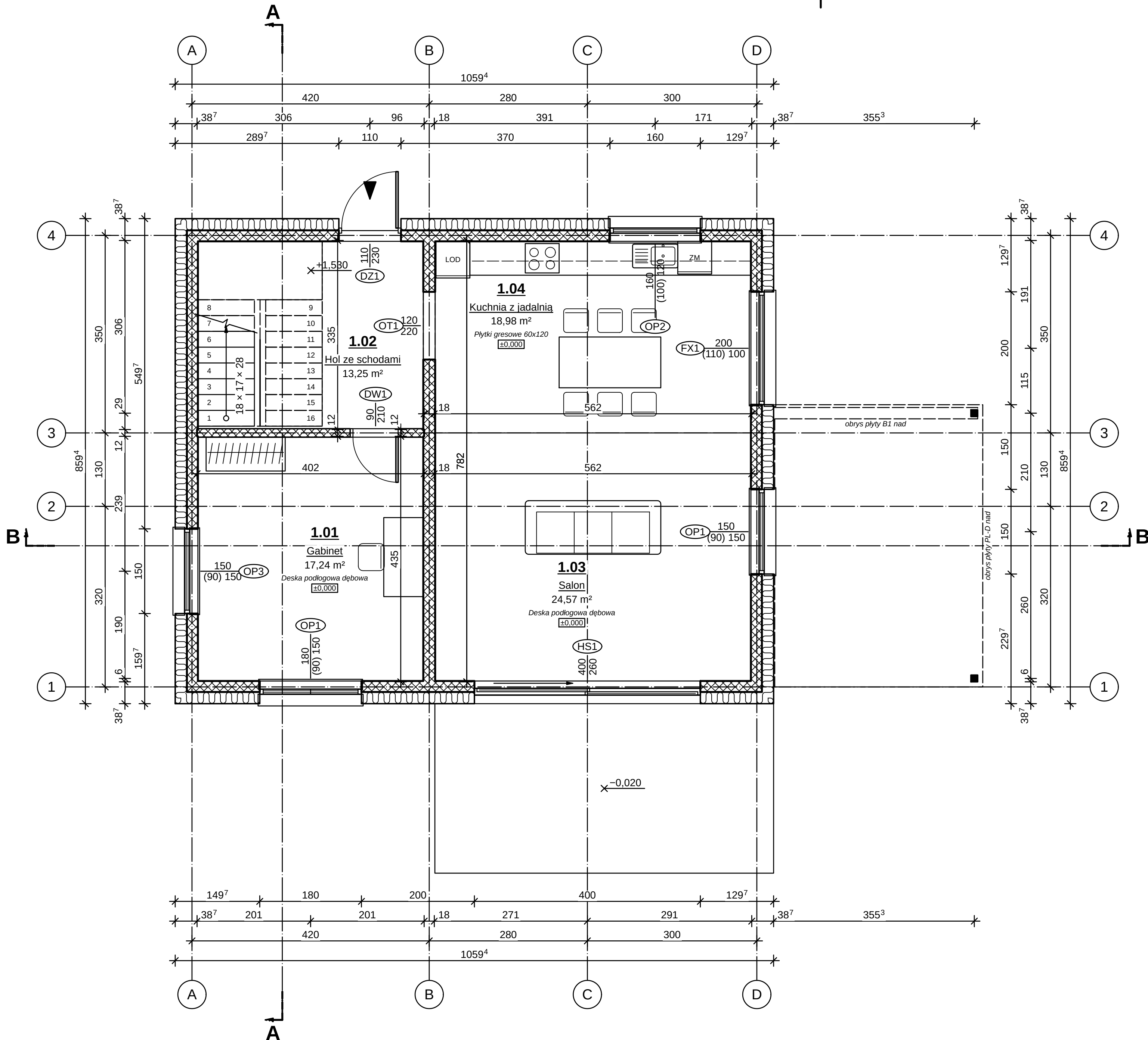
RZUT PARTERU 1:50
