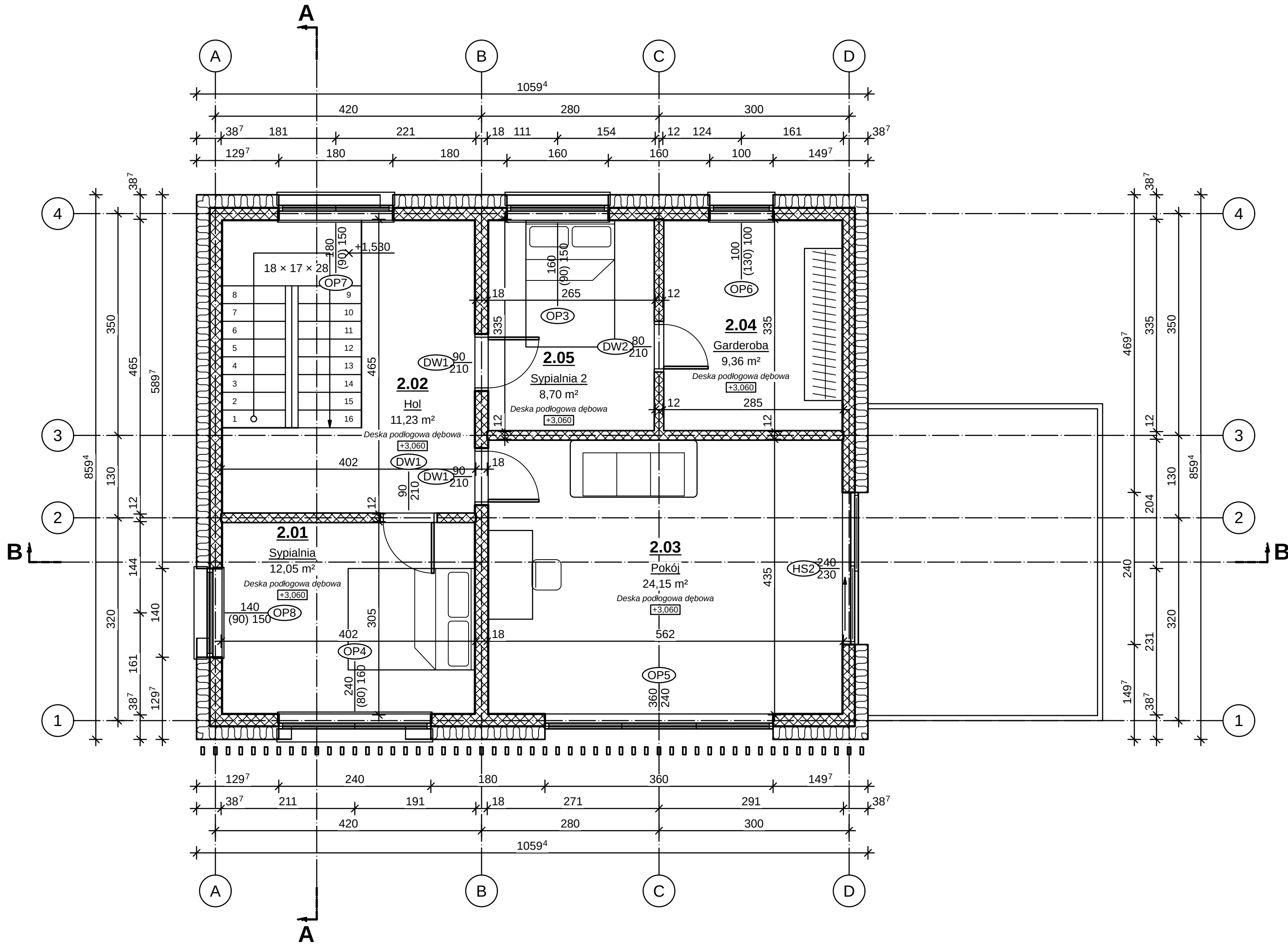
RZUT PIĘTRA 1:50
