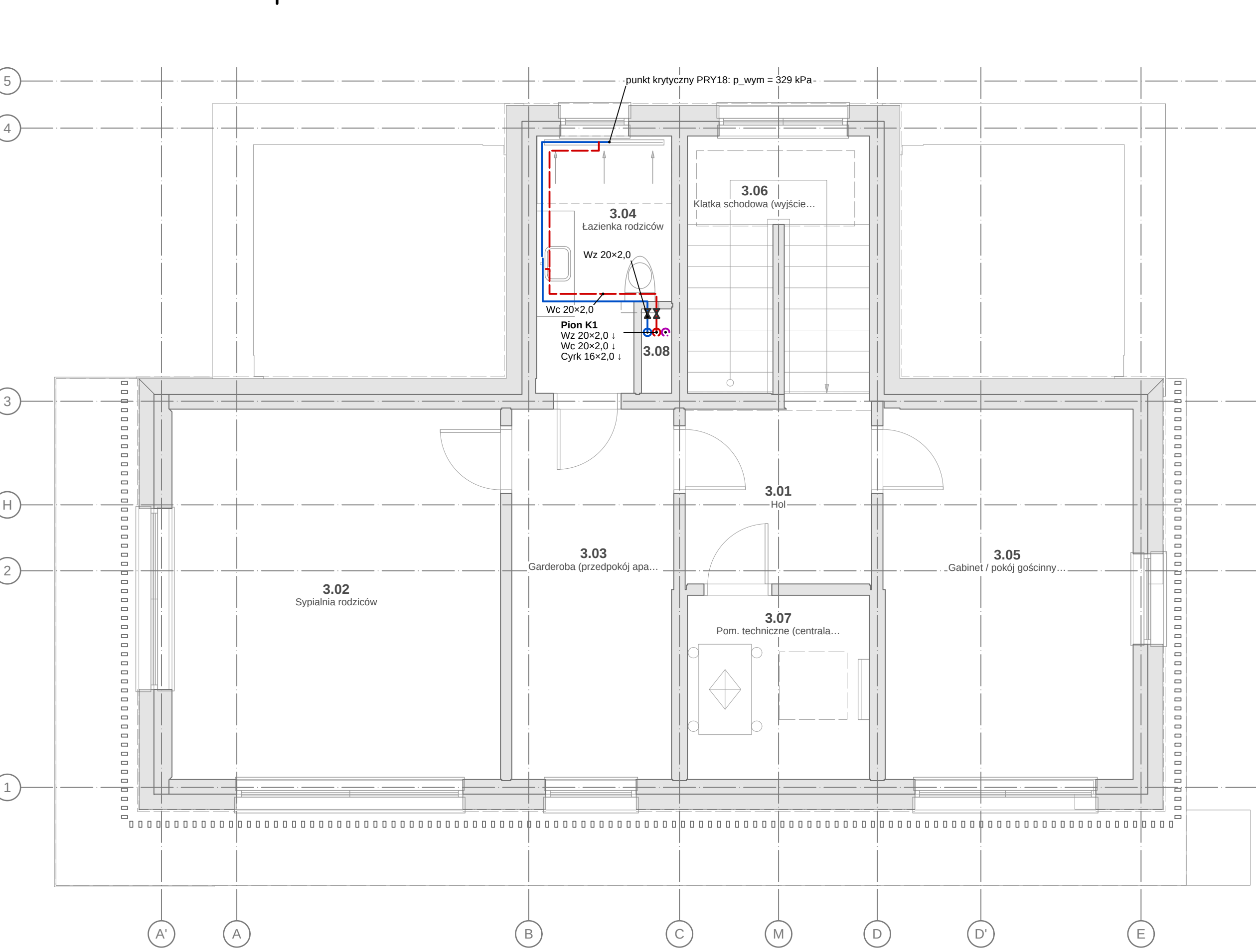
INSTALACJA WODOCIĄGOWA — RZUT II PIĘTRA 1:50
