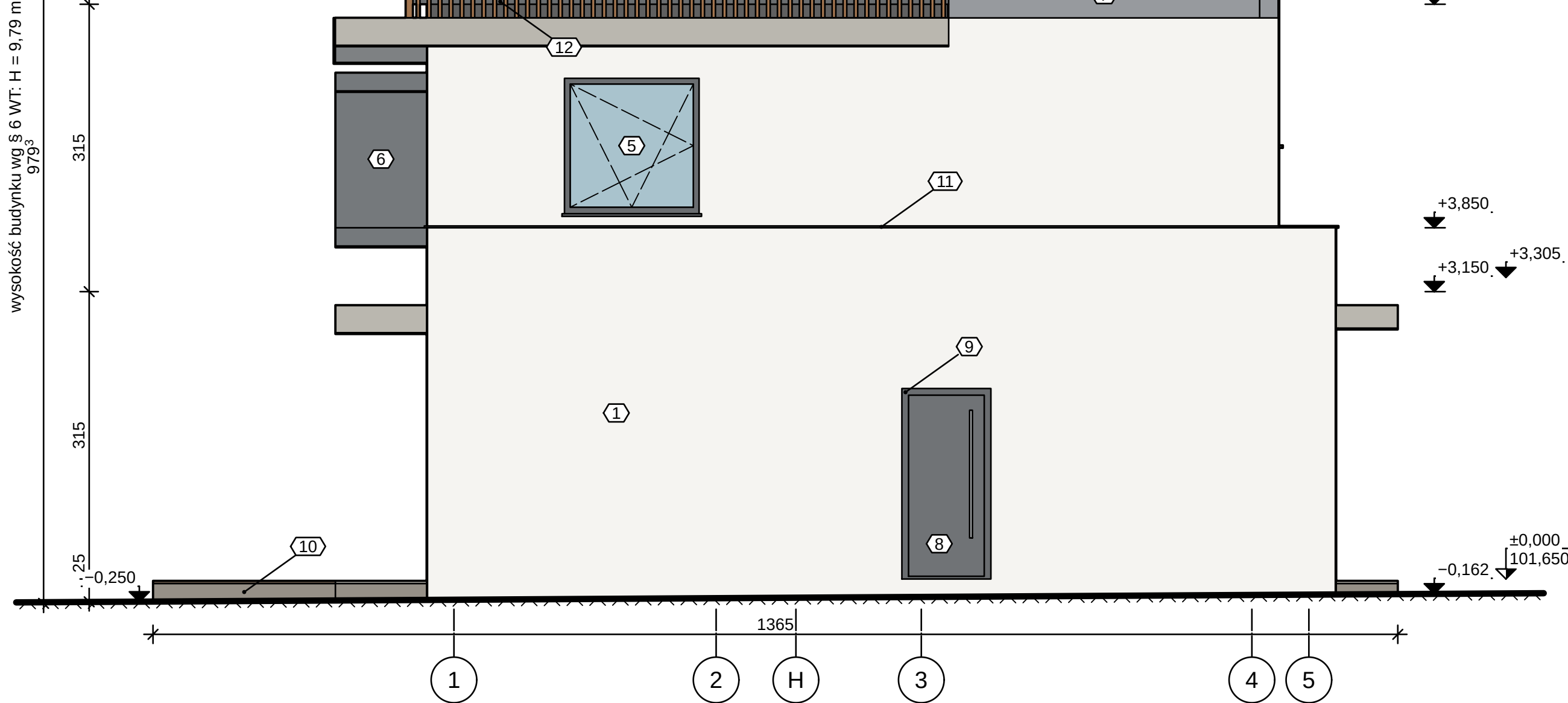
ELEWACJA WSCHODNIA 1:50
