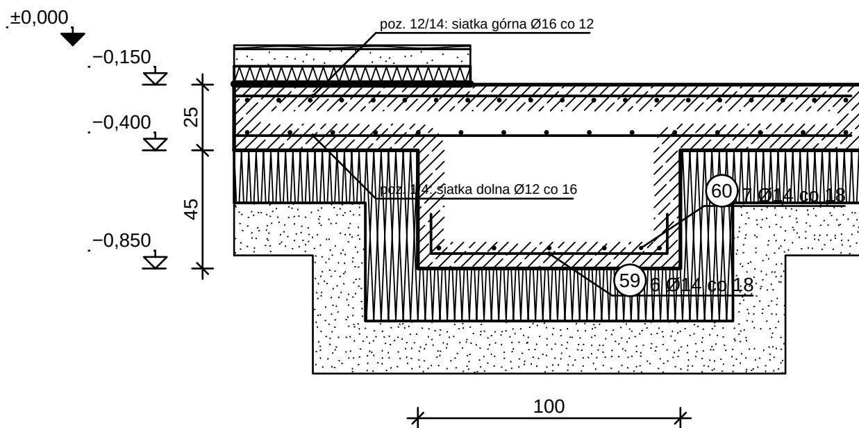
PRZEKRÓJ 3-3 — POGRUBIENIE SF1 1:20
