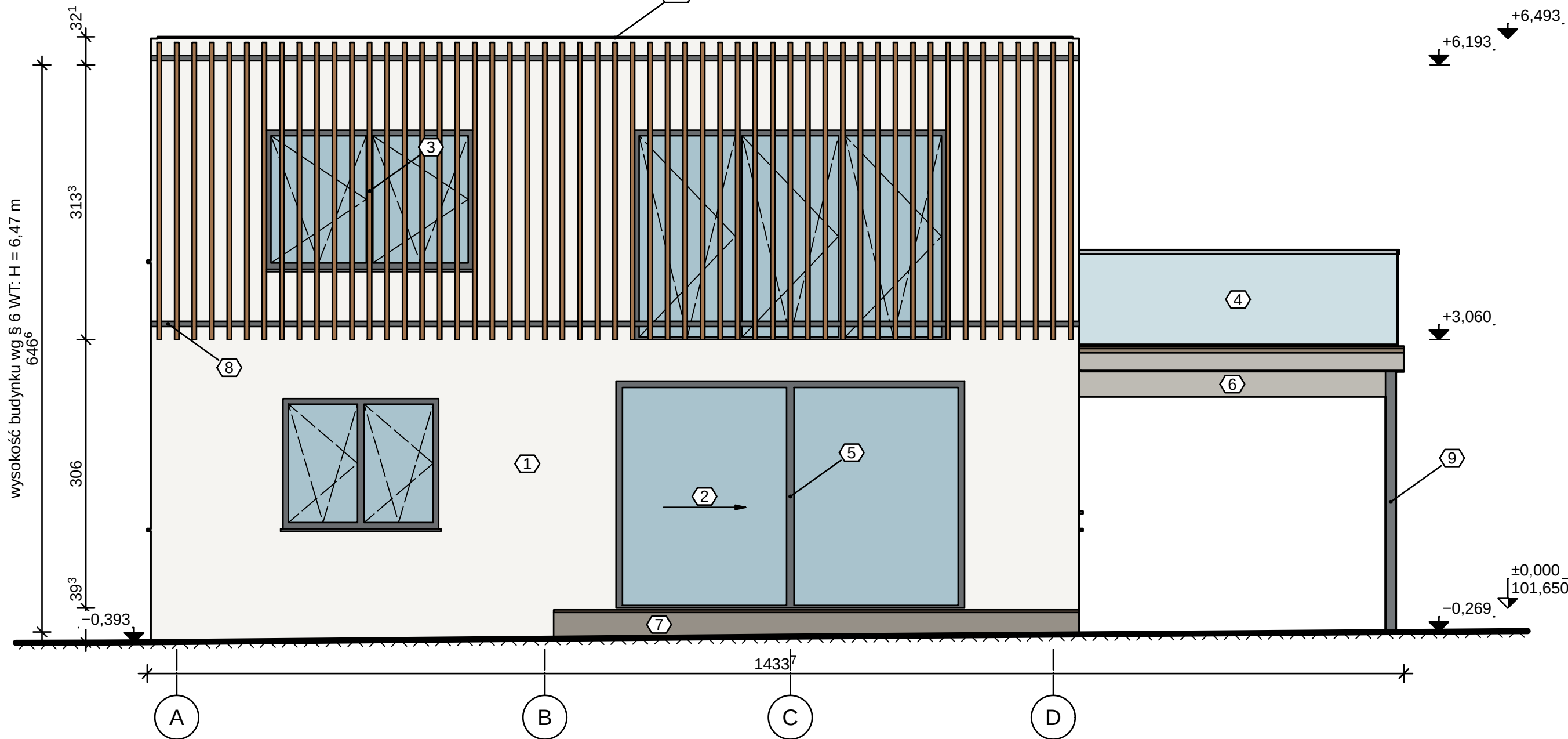
ELEWACJA POŁUDNIOWA 1:50
