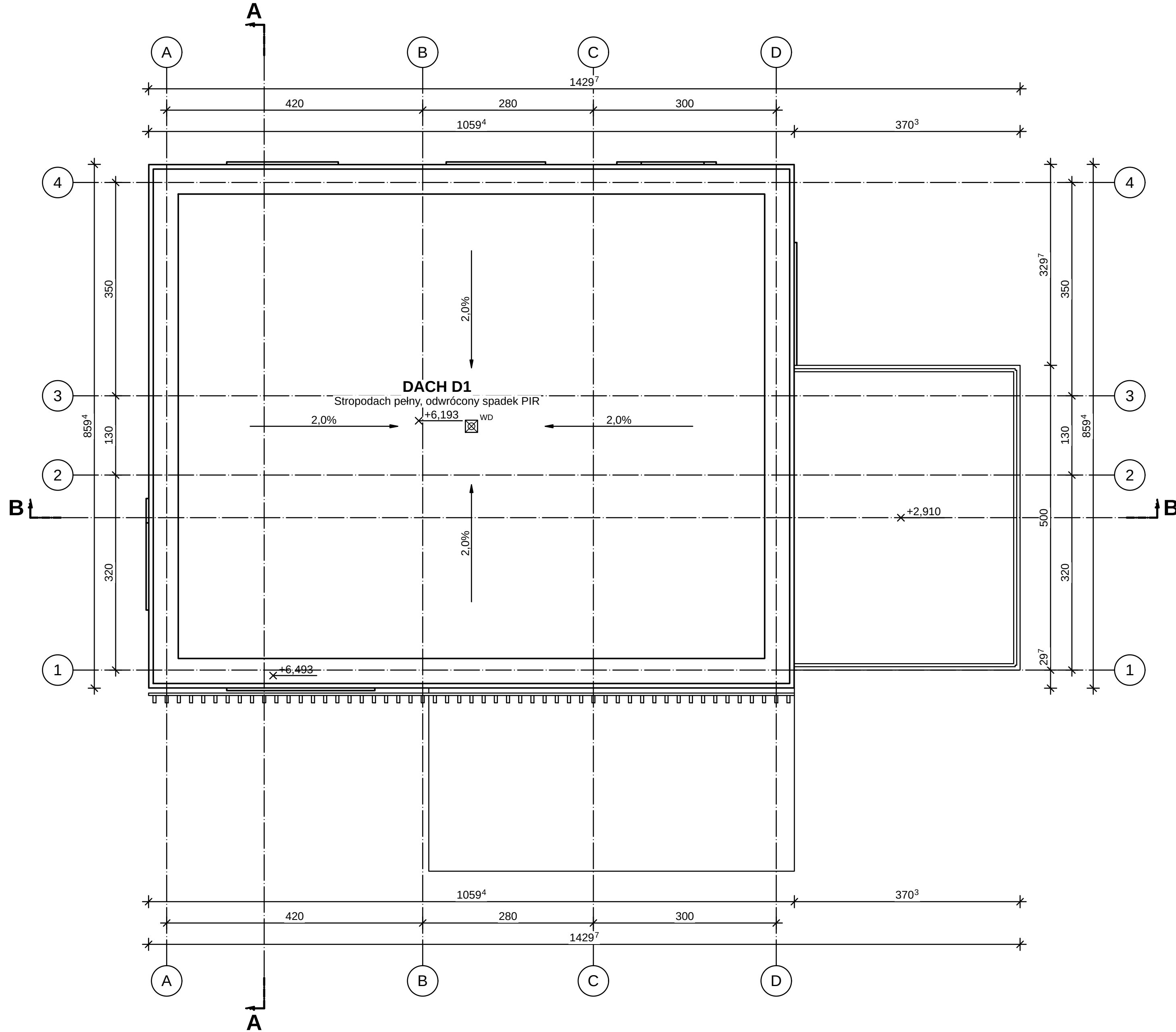
RZUT DACHU 1:50
