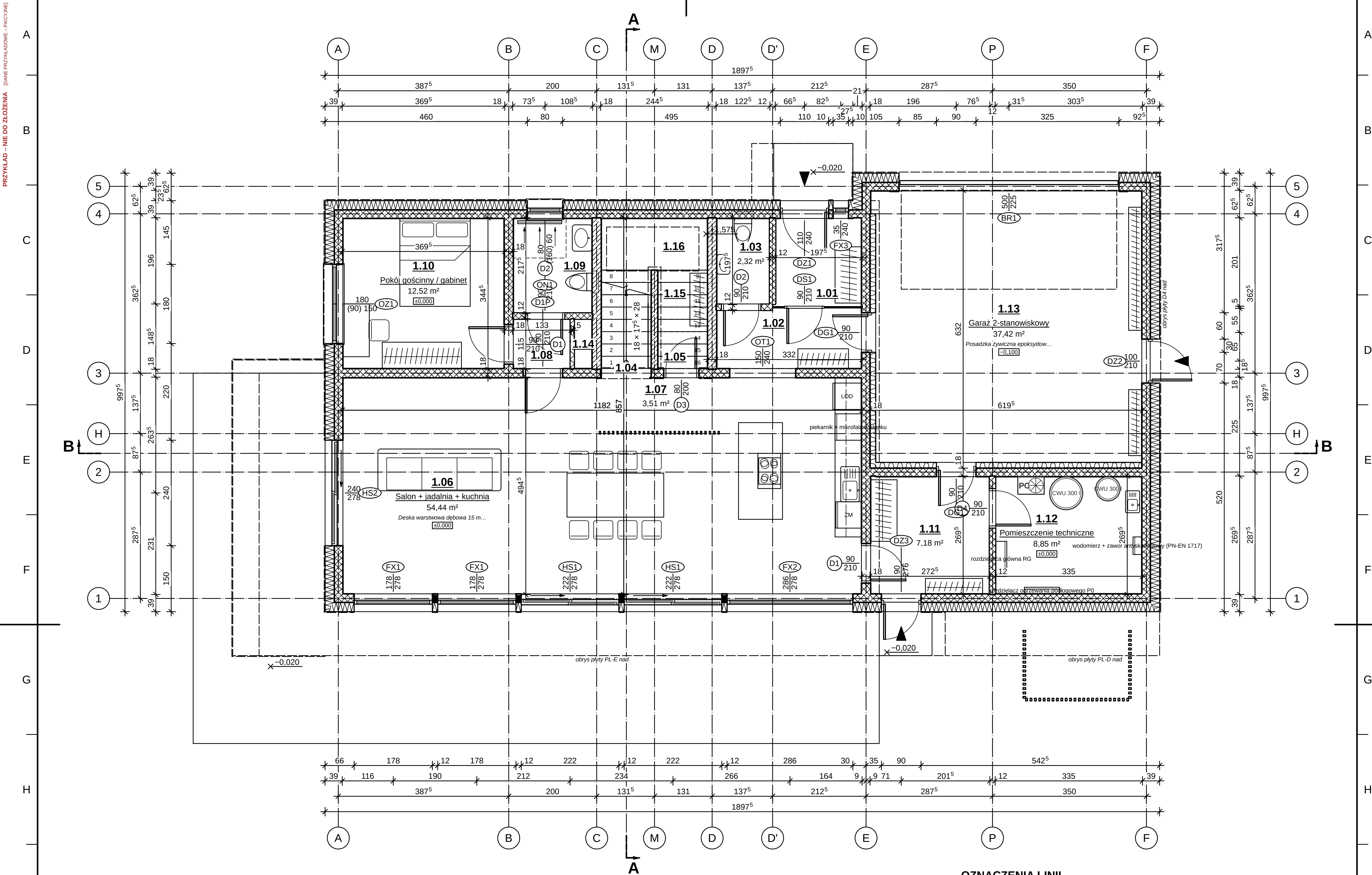
RZUT PARTERU 1:50
