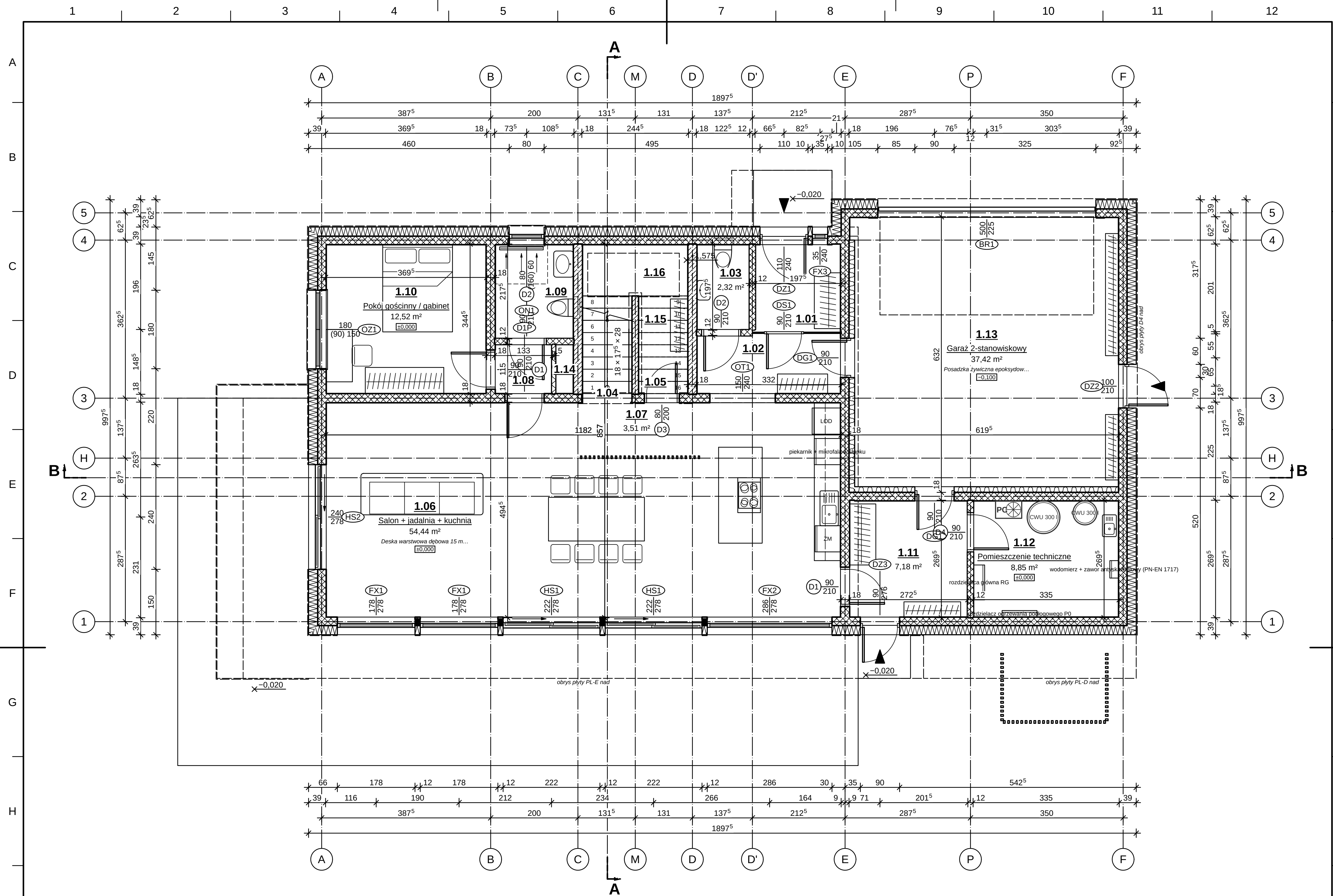
RZUT PARTERU 1:50
