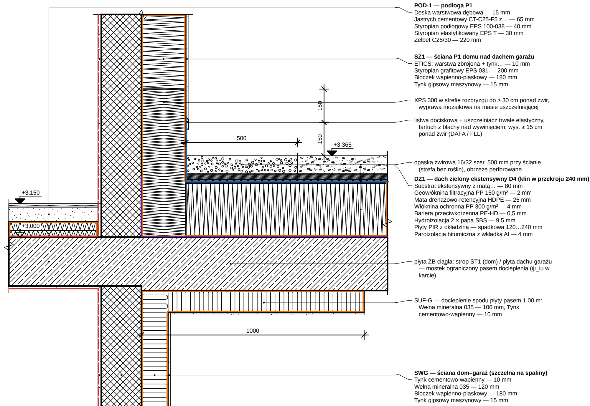
DETAL D-10 — ŚCIANA DOM-GARAŻ (SWG) I DACH ZIELONY D4 PRZY ŚCIANIE DOMU 1:10
