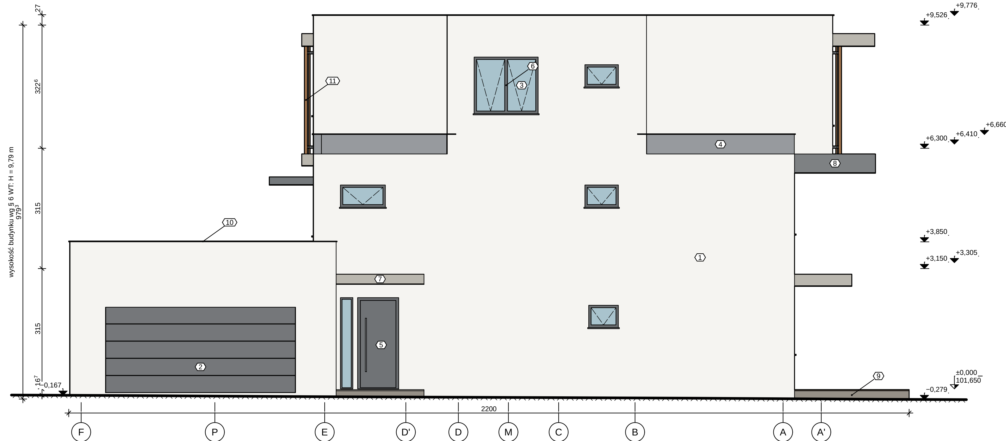
ELEWACJA PÓŁNOCNA 1:50
