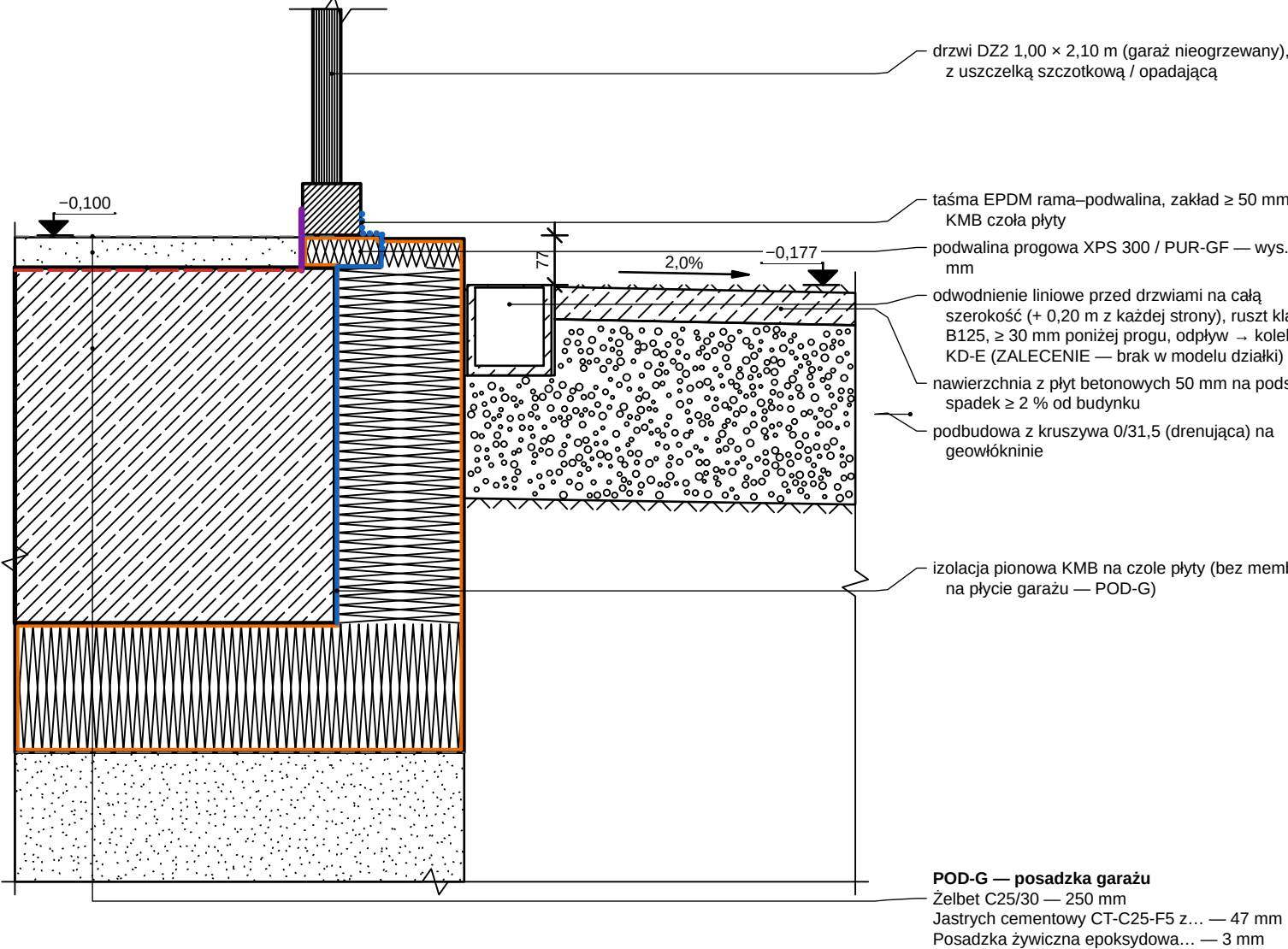
DETAL D-14 — PRÓG DRZWI DZ2 GARAŻU — ODWODNIENIE LINIOWE I USZCZELNIENIE 1:10
