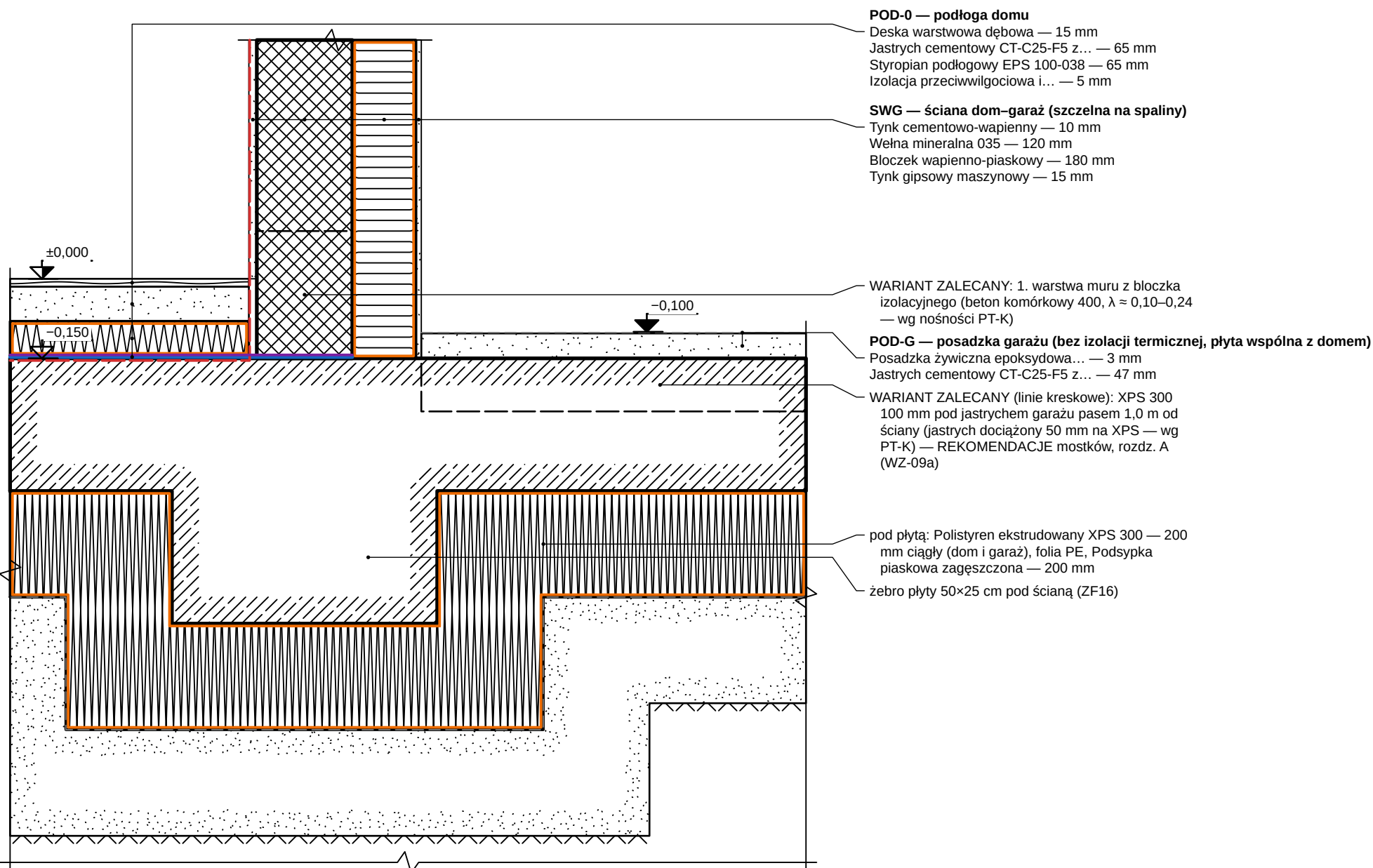
DETAL D-11 — ŚCIANA DOM-GARAŻ (SWG) NA PŁYCE FUNDAMENTOWEJ 1:10
