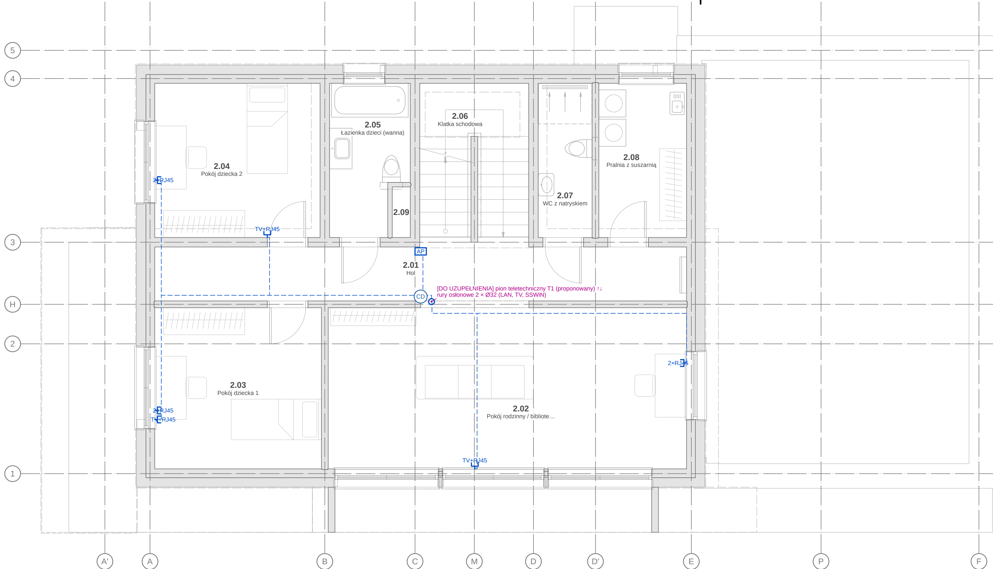
INSTALACJE TELETECHNICZNE — RZUT I PIĘTRA 1:50
