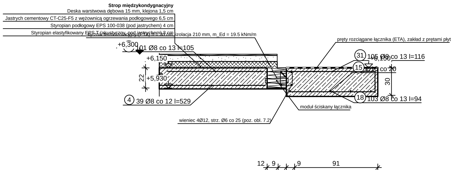
WĘZŁ WSPORNIKA PL-2 — ŁĄCZNIK TERMOIZOLACYJNY 1:20
