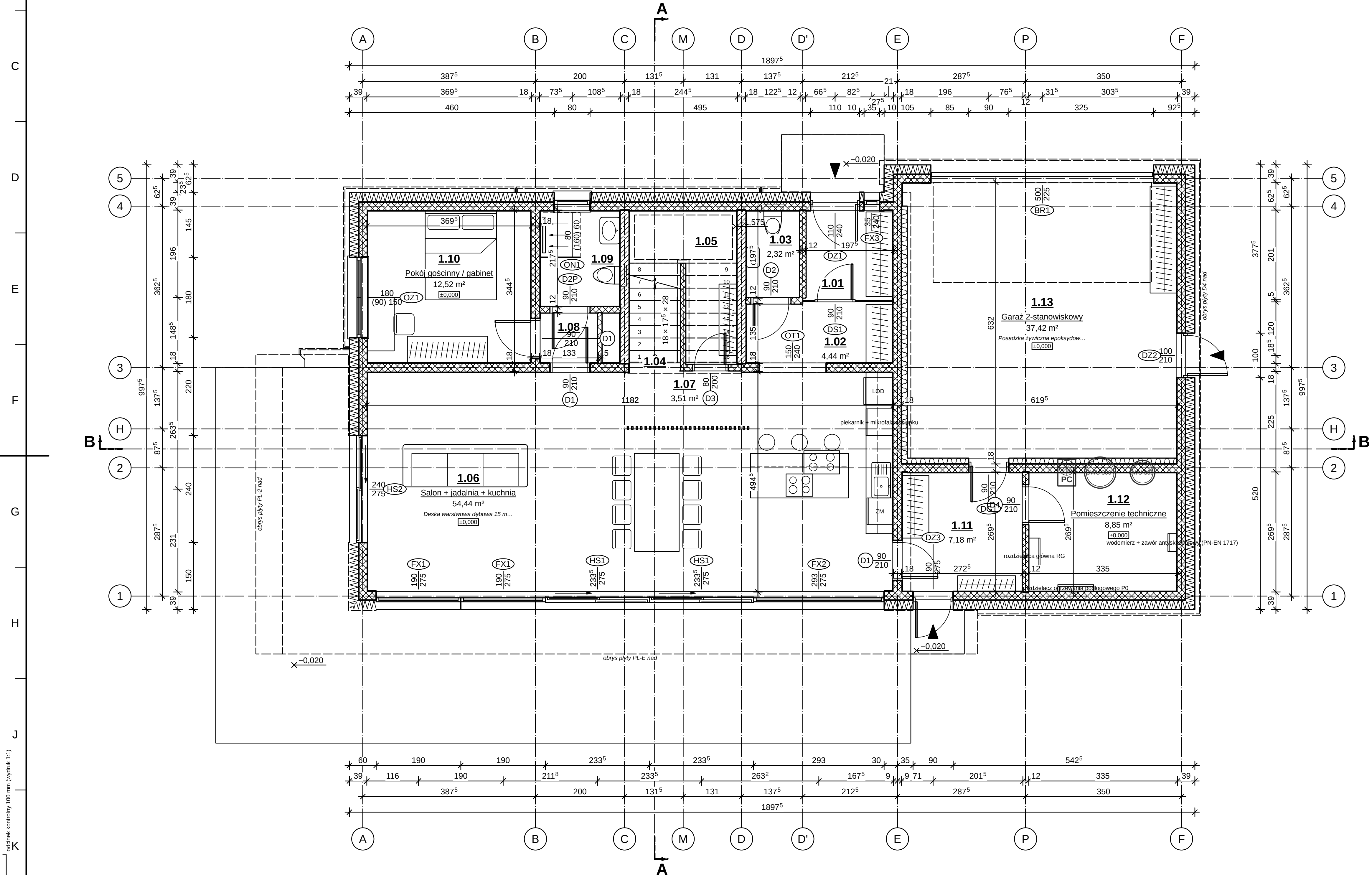
RZUT PARTERU 1:50
