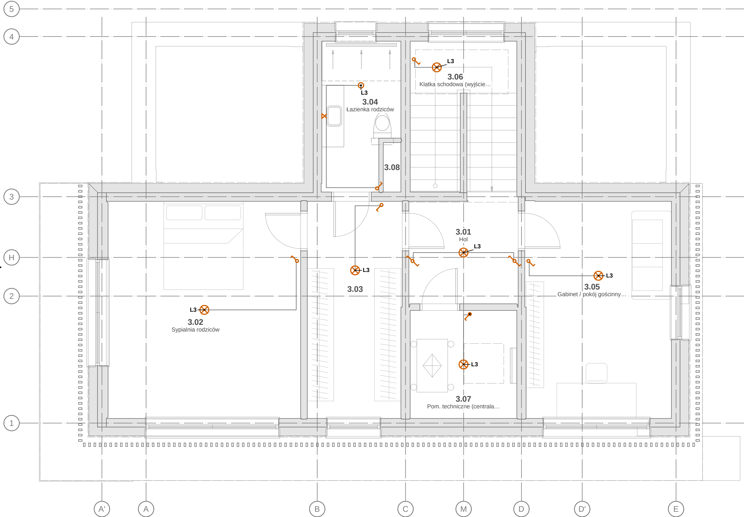
INSTALACJA OŚWIETLLENIA — RZUT II PIĘTRA 1:50
