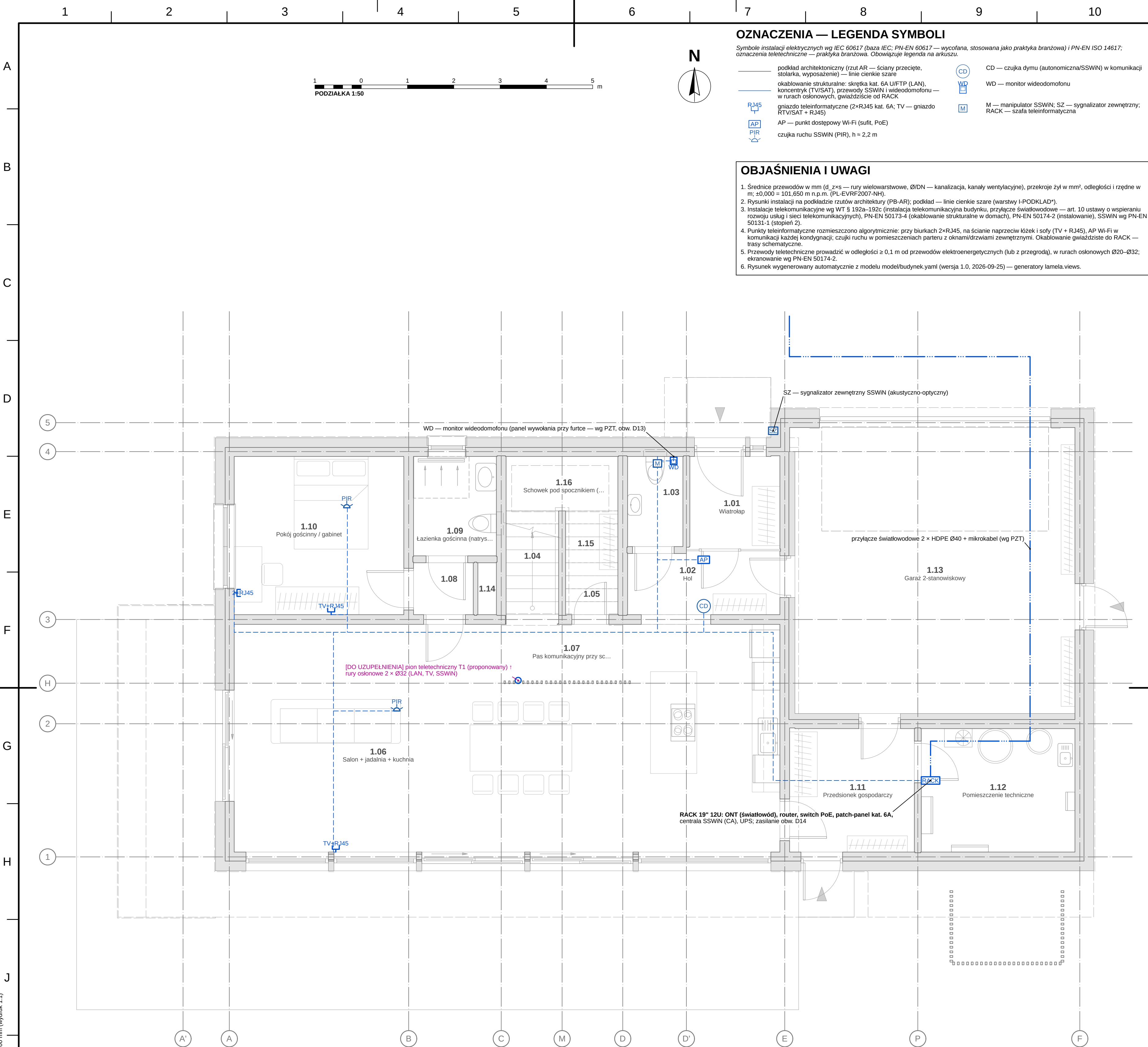
TELETECHNIKA — RZUT PARTERU 1:50
