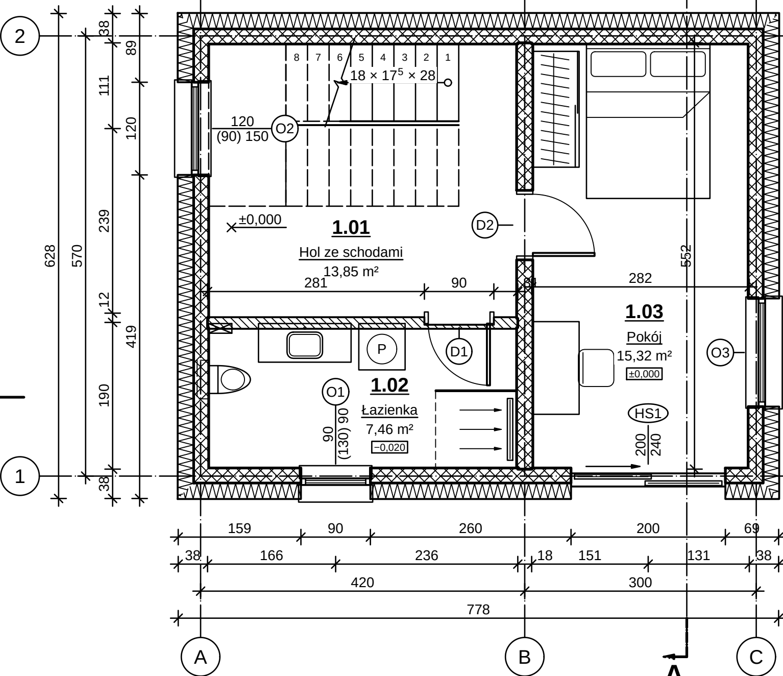
RZUT PARTERU — FRAGMENT 1:50
