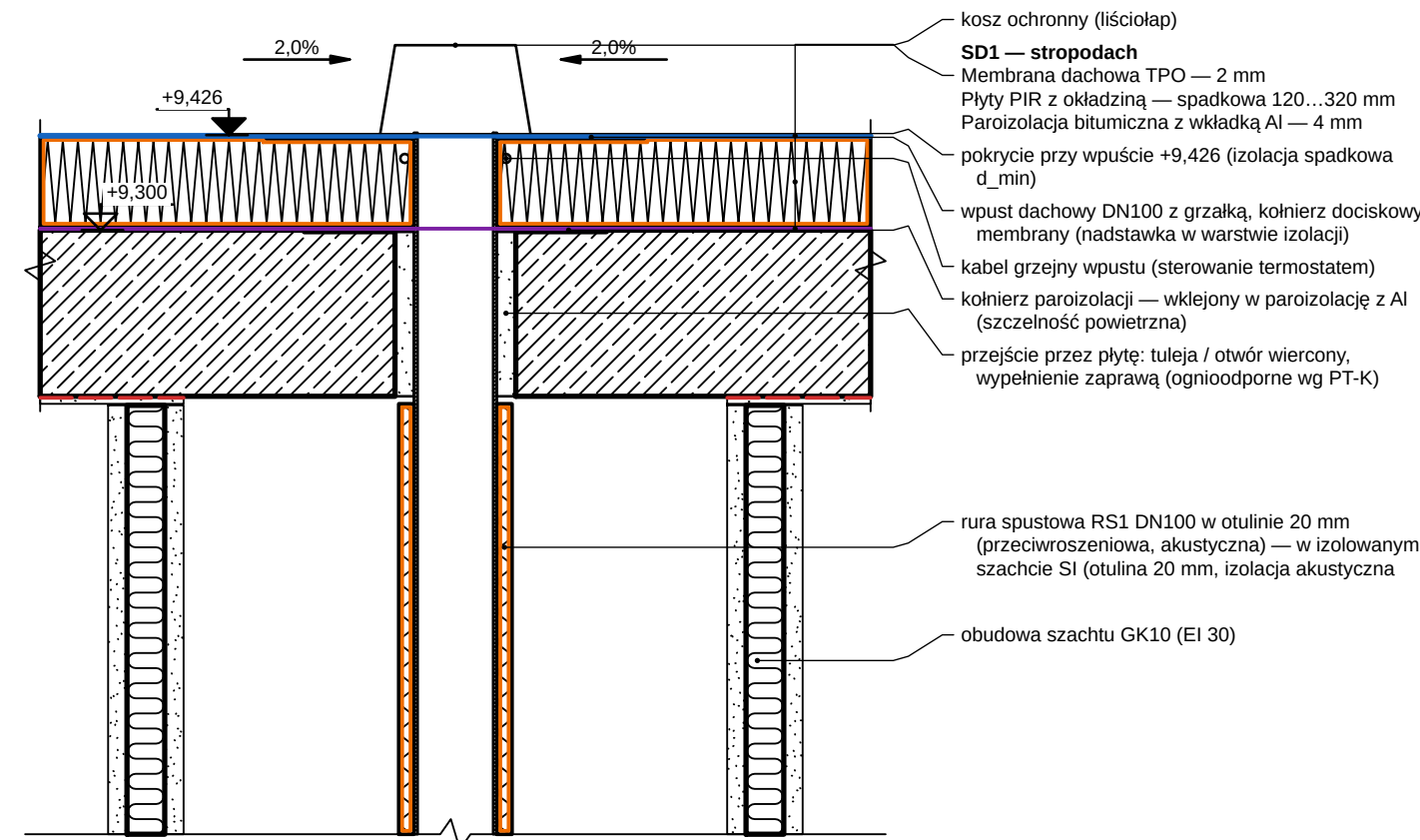
DETAL D-06 — WPUST DACHOWY WP1 I RURA RS1 1:10
