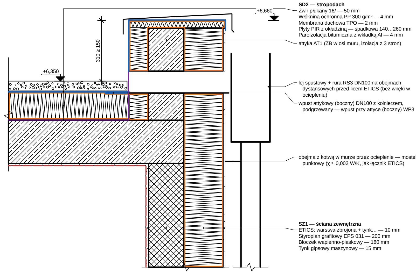
DETAL D-05 — ATTYKA DACHU D2 — WPUST BOCZNY I RURA SPUSTOWA 1:10
