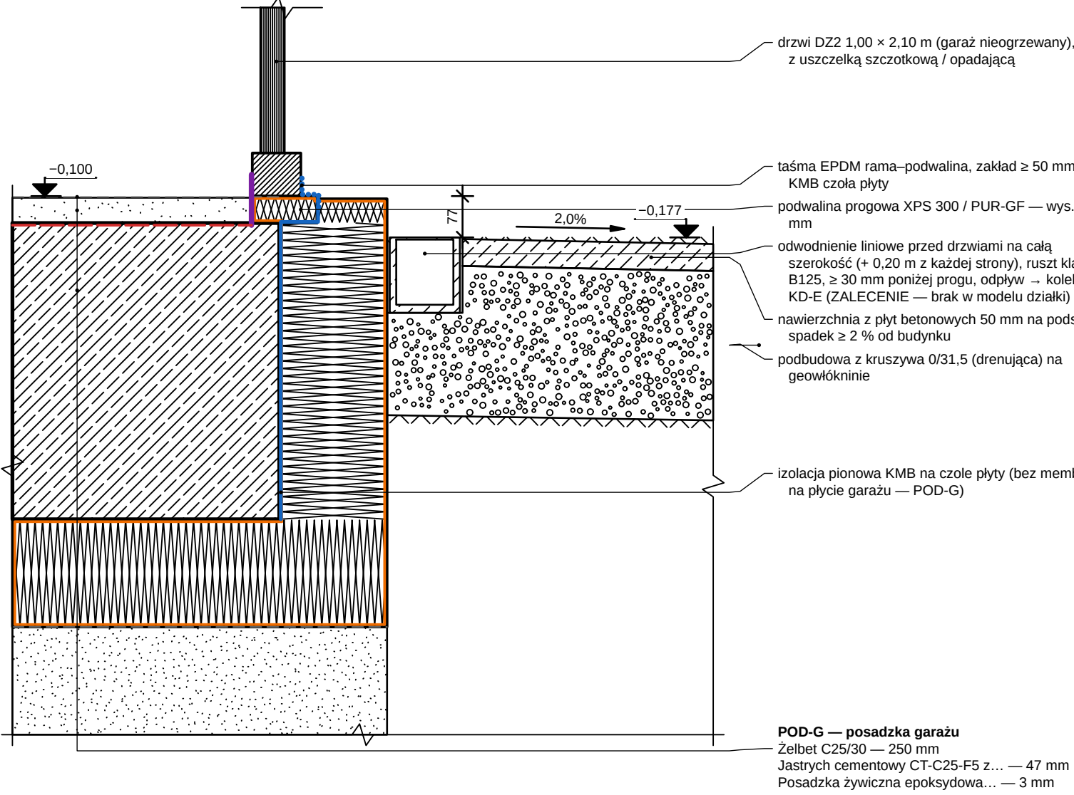
WZ-09b: \psi_e = 0,070 , \psi_{oi} = 0,081 W/(m·K); f_{Rsi} = 0,885 \pm 0,72 — ZLY 4 linie: H OK, S OK, P OK, I uwagi I: WZ-09b: przetrwana: TYNK_GIPS — SIL18 — ZB_C25 — TYNK_CW (płyta ciągła do strefy nieogrzewanej) — mostek konstrukcyjny; obrys izolacji: 3 części (w tym warstwy...)
