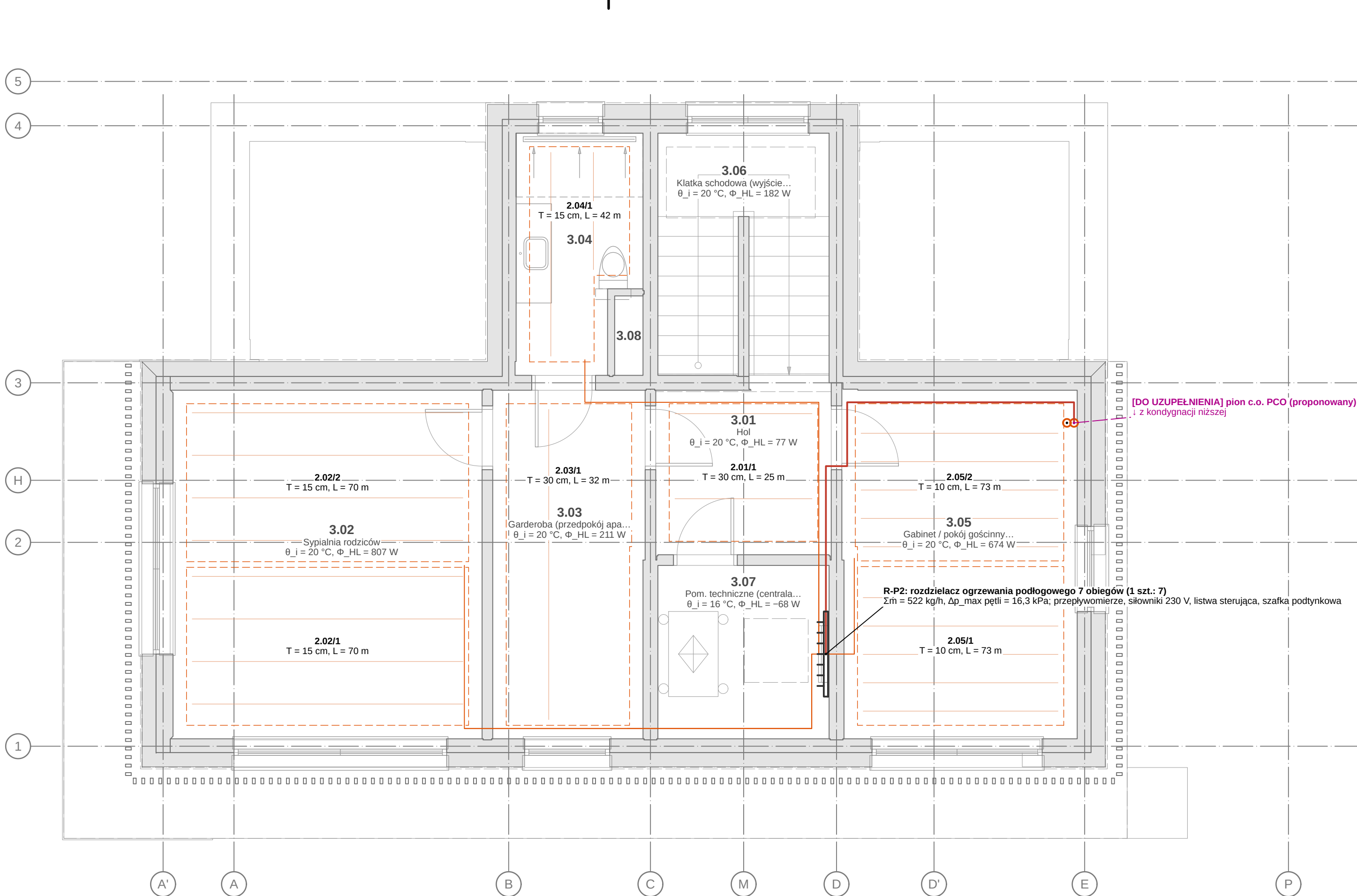
OGRZEWANIE — RZUT II PIĘTRA 1:50
